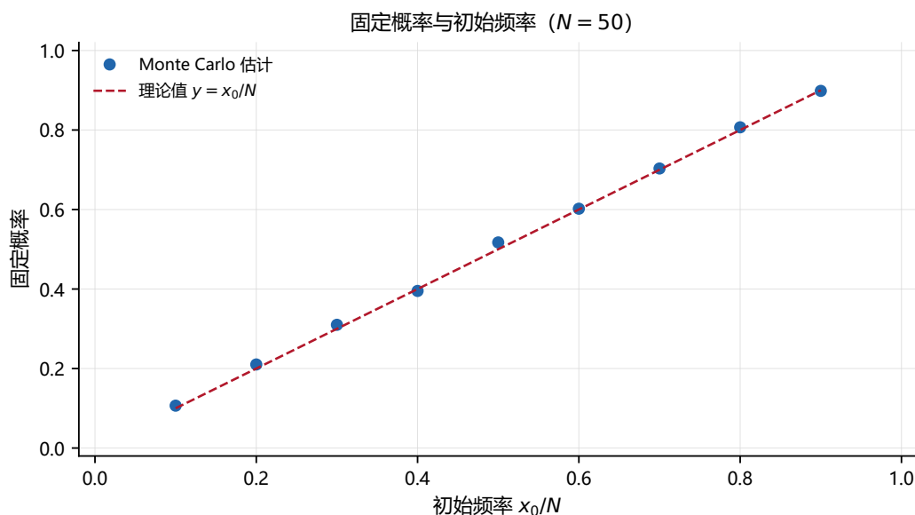
图 2.2 固定概率与初始频率的关系 ( N = 50 )。蓝色圆点为 Monte Carlo 估计 (5000 条路径)；红色虚线为理论值 y = x_0/N ，是 OST 的直接推论。估计值与理论线高度吻合。
