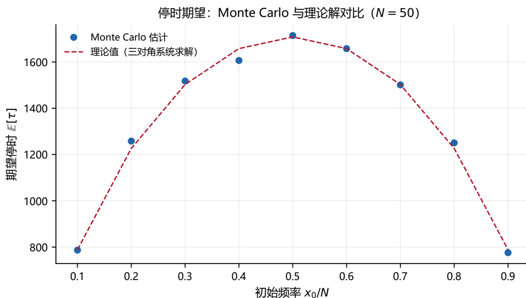
图 2.3 不同初始频率下 Monte Carlo 停时均值与理论解的对比 ( N = 50 )。蓝色圆点为 Monte Carlo 估计 (10000 条路径)；红色虚线为三对角线性系统 (2.16) 给出的理论值。
