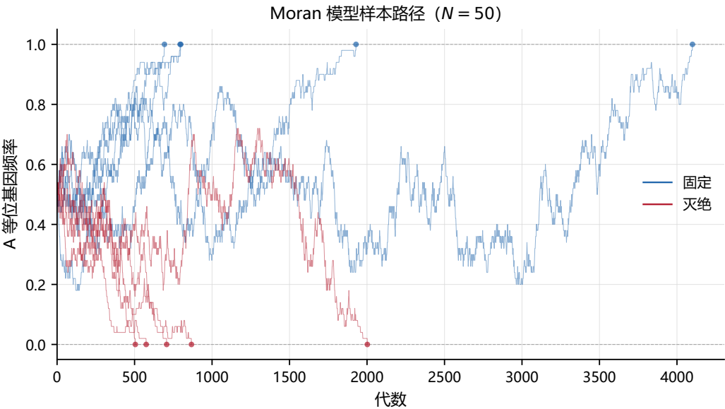
图 2.1 Moran 模型基因频率轨迹 ( N = 50 ，初始频率 0.5)。蓝色路径表示最终固定 (A 取代 a)，红色路径表示最终灭绝 (a 取代 A)。每条轨迹为锯齿状随机游走，最终被 0 或 1 吸收。圆点标记停时位置。
