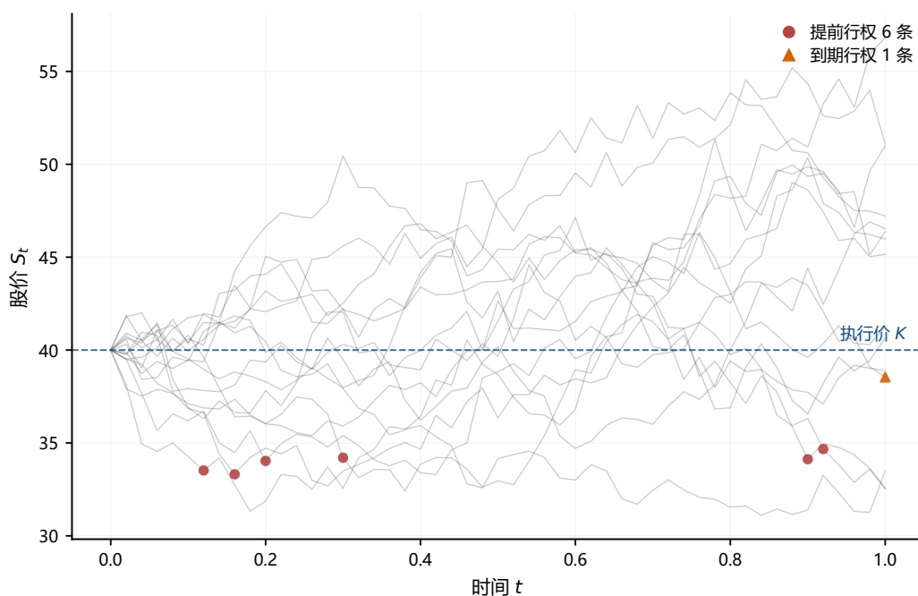
图 6.1 几何布朗运动股价路径与 LSM 判定行权时刻 ( S_0 = 40, K = 40 )。红色圆点标记提前行权，橙色三角标记到期行权；到期价外且 payoff 为 0 的路径不额外标记。水平虚线为执行价 K 。
