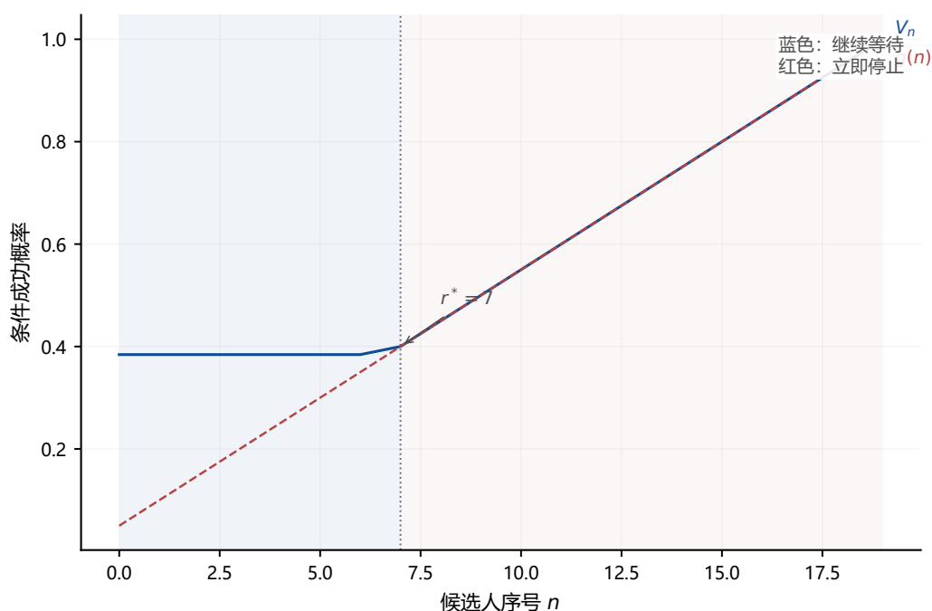
图 5.2 Snell 包络条件值 V_n 与即时 payoff g(n) 的对比 ( N = 20 )。阈值前继续等待价值高于即时收益；阈值 r^* = 7 之后两者重合，表示一旦遇到 record（历史最优）就应立即停止。 7/20 = 0.35 \approx 1/e 。
