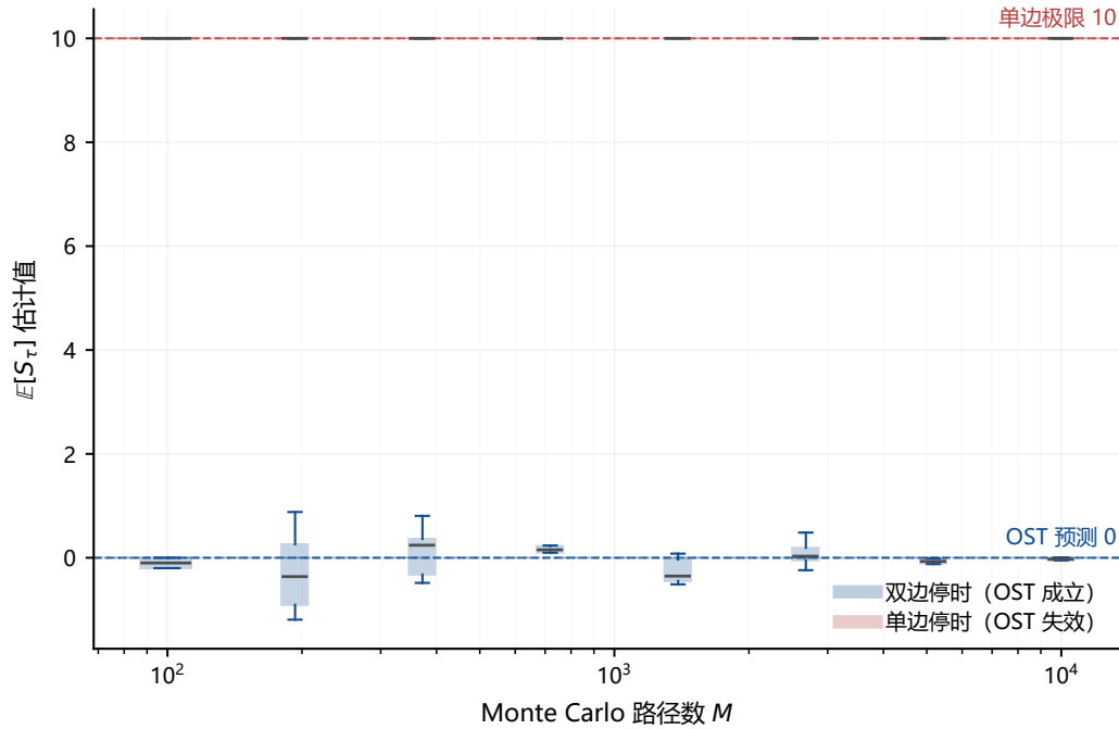
图 4.1 双边停时与单边自然停时的 \mathbb{E}[S_\tau] Monte Carlo 估计对比。双边（蓝色）快速收敛至 OST 预测值 0（虚线）；单边（红色）命中 +b 后恒有 S_\tau = b = 10 ，因此不可能收敛到 0。
