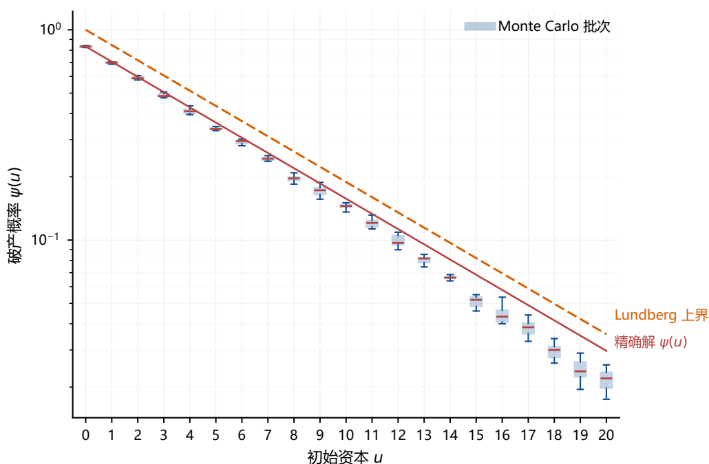
图 3.2 破产概率的半对数图。蓝色箱线图为有限时窗破产概率 P(\tau \leq 100) 的 8 个 Monte Carlo 批次分布（总路径数 16000）；红色实线为指数索赔下最终破产概率的精确解（式 (3.11)）。Lundberg 上界（橙色虚线）始终位于精确解之上，且在半对数图中与精确解保持近似恒定的垂直距离，反映了因子 1/(1 + \theta) 。
