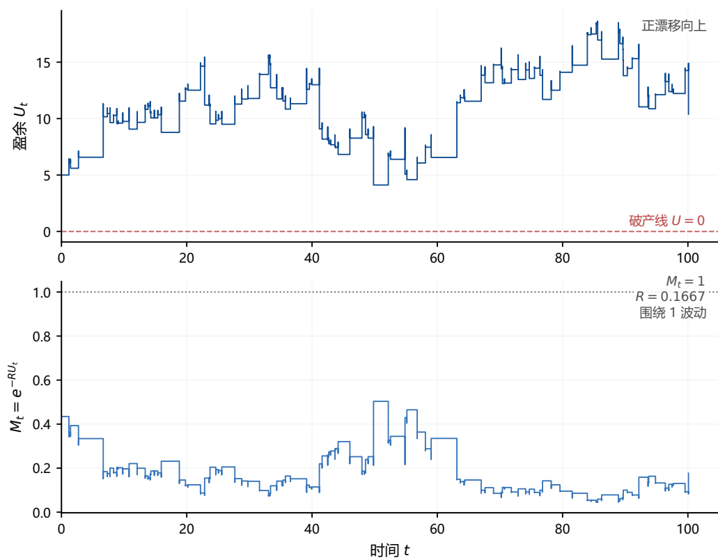
图 3.3 同一路径的盈余过程与对应指数鞅 ( R = 0.1667 )。上子图：盈余 U_t 随时间平均上升（正向漂移 c - \lambda\mu = 0.2 ）。下子图：指数鞅 M_t = e^{-RU_t} ，无趋势，围绕初始值波动——展示了指数变换如何将一个带有漂移的过程转化为鞅。
