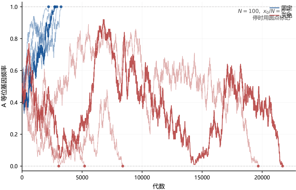
图 2.1 Moran 模型基因频率轨迹（ N = 100 ，初始频率 0.5）。蓝色路径表示最终固定（A 取代 a），红色路径表示最终灭绝（a 取代 A）。每条轨迹为锯齿状随机游走，最终被 0 或 1 吸收。圆点标记停时位置。
