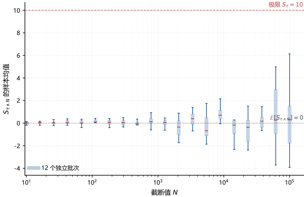
图 4.2 截断序列与不可交换极限。每个箱线图对应固定 N 下 12 次独立 Monte Carlo 估计的样本均值分布。对每个固定 N ，OST 给出 \mathbb{E}[S_{\tau \wedge N}] = 0 （灰色线）；但随机变量本身几乎处处收敛到 S_\tau = b = 10 （红色虚线）。样本均值在大 N 下方差显著增大，说明一致可积性缺失时不能将极限与期望交换。
