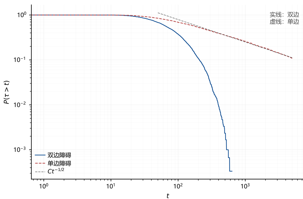
图 4.3 停时生存函数 \mathbb{P}(\tau > t) 的双对数图。双边停时为轻尾, \mathbb{E}[\tau] < \infty ; 单边停时呈 Ct^{-1/2} 型重尾, \mathbb{E}[\tau] = \infty 。重尾性是 OST 条件 3 失效的微观原因。
