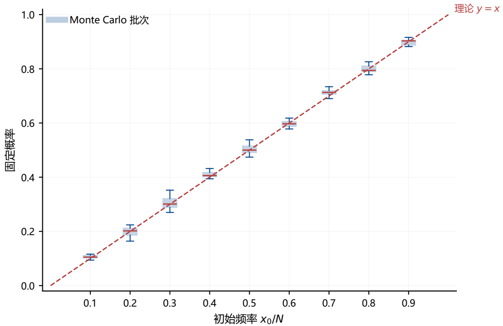
图 2.2 固定概率与初始频率的关系 ( N = 100 )。每个初始频率用 5000 条路径分成 10 个独立批次，箱线图展示批次固定概率分布；红色虚线为理论值 y = x_0/N ，是 OST 的直接推论。批次中位数与理论线高度吻合。
