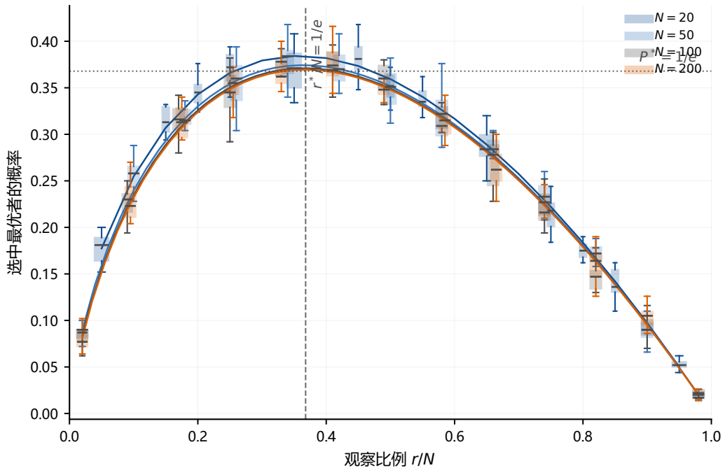
图 5.1 秘书问题成功率与观察比例 r/N 的关系。每个箱线图对应固定 (N, r) 下 10 个独立 Monte Carlo 批次的成功率分布（每点总试验数 5000）；实线为对应的理论曲线。灰色竖虚线标记最优观察比例 r^*/N = 1/e ，灰色水平虚线标记最优成功率极限 1/e 。
