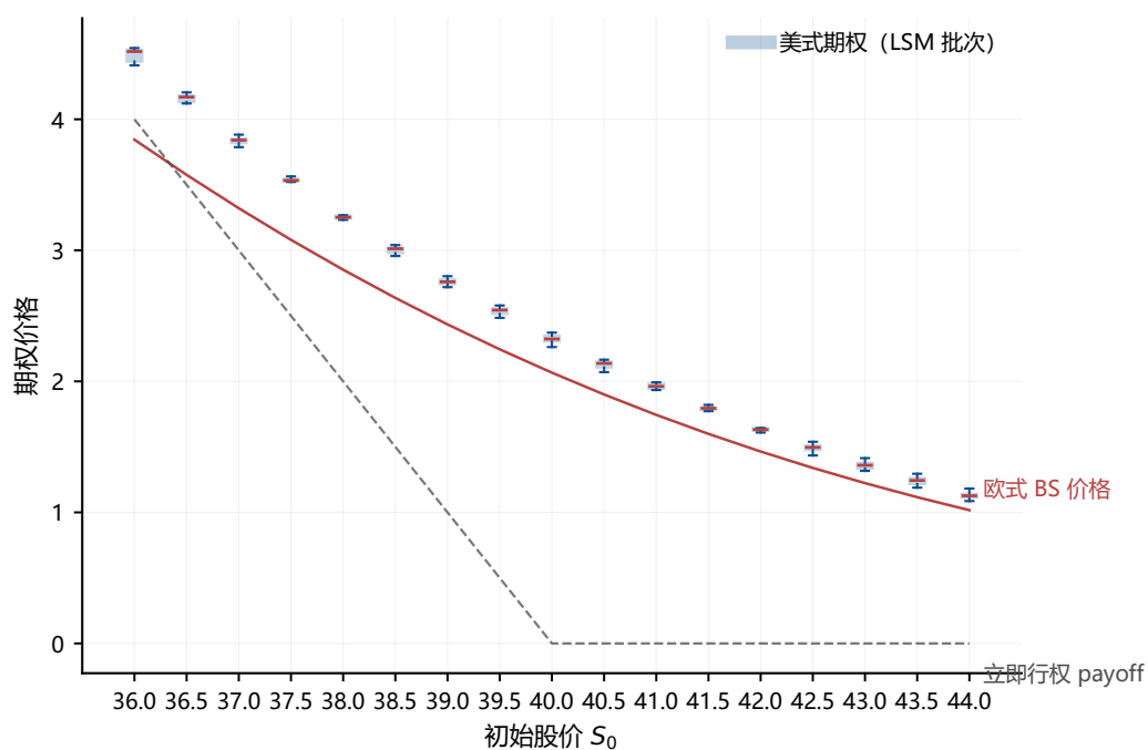
图 6.3 美式 (LSM) 与欧式 (Black-Scholes) 看跌期权价格对比。蓝色箱线图为每个 S_0 下 8 个独立 LSM Monte Carlo 批次的价格分布 (总路径数 30000, N = 50 ); 红色实线为欧式 BS 公式。灰色虚线为立即行权 payoff。美式期权在所有 S_0 处均高于欧式期权, 差额即为提前行权溢价。
