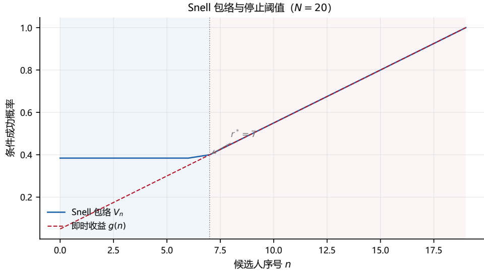
Figure 11: Snell 包络条件值 V_n 与即时 payoff g(n) 的对比 ( N = 20 )。阈值前继续等待价值高于即时收益；阈值 r^* = 7 之后两者重合，表示一旦遇到 record（历史最优）就应立即停止。 7/20 = 0.35 \approx 1/e 。
