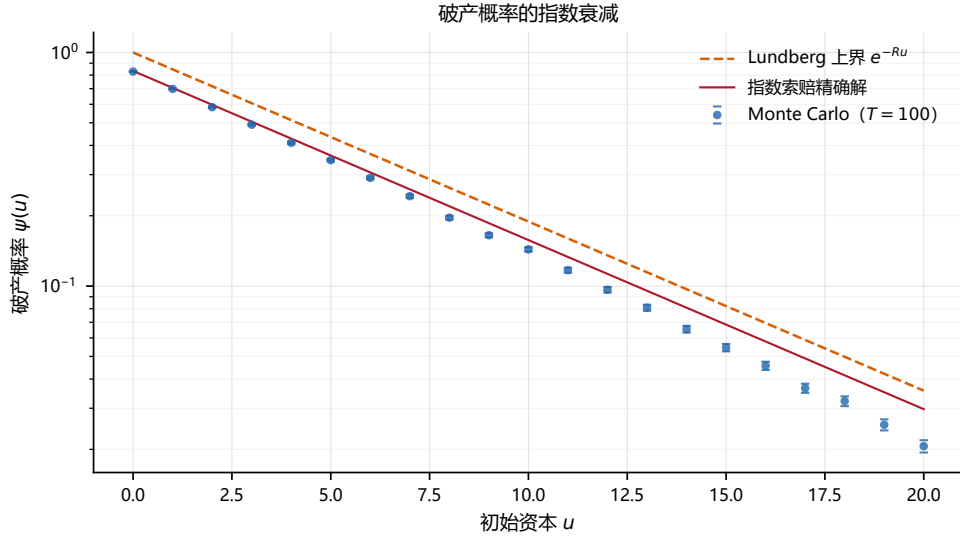
Figure 5: 破产概率的半对数图。Monte Carlo 估计（蓝色圆点， M = 50000 ， T = 100 ）对应有有限视窗破产概率；红色实线为指数索赔下最终破产概率的精确解（式 (27)）。Lundberg 上界（橙色虚线）始终位于精确解之上，且在半对数图中与精确解保持近似恒定的垂直距离，反映了因子 1/(1 + \theta) 。
