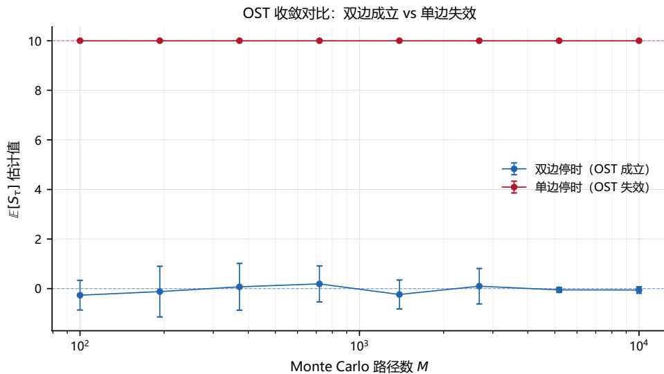
Figure 7: 双边停时与单边自然停时的 \mathbb{E}[S_\tau] Monte Carlo 估计对比。双边 (蓝色) 快速收敛至 OST 预测值 0 (虚线)；单边 (红色) 命中 +b 后恒有 S_\tau = b = 10 ，因此不可能收敛到 0。
