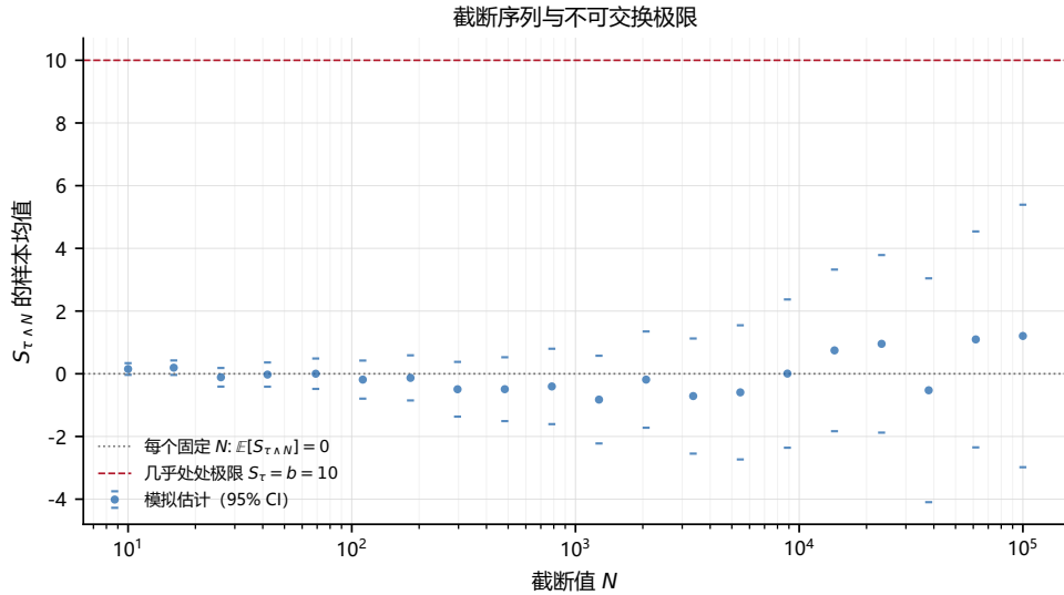
Figure 8: 截断序列与不可交换极限。对每个固定 N ，OST 给出 \mathbb{E}[S_{\tau \wedge N}] = 0 （灰色线）；但随机变量本身几乎处处收敛到 S_\tau = b = 10 （红色虚线）。样本均值在大 N 下方差显著增大，说明一致可积性缺失时不能将极限与期望交换。
