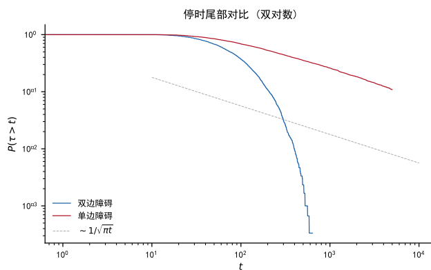
图 9. 停时生存函数 P(\tau > t) 的双对数图。双边停时：指数衰减（轻尾）， E[\tau] < \infty 。单边停时： \sim 1/\sqrt{\pi t} 衰减（重尾）， E[\tau] = \infty 。灰色虚线为参考线 1/\sqrt{\pi t} 。重尾性是 OST 条件 3 失效的微观原因。
