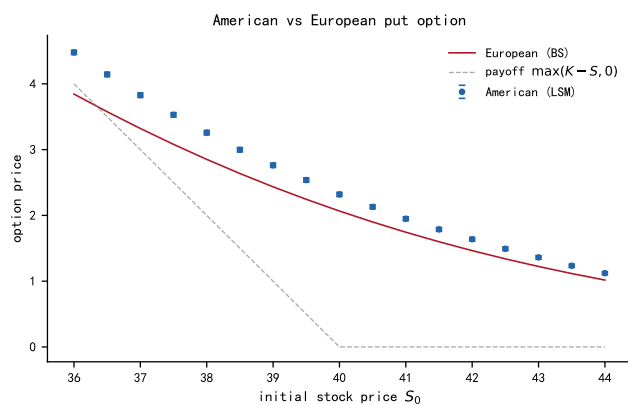
图 15. 美式 (LSM) 与欧式 (Black-Scholes) 看跌期权价格对比。蓝色圆点为 LSM Monte Carlo 估计 ( M = 30000 , N = 50 ), 误差棒极小 (95% CI)。红色实线为欧式 BS 公式。灰色虚线为立即行权 payoff。美式期权在所有 S_0 处均高于欧式期权, 差额即为提前行权溢价。
