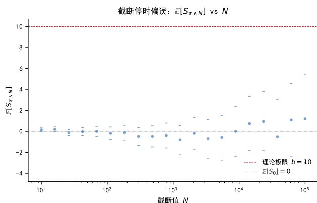
图 8. 截断停时偏差: E[S_{\tau \wedge N}] 随截断值 N 的变化。尽管 OST 对任意固定 N 成立 ( E[S_{\tau \wedge N}] = 0 )，但 E[S_{\tau \wedge N}] 随 N \rightarrow \infty 的收敛极慢，即便 N = 10^5 时仍显著偏离 0。两条参考线标明了 OST 预测值 (0) 和极限值 ( b = 10 )。
