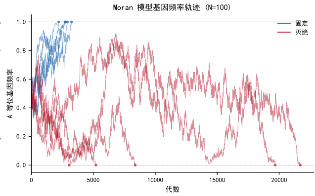
图 1. Moran 模型基因频率轨迹 ( N = 100 ，初始频率 0.5)。蓝色路径表示最终固定（A 取代 a），红色路径表示最终灭绝（a 取代 A）。每条轨迹为锯齿状随机游走，最终被 0 或 1 吸收。圆点标记停时位置。
