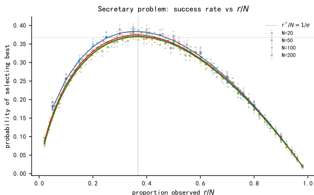
图 10. 秘书问题成功率与观察比例 r/N 的关系。散点为 Monte Carlo 估计（每种 N 各 5000 次试验）。实线为 N \rightarrow \infty 时的理论曲线。灰色竖虚线标记最优观察比例 r^*/N = 1/e ，灰色水平虚线标记最优成功率极限 1/e 。
