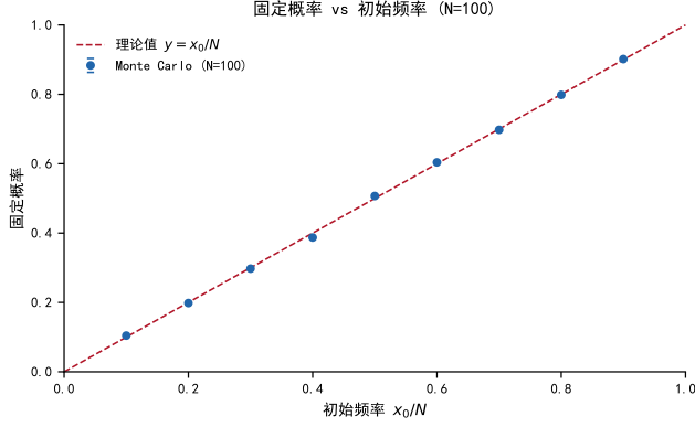
图 2. 固定概率与初始频率的关系 ( N = 100 )。散点为 Monte Carlo 估计 (5000 条路径 \times 9 个初始频率)，误差棒为 95% 置信区间。红色虚线为理论值 y = x_0/N ，是 OST 的直接推论。模拟与理论高度吻合，所有误差棒均跨越对角线。
