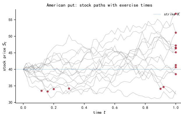
图 13. 几何布朗运动股价路径与 LSM 判定行权时刻（ S_0 = 40, K = 40 ）。红色圆点标记 LSM 算法判定的最优行权位置。多数行权发生在股价低于执行价（in-the-money）且离到期日尚有一段时间时。水平虚线标记执行价 K 。
