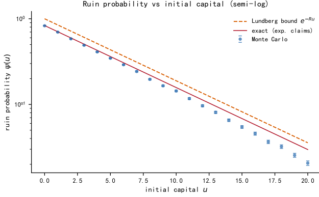
图 5. 破产概率的半对数图。Monte Carlo 估计（蓝色圆点， M = 50000 ）与指数索赔精确解（红色实线，式 (27)）在 u \leq 10 区域高度吻合。Lundberg 上界（橙色虚线）始终位于两者之上，且在半对数图中与精确解保持近似恒定的垂直距离，反映了因子 1/(1 + \theta) 。
