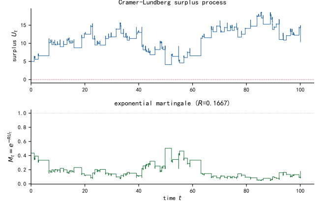
图 6. 同一路径的盈余过程与对应指数鞅（ R = 0.1667 ）。上子图：盈余 U_t 随时间平均上升（正向漂移 c - \lambda\mu = 0.2 ）。下子图：指数鞅 M_t = e^{-RU_t} ，无趋势，围绕初始值波动——展示了指数变换如何将一个带有漂移的过程转化为鞅。
