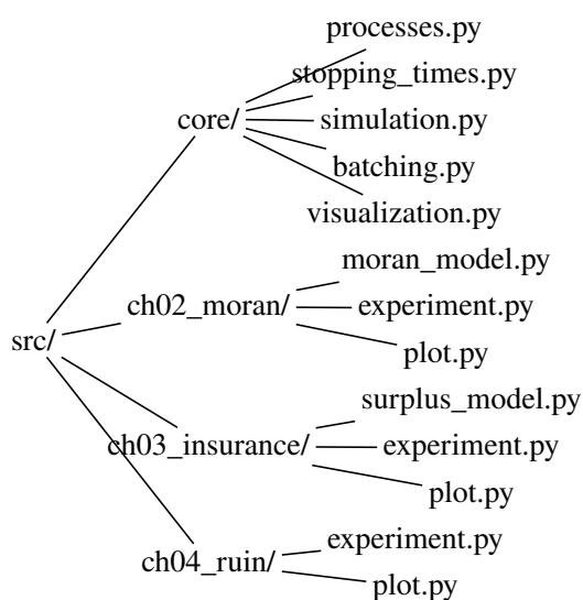
图 1.1 项目代码文件架构。核心层 ( src/core/ ) 提供可复用的鞅过程、停时和模拟引擎；实验层每章包含模型定义、实验脚本和绘图脚本三个模块。
