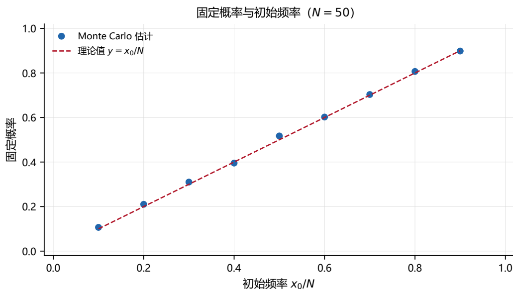
图 2.2 固定概率与初始频率的关系 ( N = 50 )。蓝色圆点为 Monte Carlo 估计 (5000 条路径); 红色虚线为理论值 y = x_0/N , 是 OST 的直接推论。估计值与理论线高度吻合。
