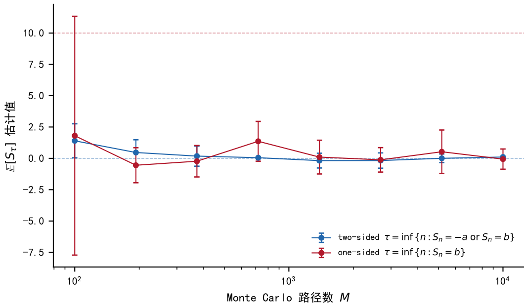
OST 收敛对比：双边成立 vs 单边失效
