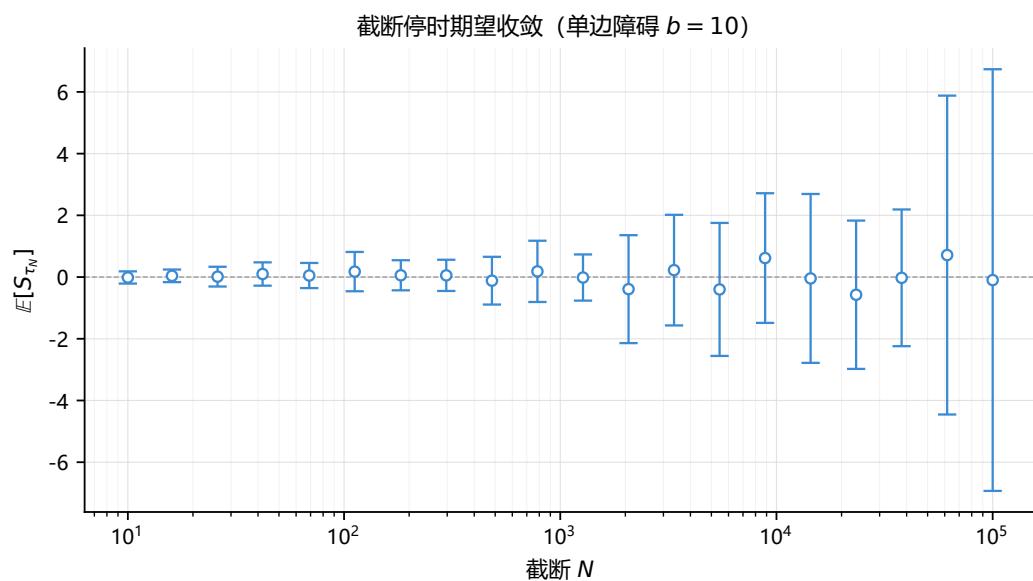
图 4.4 截断停时期望 \mathbb{E}[S_{\tau_N}] 随截断 N 的变化。Monte Carlo 估计 (1000 条路径, 12 批次, 误差棒为 95% 置信区间), 灰色虚线为零线。对所有 N , 估计值均围绕零波动, 不收敛至 b = 10 , 体现了一致可积性的缺失。
