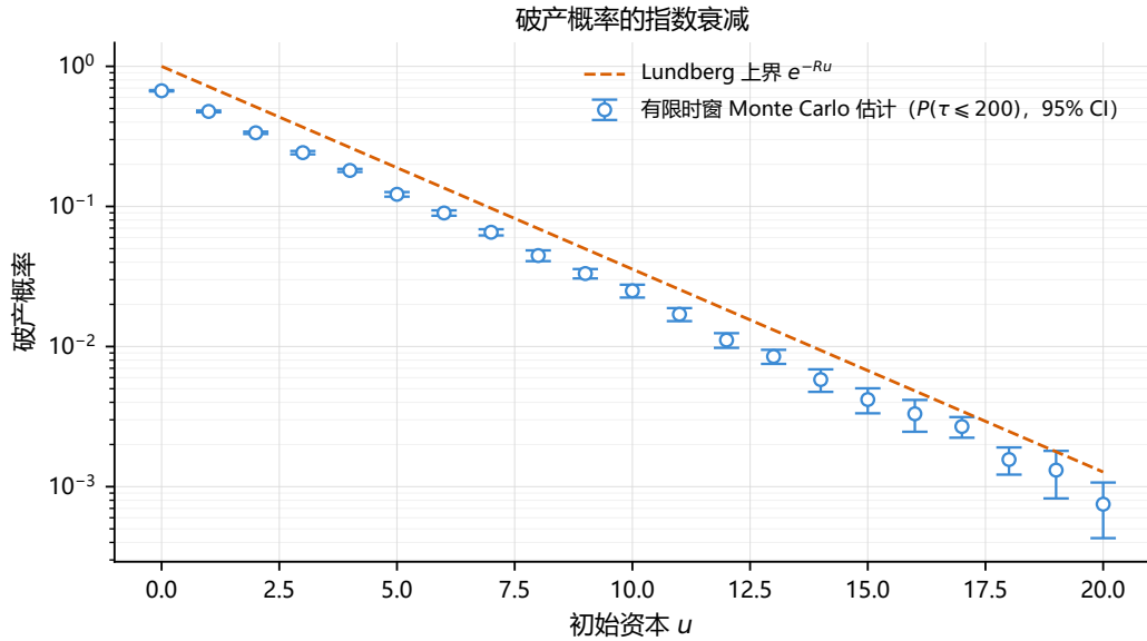
图 3.2 破产概率的半对数图。蓝色圆点为有限时窗破产概率 P(\tau \leq 200) 的 Monte Carlo 估计 (16000 条路径)，误差棒表示 95% 置信区间；橙色虚线为 Lundberg 上界 e^{-Ru} 。上界始终位于模拟结果之上。
