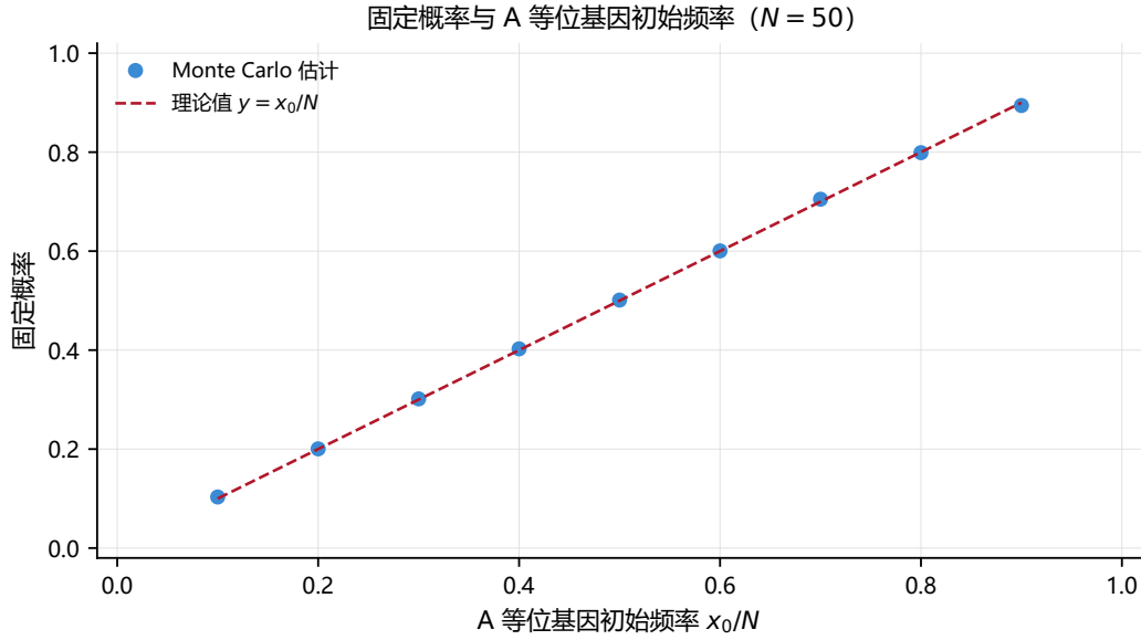
图 2.2 固定概率与 A 等位基因初始频率的关系 ( N = 50 )。蓝色圆点为 Monte Carlo 估计 (20000 条路径)；红色虚线为理论值 y = x_0/N ，是 OST 的直接推论。估计值与理论线高度吻合。
