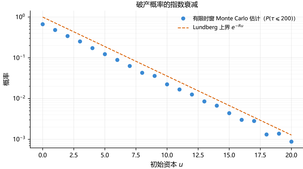
图 3.2 破产概率的半对数图。蓝色圆点为有限时窗破产概率 P(\tau \leq 200) 的 Monte Carlo 估计 (16000 条路径)；橙色虚线为 Lundberg 上界 e^{-Ru} 。上界始终位于模拟结果之上。
