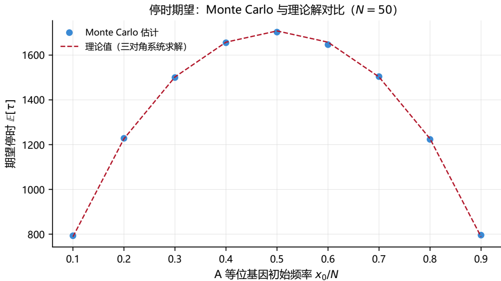
图 2.3 不同 A 等位基因初始频率下 Monte Carlo 停时均值与理论解的对比 ( N = 50 )。蓝色圆点为 Monte Carlo 估计 (20000 条路径)；红色虚线为三对角线性系统 (2.10) 给出的理论值。
