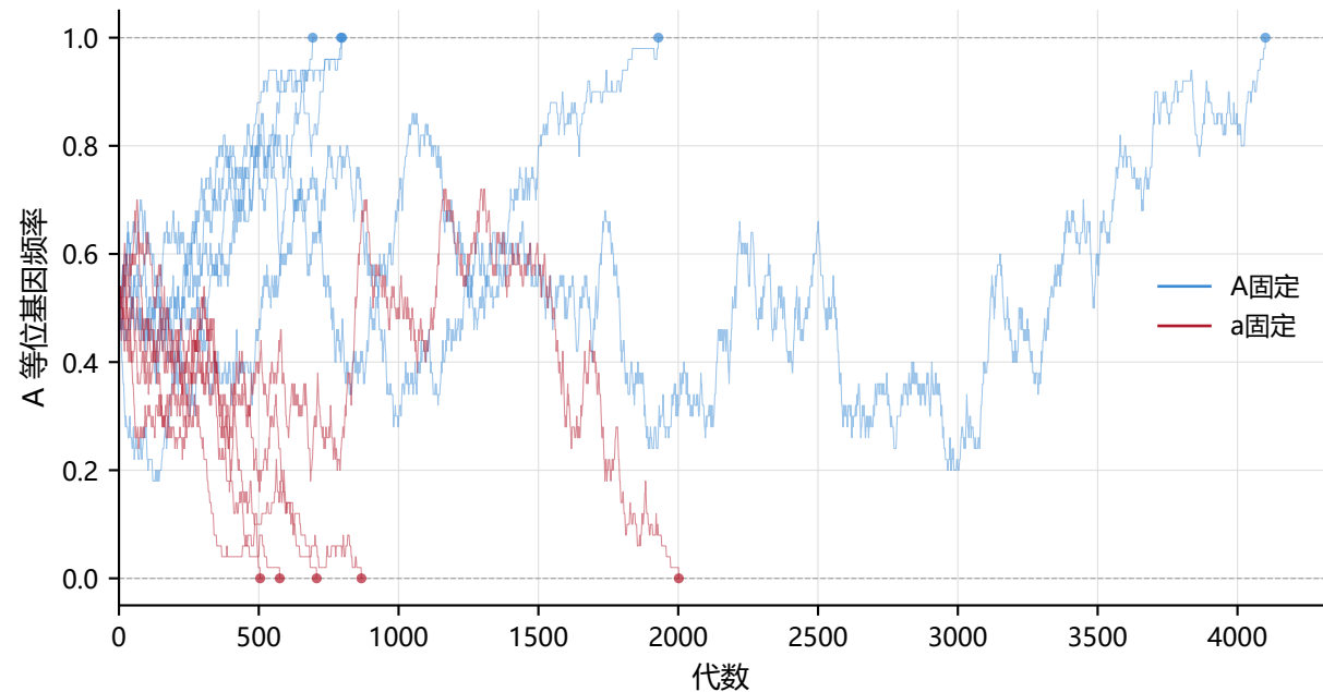
Moran 模型样本路径 ( N = 50 )
