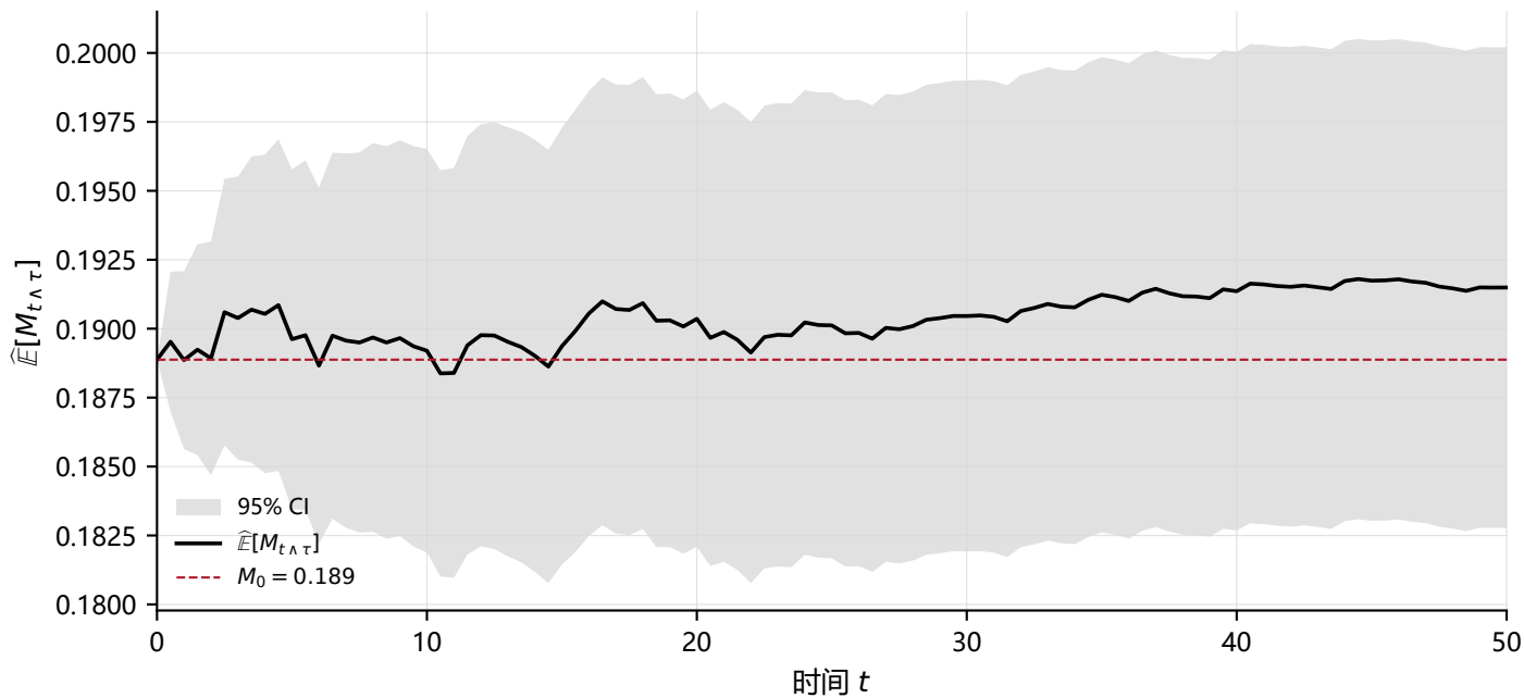
停止指数鞅的均值曲线 ( R = 0.3333 )
