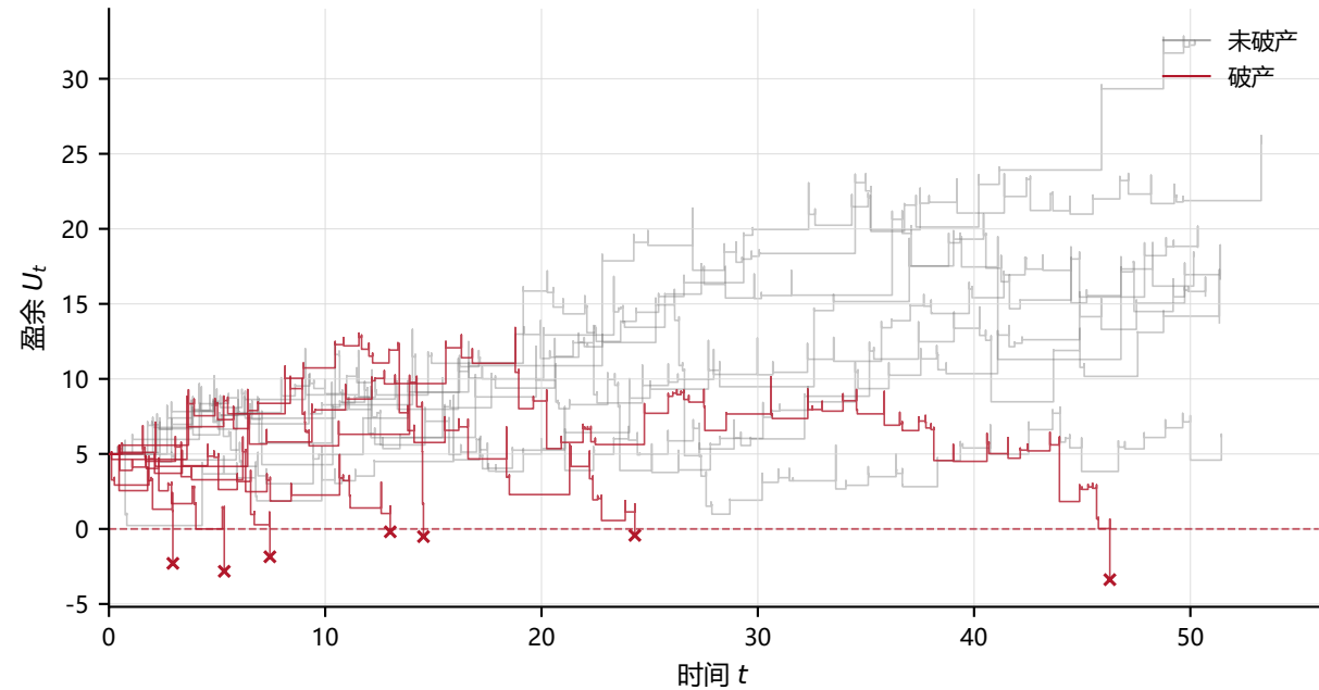
Cramér-Lundberg 盈余路径 (破产 7/15)
