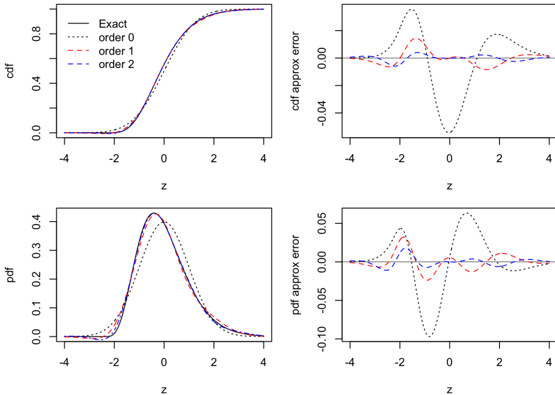
图 2.2: n = 6 时指数分布标准化样本均值的 Edgeworth 近似; 图片来自 https://gregorkb.github.io/nonparam/edgeworthplay.html
