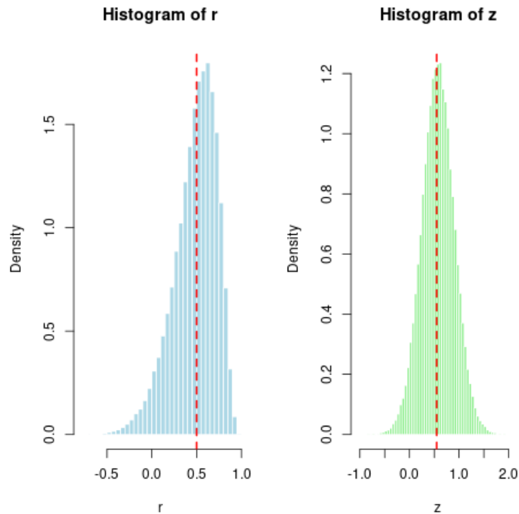
图 5.1: Fisher z -变换前后的模拟分布 (R 绘制)
