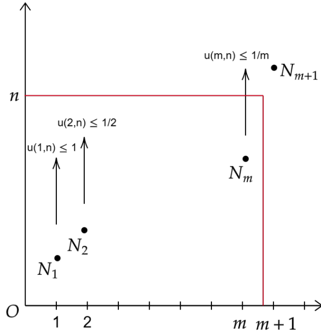
图 3.1: 对角序列 m_n 的构造示意图 (Mathcha 绘制)
