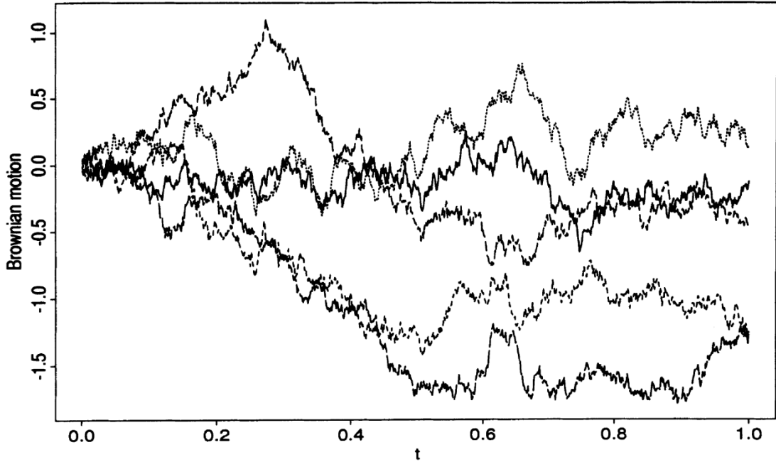
图 4.6: [0, 1] 上标准 Brown 运动的五条样本轨迹。图片来自 [3], p. 89
