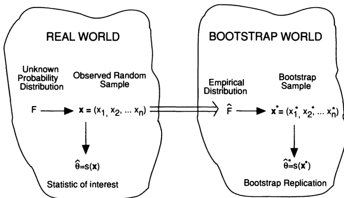
图 11.1: Bootstrap 中总体、经验分布与重抽样经验分布的对应。图片来自 [10], p. 91
