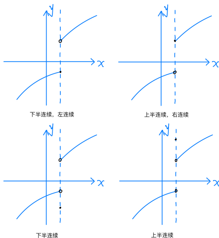
图 9.3: 上半连续与下半连续的示意图。图片来自 https://www.cnblogs.com/BoyaYan/p/17237330.html
