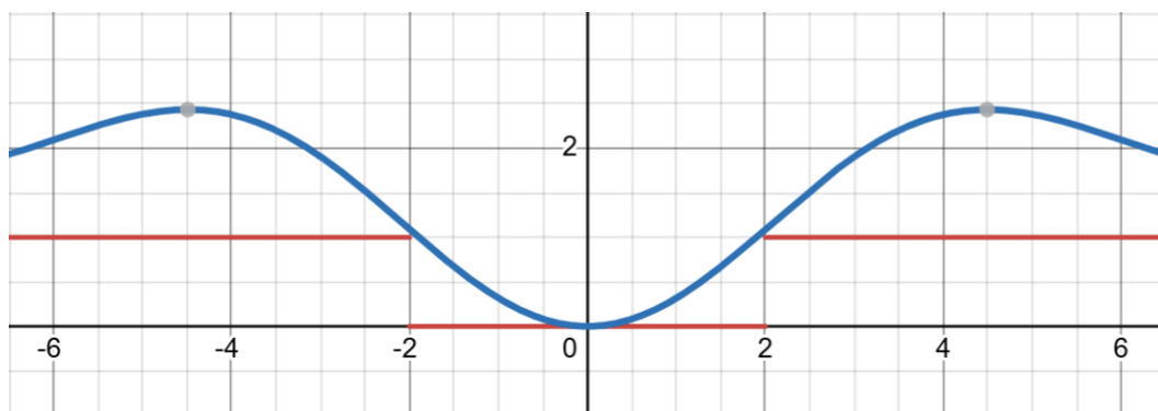
图 2.1: \mathbb{I}(|x| > 2) 与 2(1 - \sin x/x) 的比较 (Desmos 绘制)
