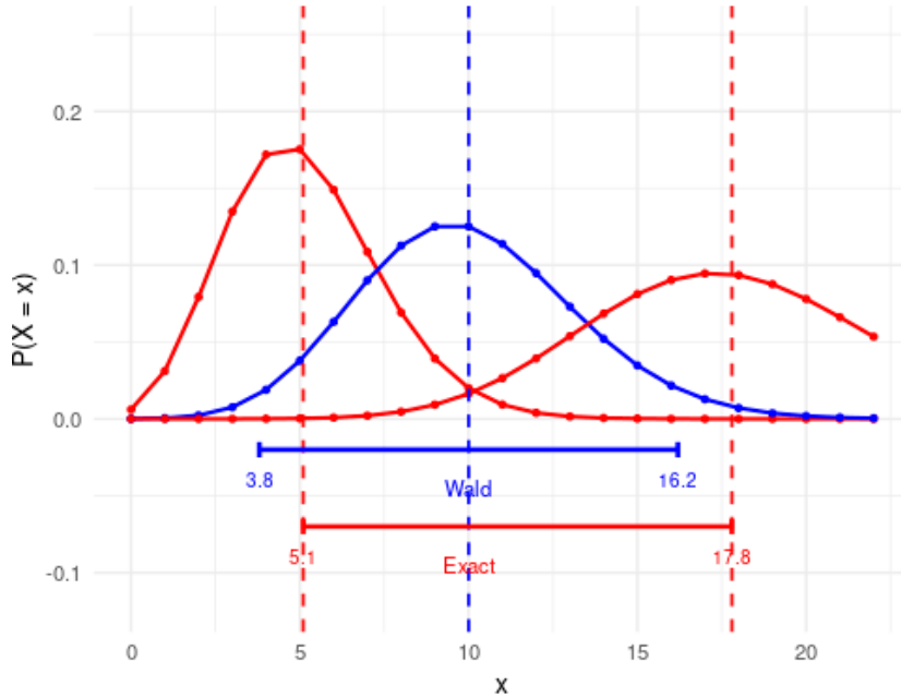
图 11.3: Poisson 均值的 Wald 区间与等尾区间 (R 绘制)
