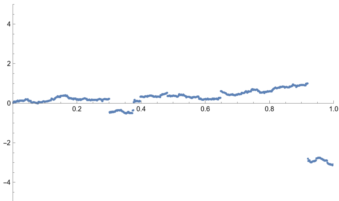
图 4.9: \alpha -稳定过程的模拟路径 (Mathematica 13.3)
