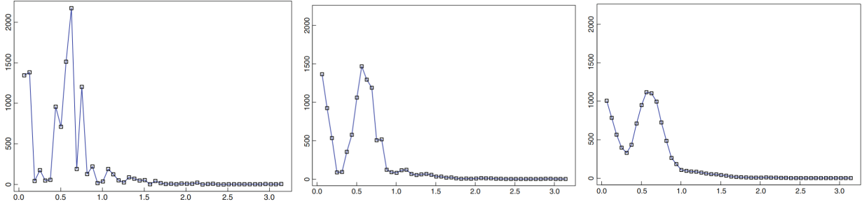
图 4.3: 离散谱平均估计的示意图。图片来自 [5], §4.2
