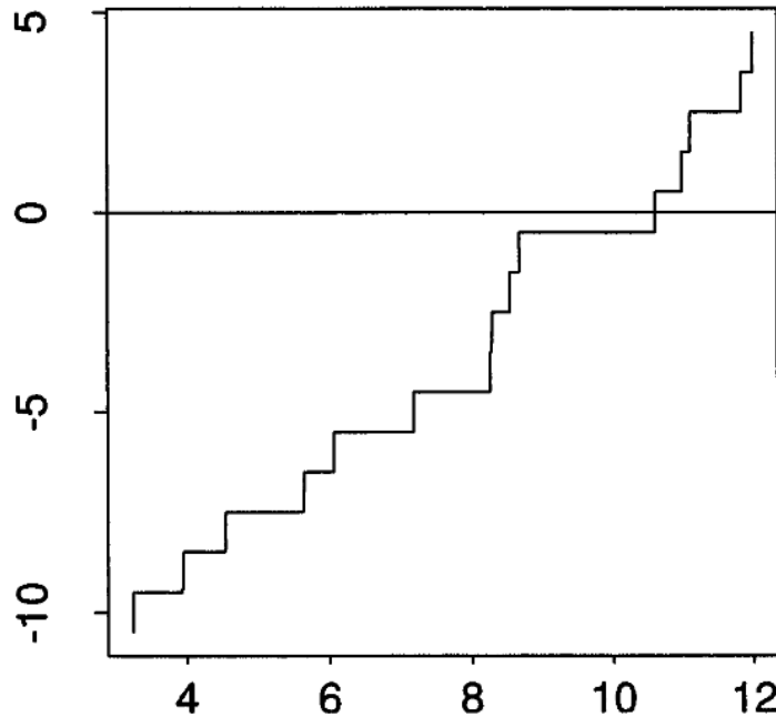
图 9.1: 从 \text{Gamma}(5, 1) 抽取 15 个样本得到的 \Psi_n(\theta) 。图片来自 [8], p. 44
