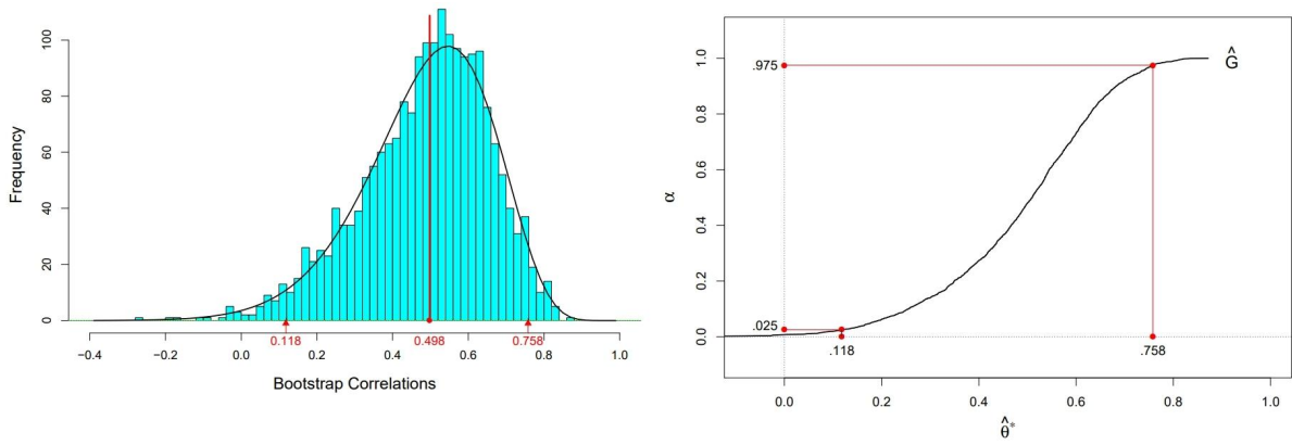
图 11.4: 相关系数的 Bootstrap 分布与百分位区间。图片来自 [9], §11.2
