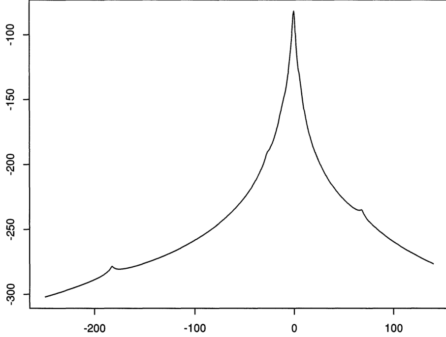
图 7.1: Cauchy 位置模型的对数似然函数。图片来自 [11], p. 74
