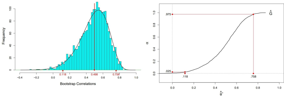
图 11.4: 相关系数的 Bootstrap 分布与百分位区间。图片来自 [10], §11.2
