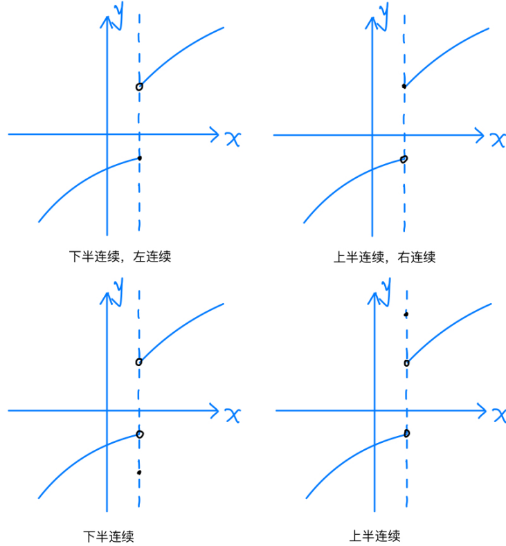
图 9.4: 上半连续与下半连续的示意图。图片来自 https://www.cnblogs.com/BoyaYan/p/17237330.html
