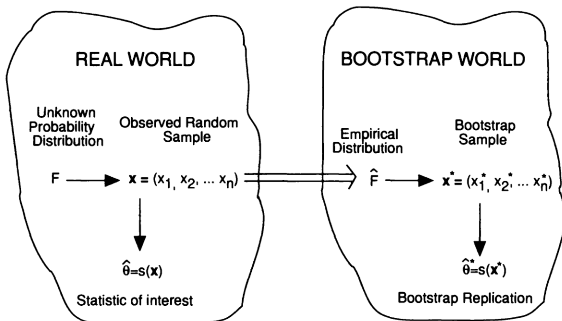
图 11.1: Bootstrap 中总体、经验分布与重抽样经验分布的对应。图片来自 [11], p. 91
