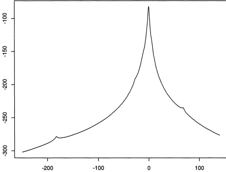
图 7.1: Cauchy 位置模型的对数似然函数。图片来自 [11], p. 74
