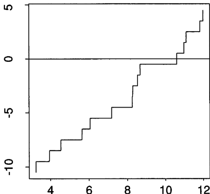
图 9.2: 从 \text{Gamma}(5, 1) 抽取 15 个样本得到的 \Psi_n(\theta) 。图片来自 [9], p. 44
