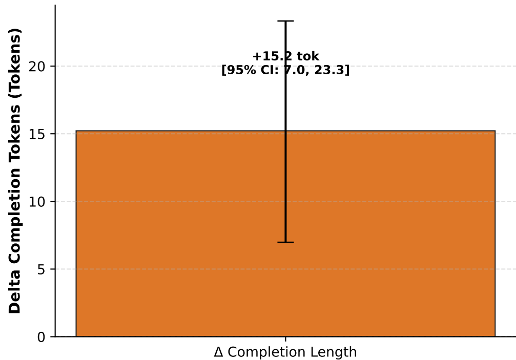
Completion Token Shift ( \Delta Tokens) Permutation p = 0.0003
