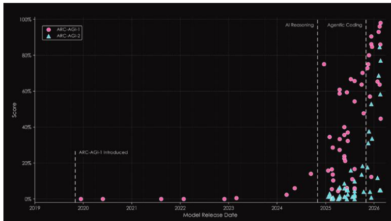
Arc AGI 1 & 2
