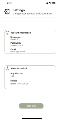
Fig. 18. Settings page
