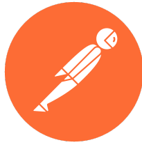
Fig. 10. Postman
