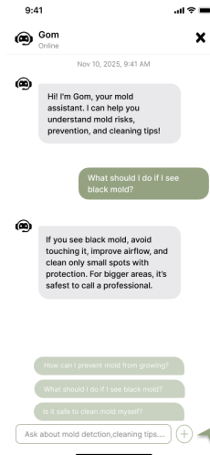
Fig. 17. Chatbot page
