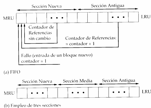
FIGURA 10.9 Reemplazo en función de la frecuencia
