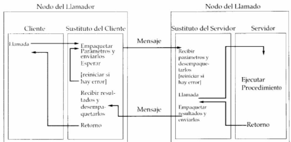
FIGURA 12.25 Lógica de llamada a procedimientos remotos [KRAK88]
