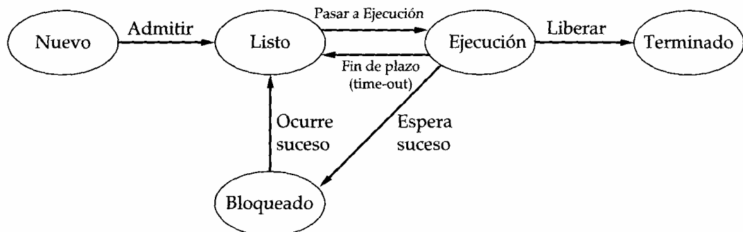
FIGURA 3.5 Modelo de procesos de cinco estados
