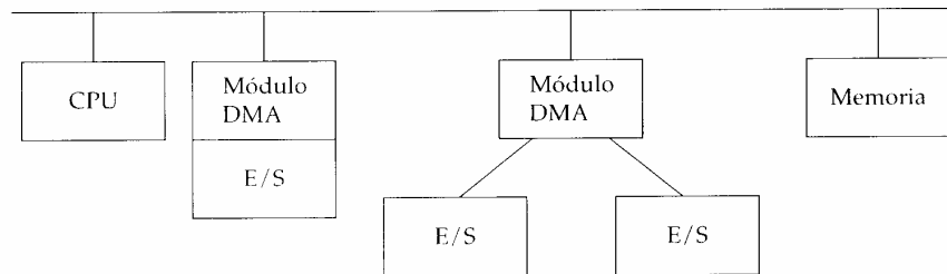
(b) Integración DMA-E/S de bus sencillo
