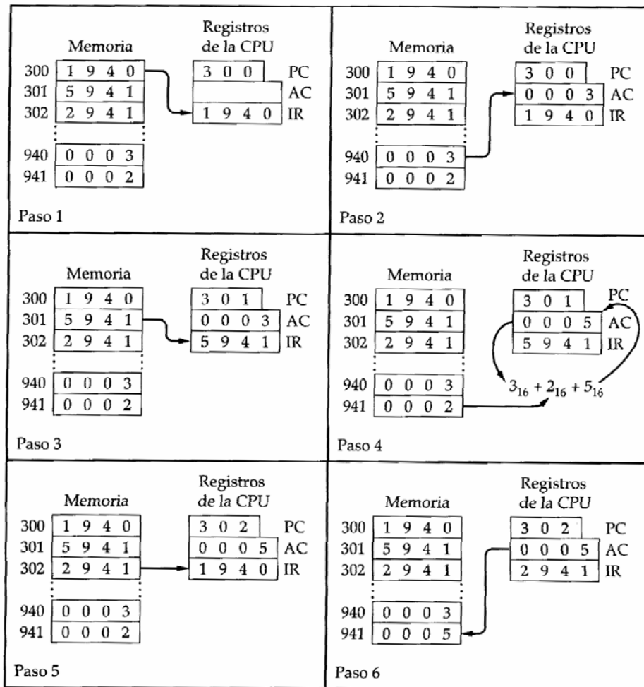
FIGURA 1.4 Ejemplo de ejecución de un programa
