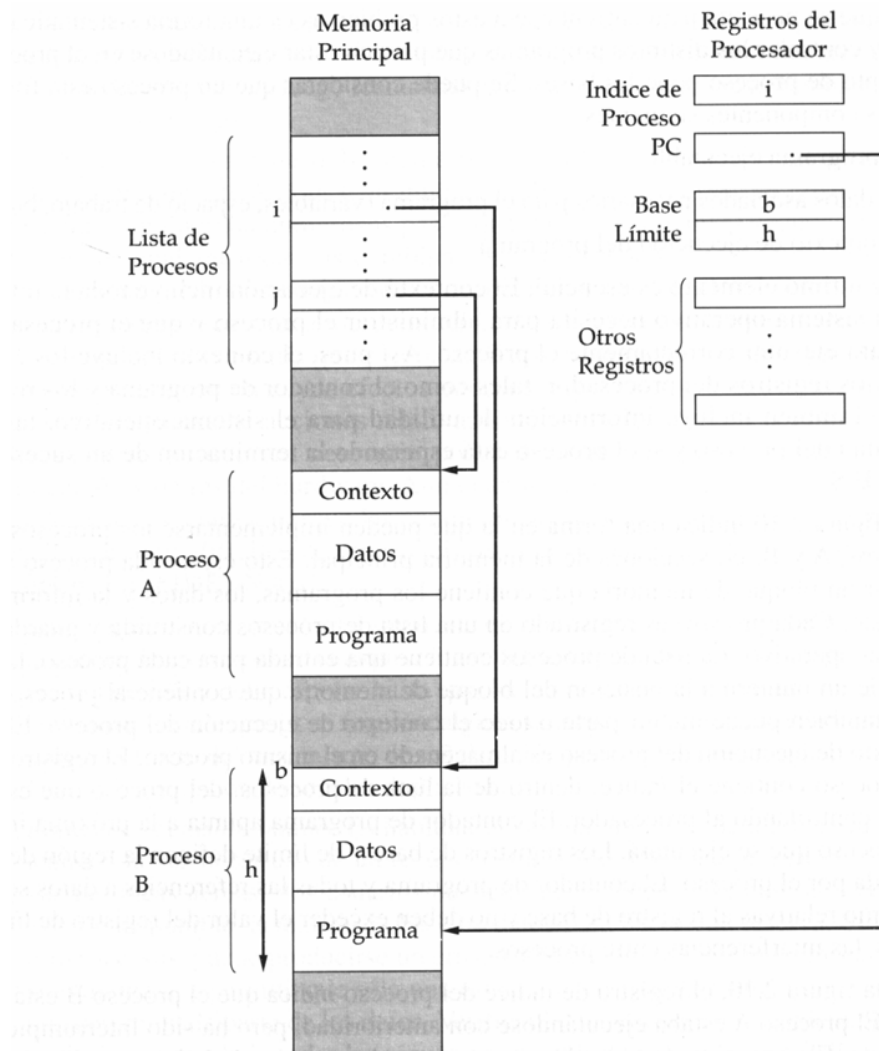
FIGURA 2.10 Implementación típica de los procesos
