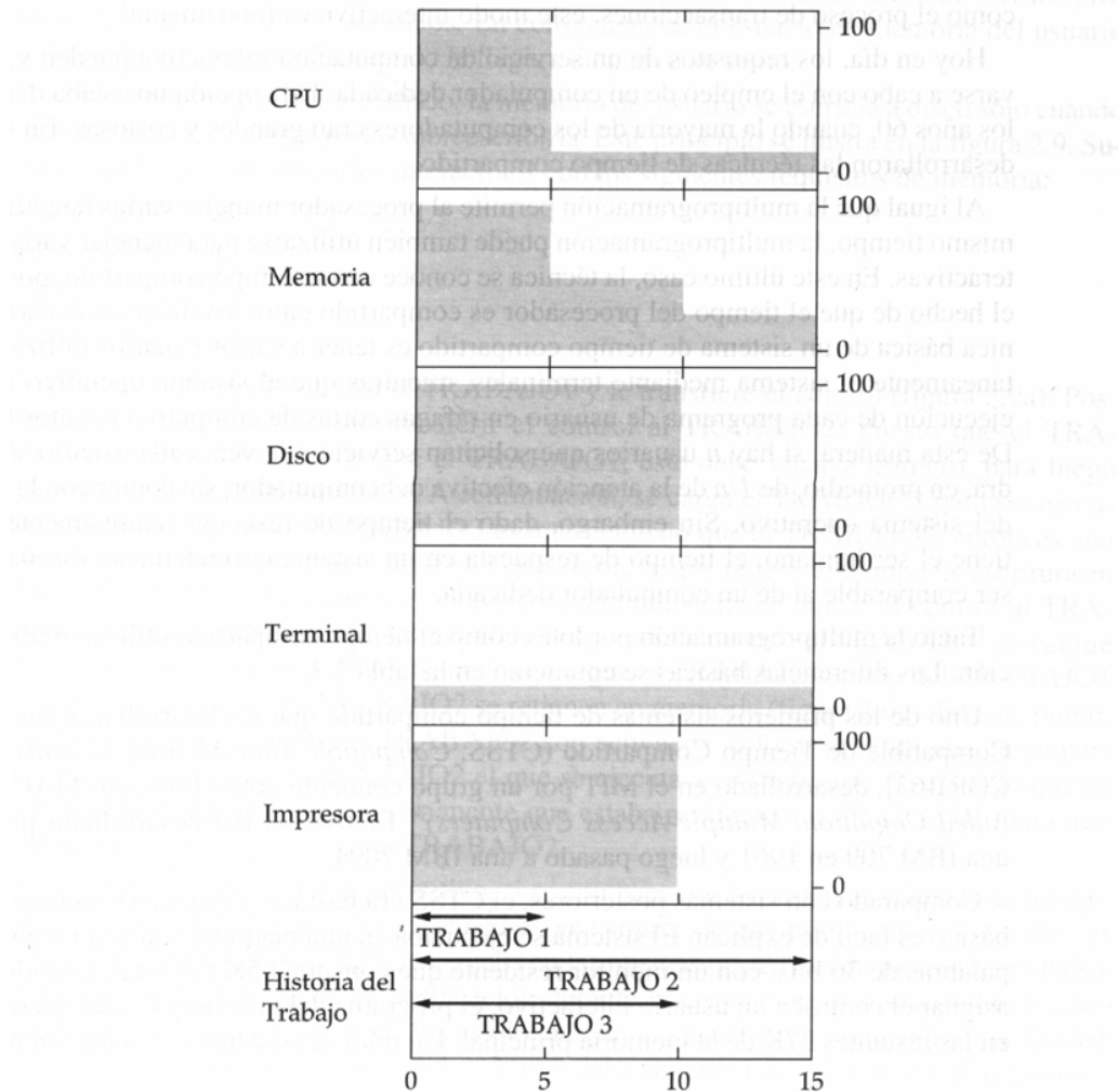
FIGURA 2.8. Histograma de utilización con multiprogramación [TURN86]
