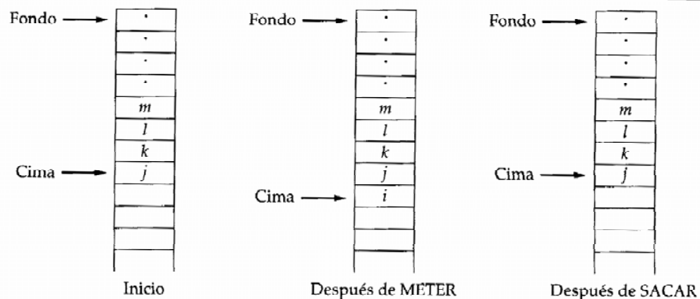
FIGURA 1.26 Operaciones básicas sobre una pila
