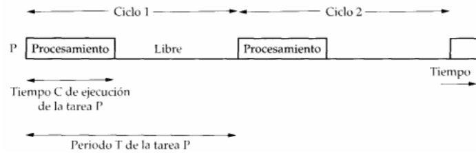
FIGURA 9.7 Diagrama de tiempos de tareas periódicas
