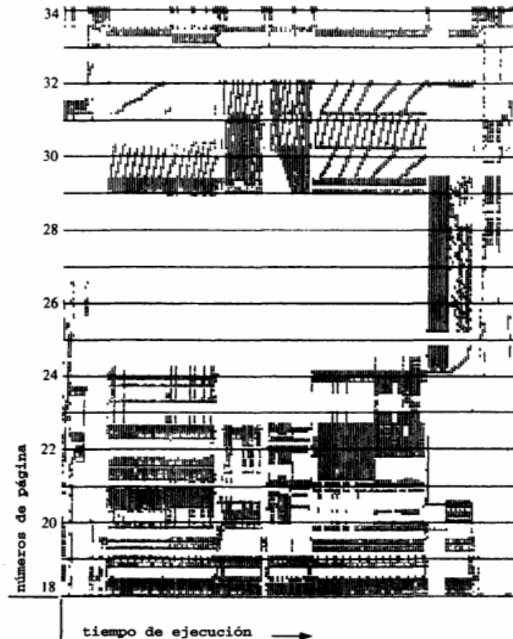
FIGURA 7.1 Comportamiento de la paginación
