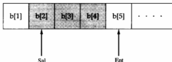
FIGURA 4.13 Buffer ilimitado en el problema del productor/consumidor
