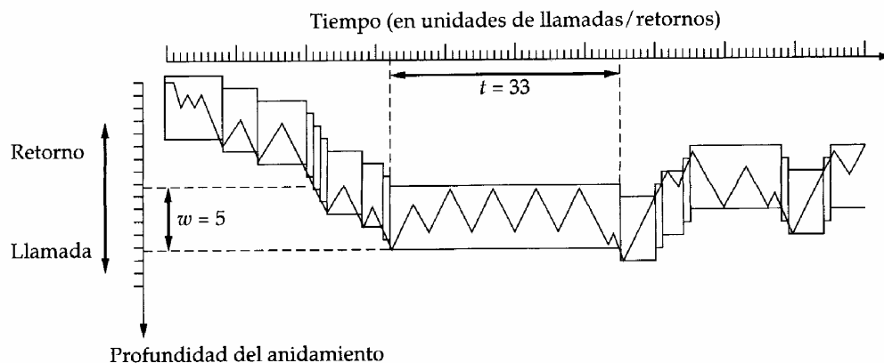
FIGURA 1.22 Comportamiento de llamadas/retornos en los programas
