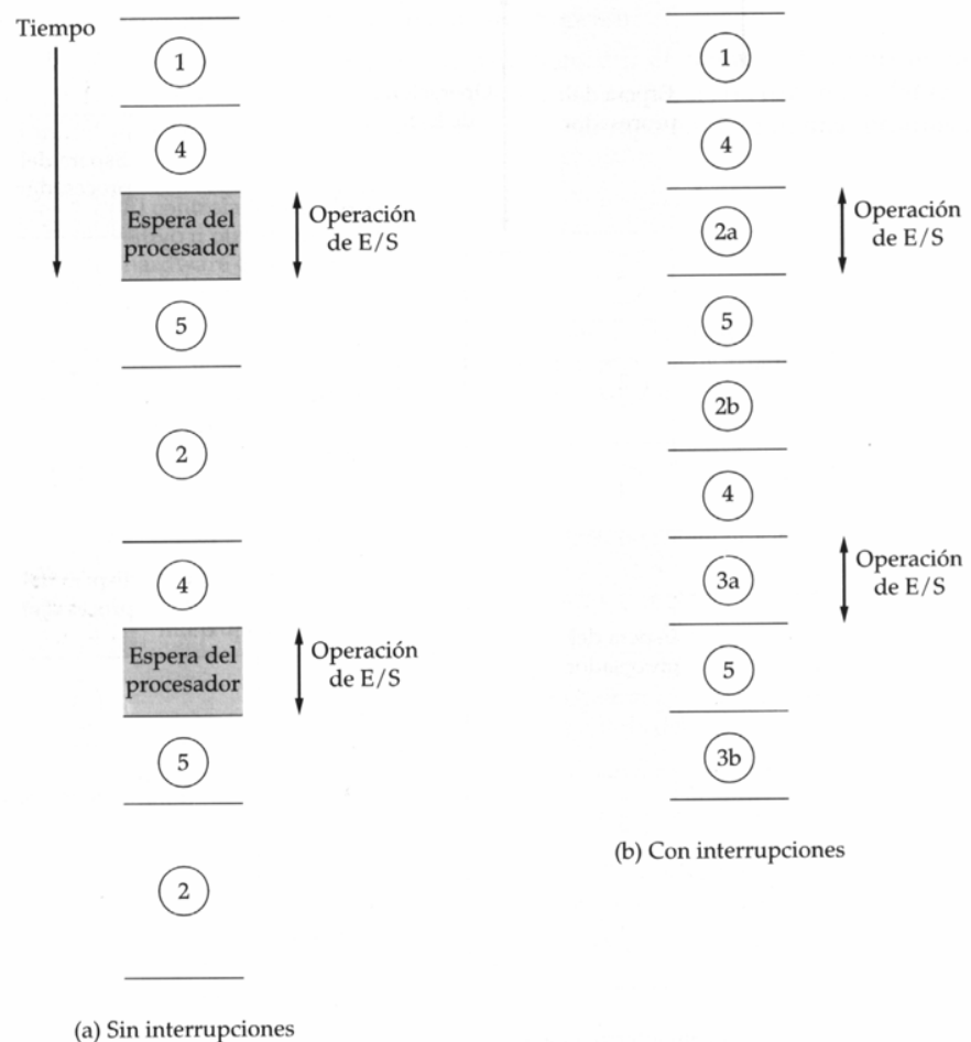
FIGURA 1.8 Diagrama de tiempos de un programa; espera corta de E/S
