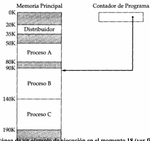
FIGURA 3.1 instantánea de un ejemplo de ejecución en el momento 18 (ver figura 3.3)
