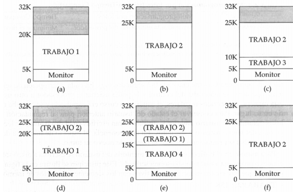
FIGURA 2.9 Funcionamiento del CTSS
