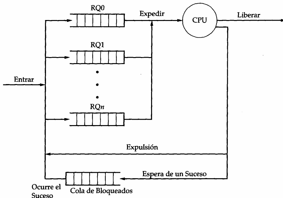
FIGURA 8.4 Planificación por prioridades
