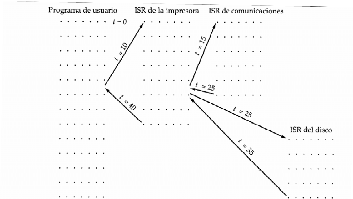
FIGURA 1.13 Ejemplo de secuencia de tiempo para interrupciones múltiples [TANE90]
