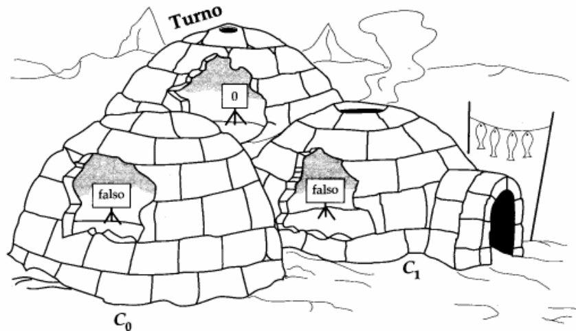
FIGURA 4.5 Una solución de tres iglúes a la exclusión mutua
