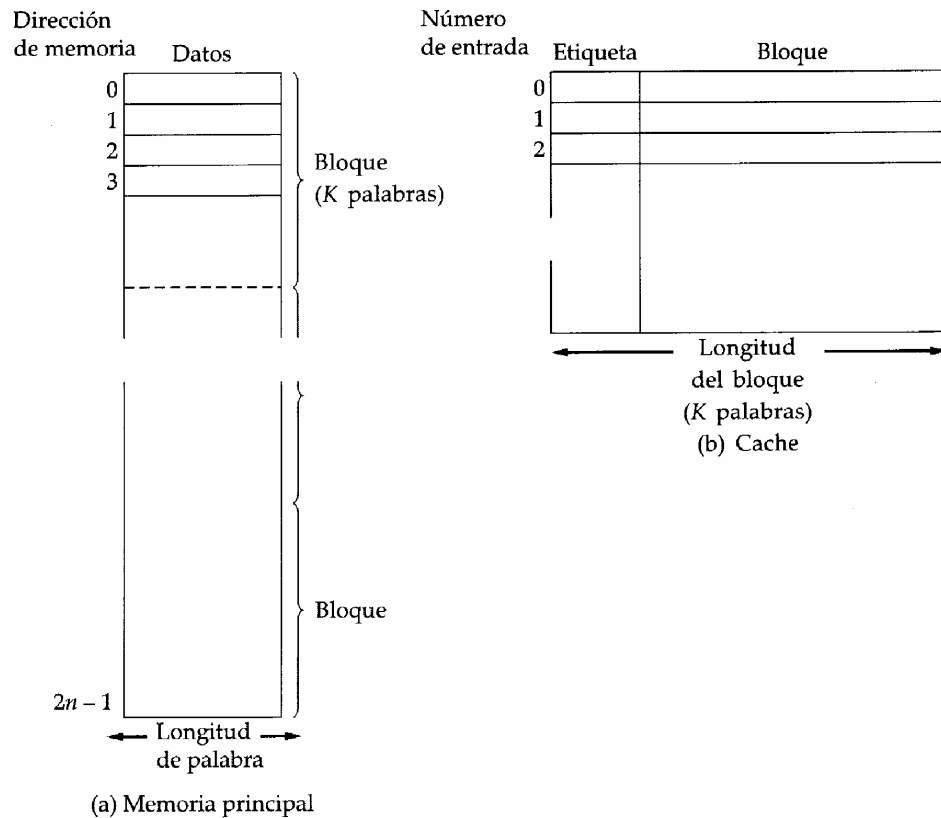
FIGURA 1.19 Estructura de cache/memoria principal
