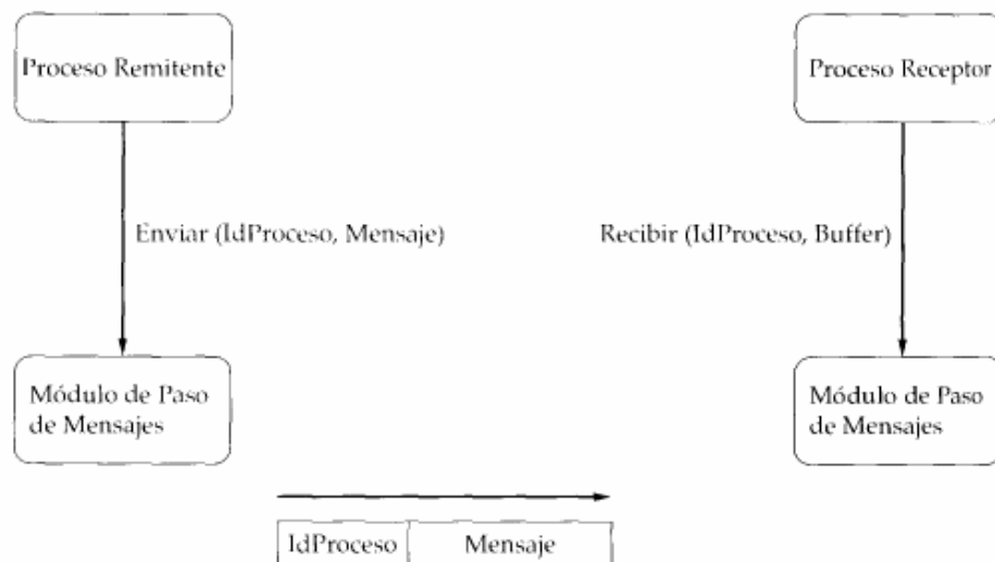
FIGURA 12.23 Primitivas básicas de paso de mensajes
