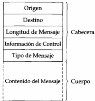
FIGURA 4.26 Formato típico de mensaje
