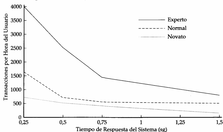
FIGURA 8.20 Resultados del tiempo de respuesta para gráficos de alto rendimiento
