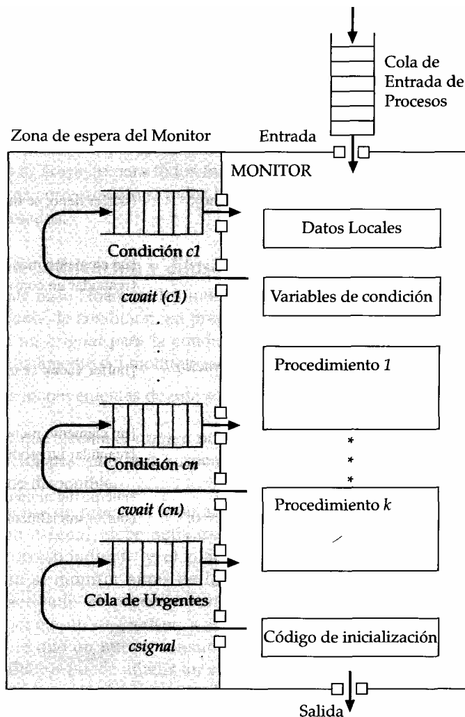
FIGURA 4.23 Estructura de un monitor
