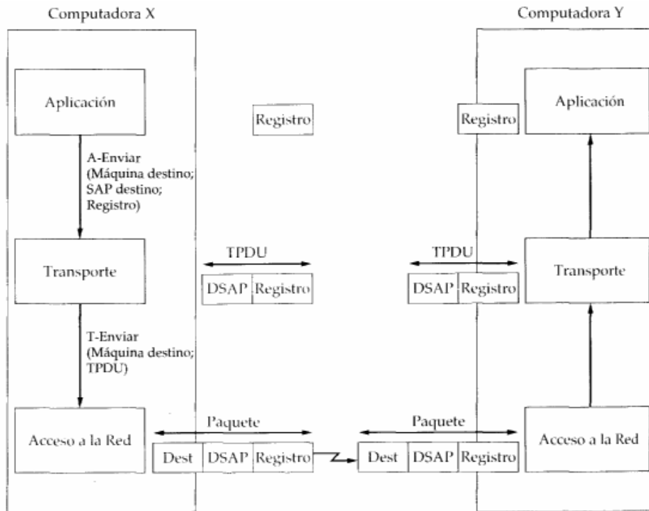
FIGURA 12.5 Operación en una arquitectura de comunicaciones
