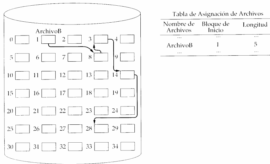
FIGURA 11.9 Asignación encadenada
