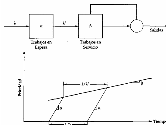
FIGURA 8.19 Round-robin egoísta
