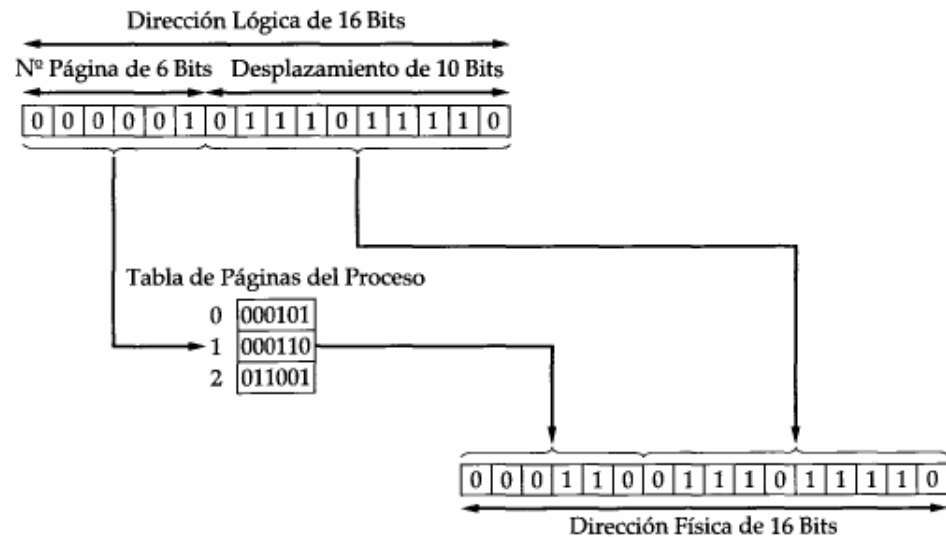
(a) Paginación
