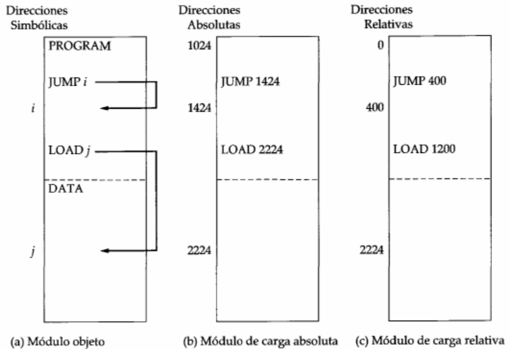
FIGURA 6.13 Módulos de carga absolutos y reubicables
