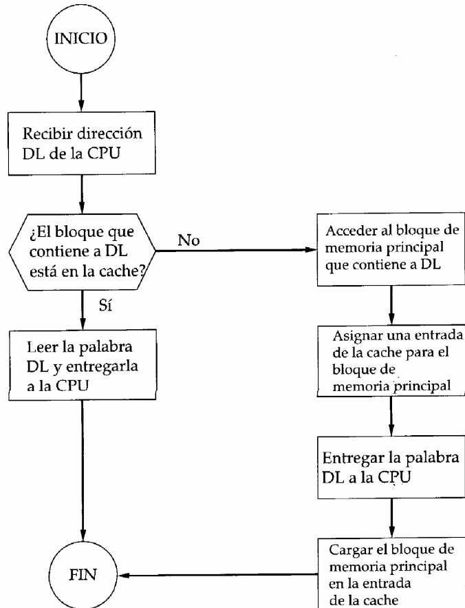
FIGURA 1.20 Operación de lectura de la cache
