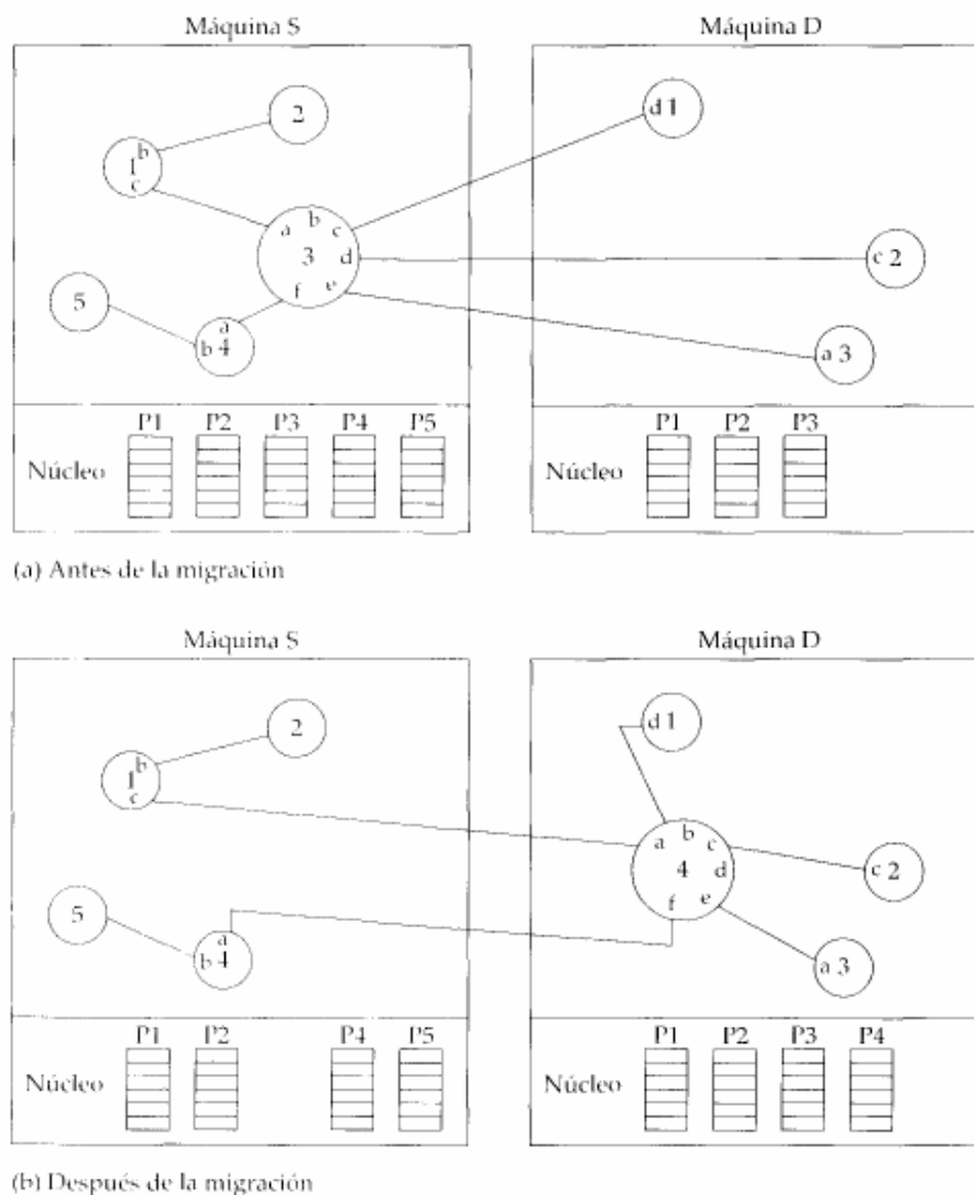
FIGURA 13.1 Ejemplo de migración de procesos
