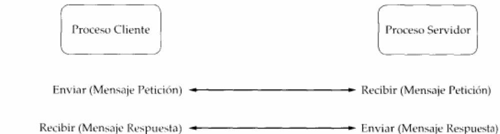
FIGURA 12.22 Paradigma del proceso distribuido mediante envío de mensajes
