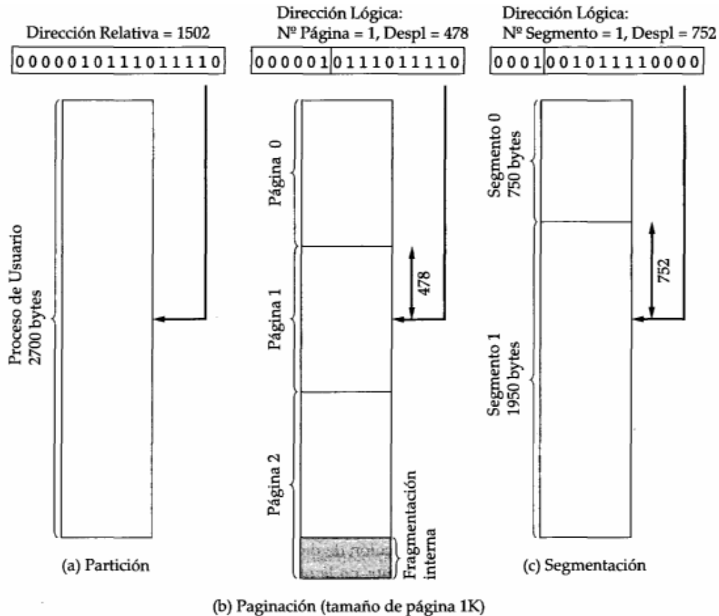
FIGURA 6.9 Direcciones Lógicas
