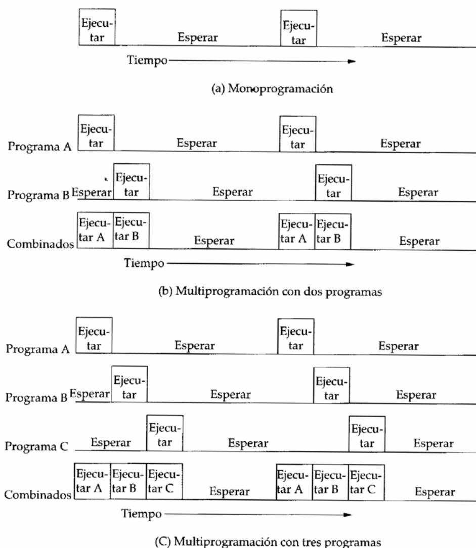
FIGURA 2.6 Multiprogramación
