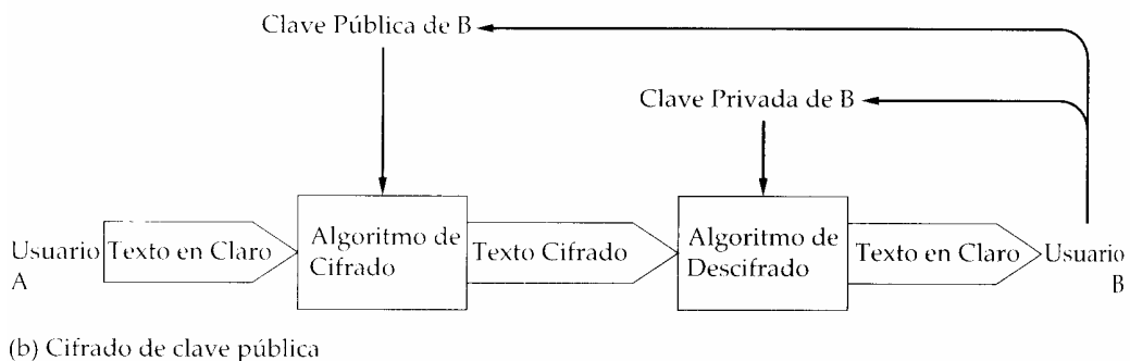
FIGURA 14.21 Cifrado
