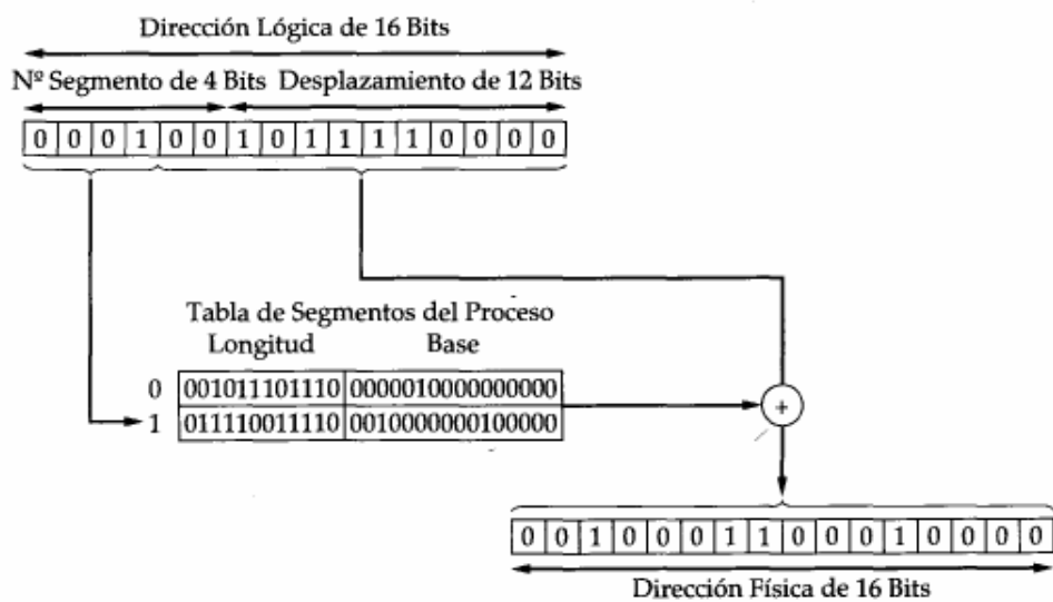
(b) Segmentación
