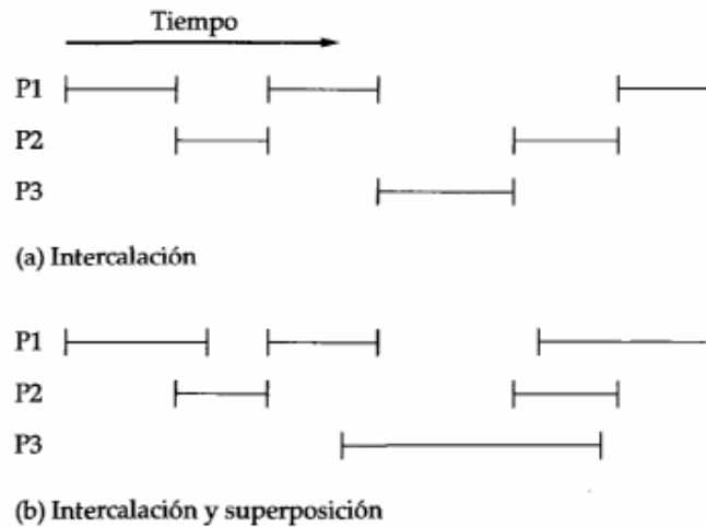
FIGURA 4.1 La ejecución de procesos concurrentes
