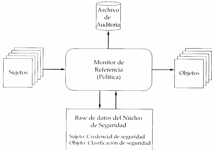
FIGURA 14.14 Concepto de monitor de referencia
