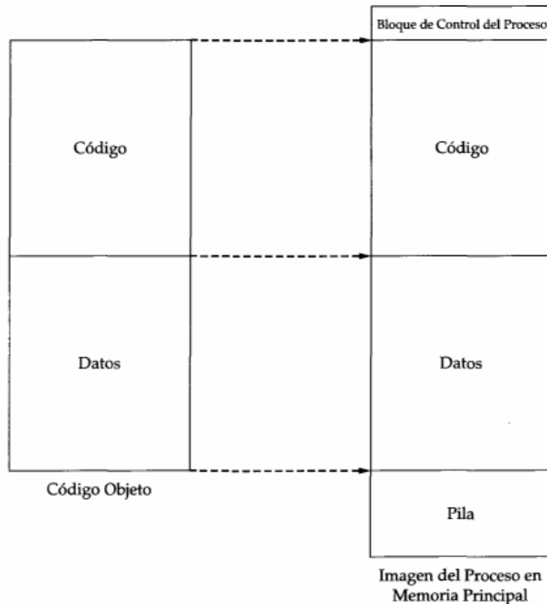
FIGURA 6.11 La función de carga
