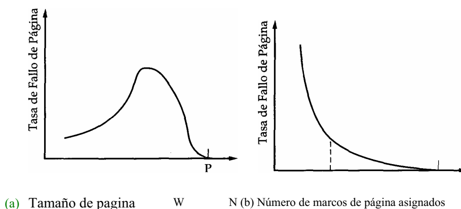
FIGURA 7.9 Comportamiento típico de la paginación en un programa
