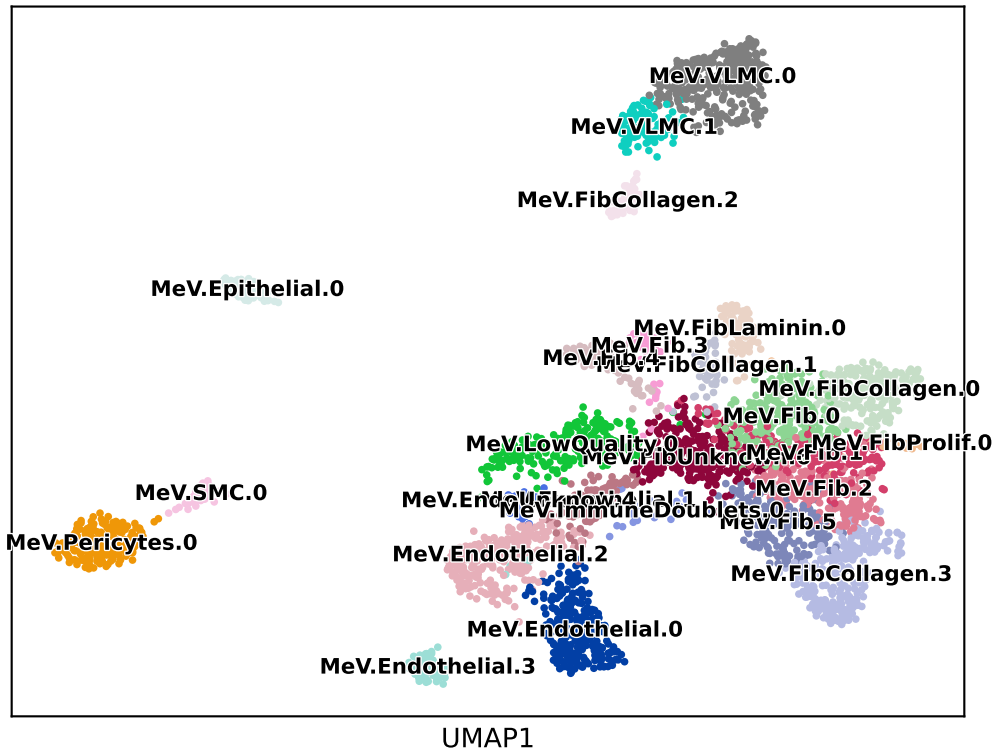
UMAP - leiden_fusion
