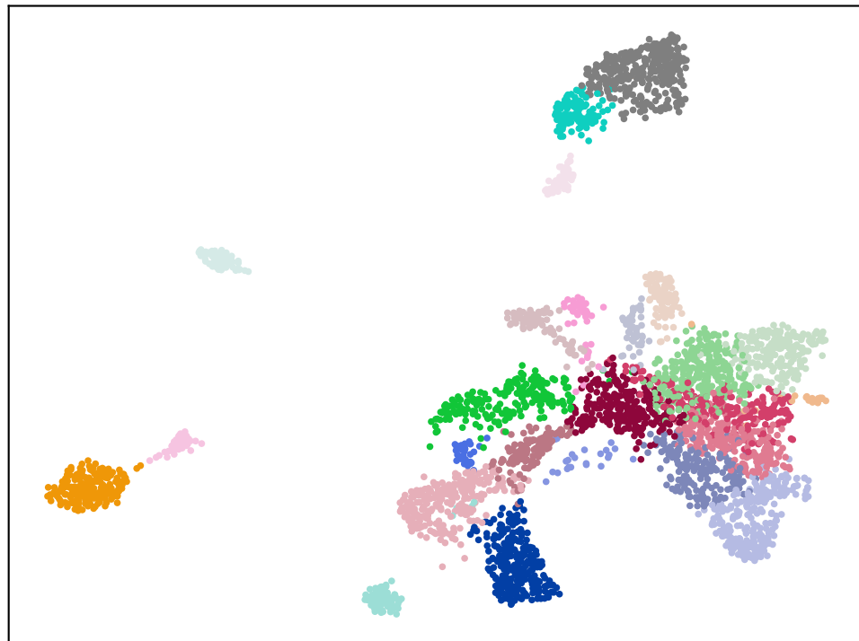
UMAP - leiden_fusion
