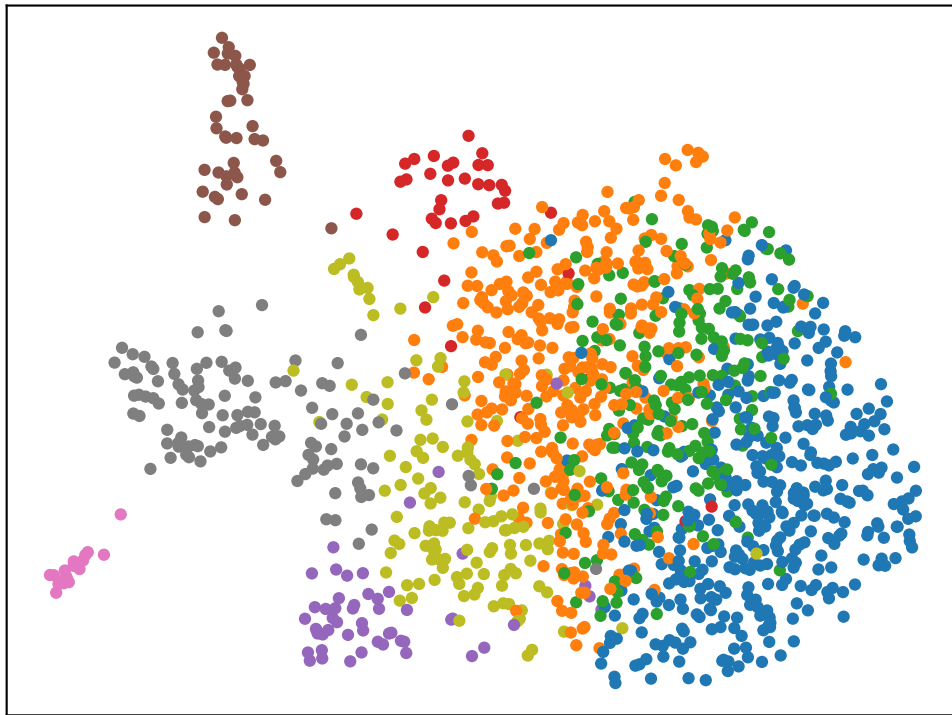
UMAP - leiden_fusion
