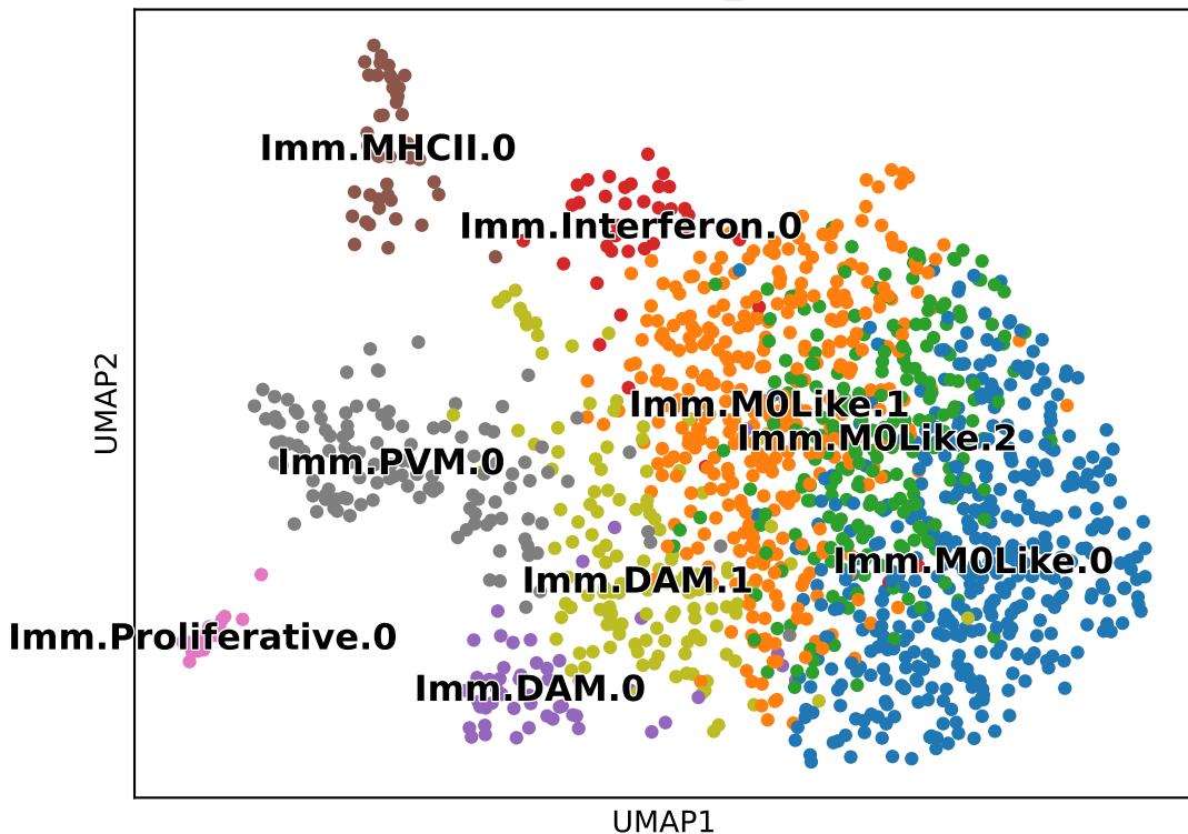
UMAP - leiden_fusion
