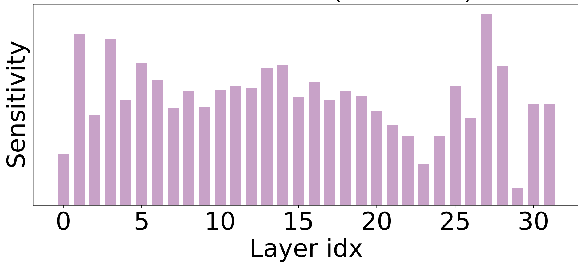
CommenSense (LLaMA-7B)
