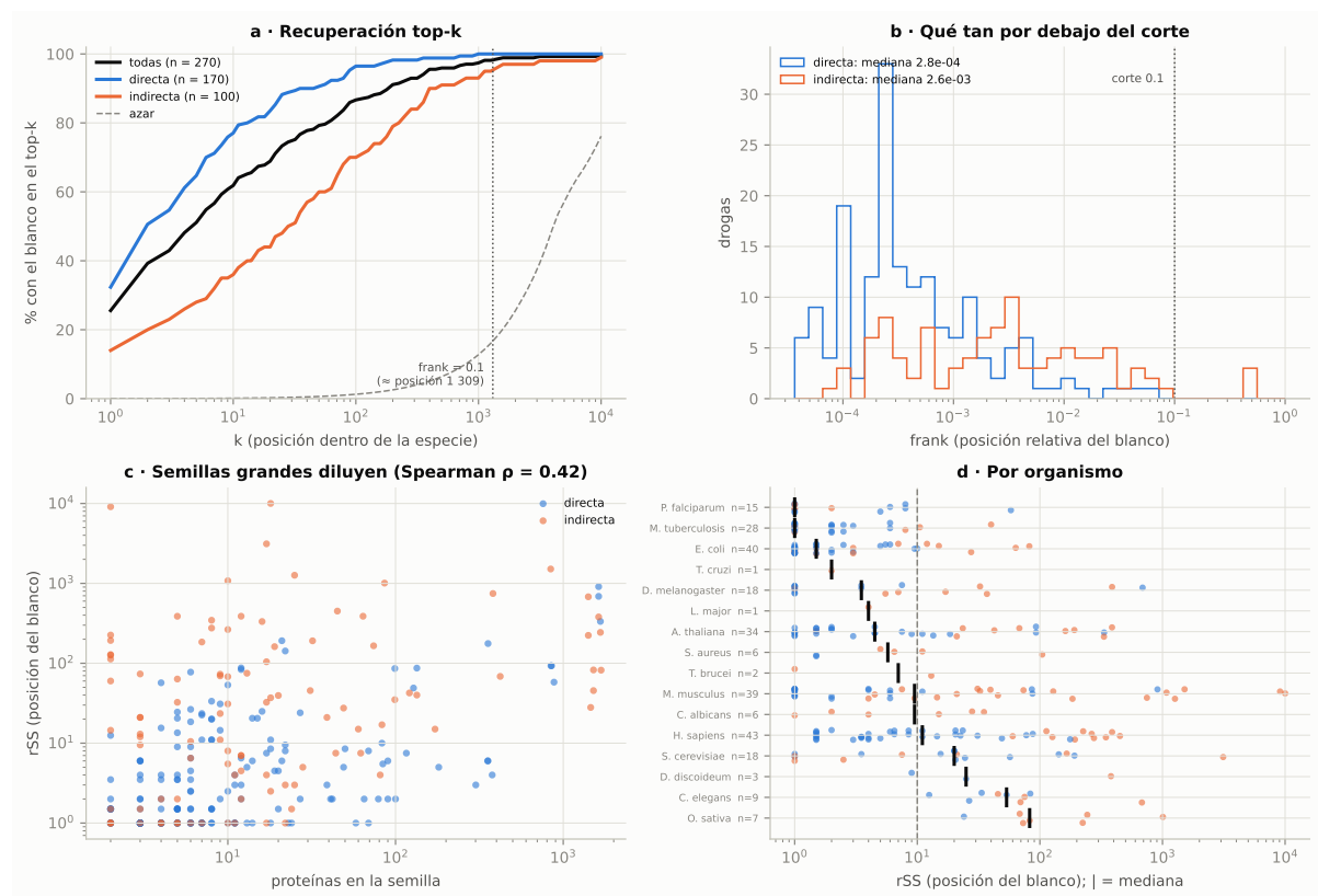
Figura 10: Las 270 pseudohuérfanas con semilla informativa. (a) Fracción con el blanco entre las k primeras proteínas de su organismo, frente al azar; la línea punteada es el corte \text{frank} = 0.1 . (b) \text{frank} en escala logarítmica. (c) Tamaño de la semilla contra posición del blanco. (d) Posición por organismo; la barra es la mediana.
