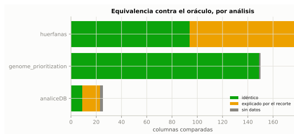
Figura 12: Columnas comparadas contra el oráculo v4, por análisis. Verde: idéntica; ámbar: cambio explicado por el recorte; rojo sería una discrepancia.
