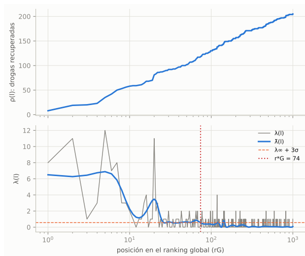
Figura 11: Arriba: compuestos cuyo blanco verdadero cae antes de la posición l del ranking global. Abajo: su derivada, suavizada, y el umbral \lambda_\infty + 3\sigma que define r_G^* .
