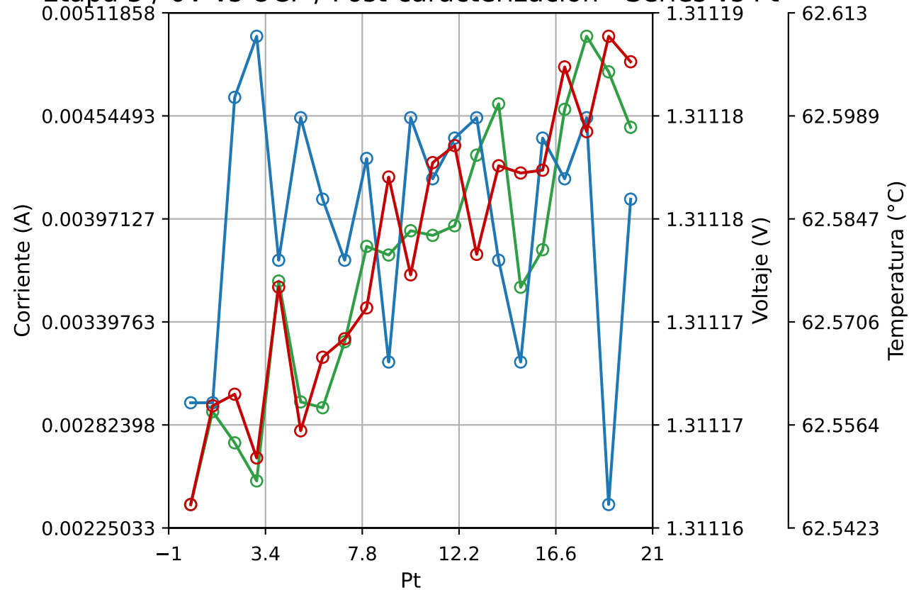
Etapa 5 / 0V vs OCP / Post-caracterización - Series vs Pt
