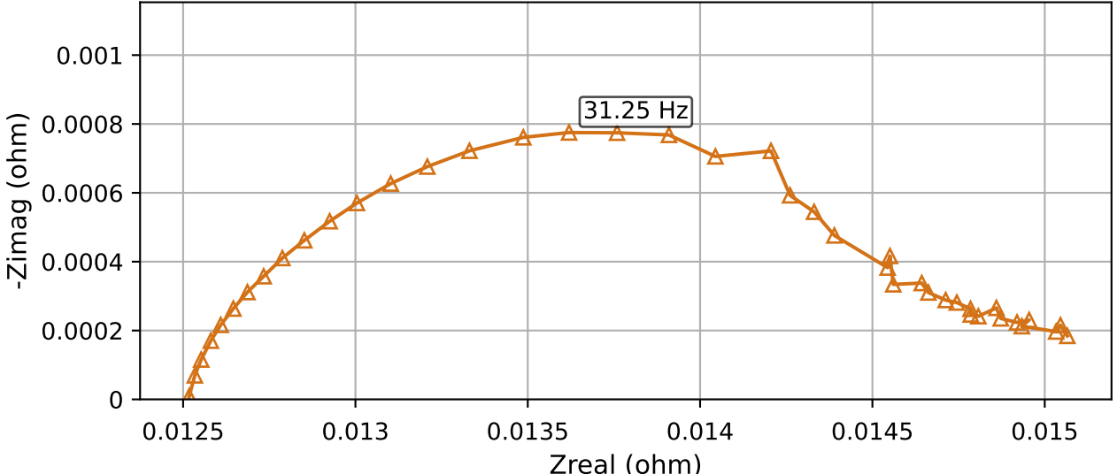
Etap 5 / 18A / 1,81696V
