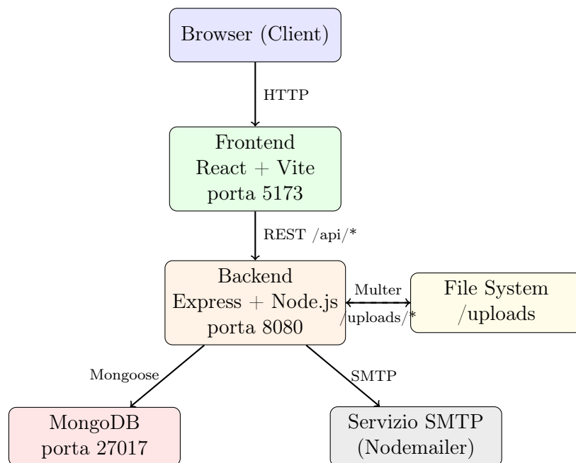
Figure 2: Architettura di deploy di TrentoParking
