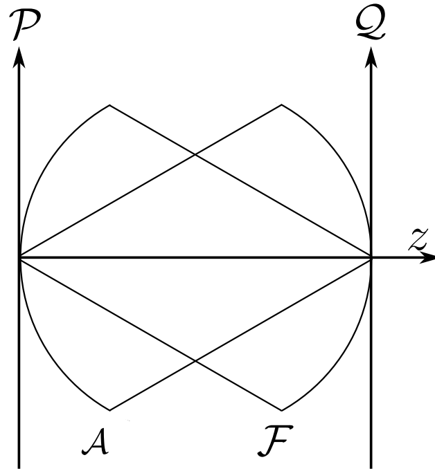
Figura 1.4: Esquema de las esferas cardinales cofocales, con radios equivalentes a la propagación z del campo.
