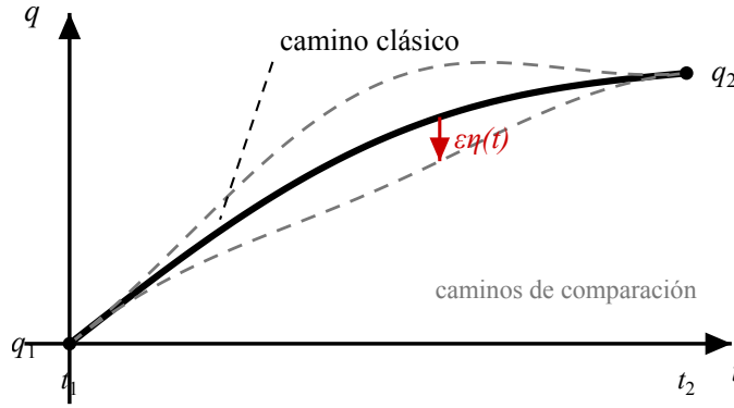
Figura 3.1: El camino efectivo y los caminos de comparación que se usan para variarlo. Todos parten de la misma configuración inicial y llegan a la misma final, de modo que la desviación \varepsilon\eta(t) se anula en los dos extremos.
