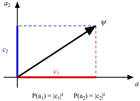
Figura 4.1: Contenido geométrico de la regla de Born. El estado se descompone en la base propia del observable y la probabilidad de cada resultado es el cuadrado del módulo de la componente correspondiente.
