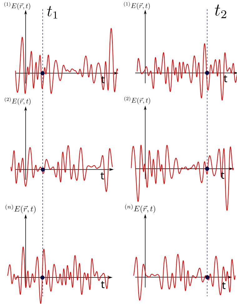
Figura 2.5: Evolución de las realizaciones al propagar el campo eléctrico.
