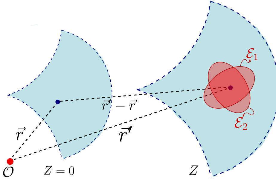
Figura 2.3: Propagación del campo eléctrico desde un plano Z = 0 hasta un plano Z , donde cada punto del frente de onda lleva su elipse de polarización media.
