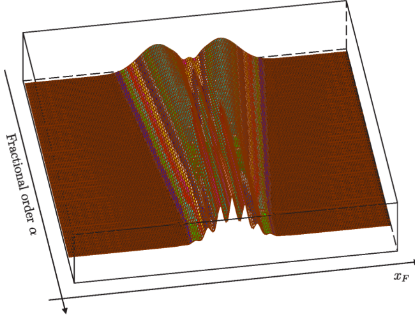
Figura 8.5: Simulación de varias distribuciones de densidad de probabilidad a una distancia z .
