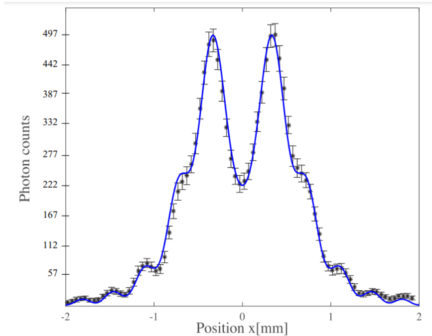
Figura 8.4: Los datos experimentales se superpusieron a la curva azul que es la densidad de probabilidad normalizada, |\Psi(x, z)|^2 , obtenido por simulación computacional.
