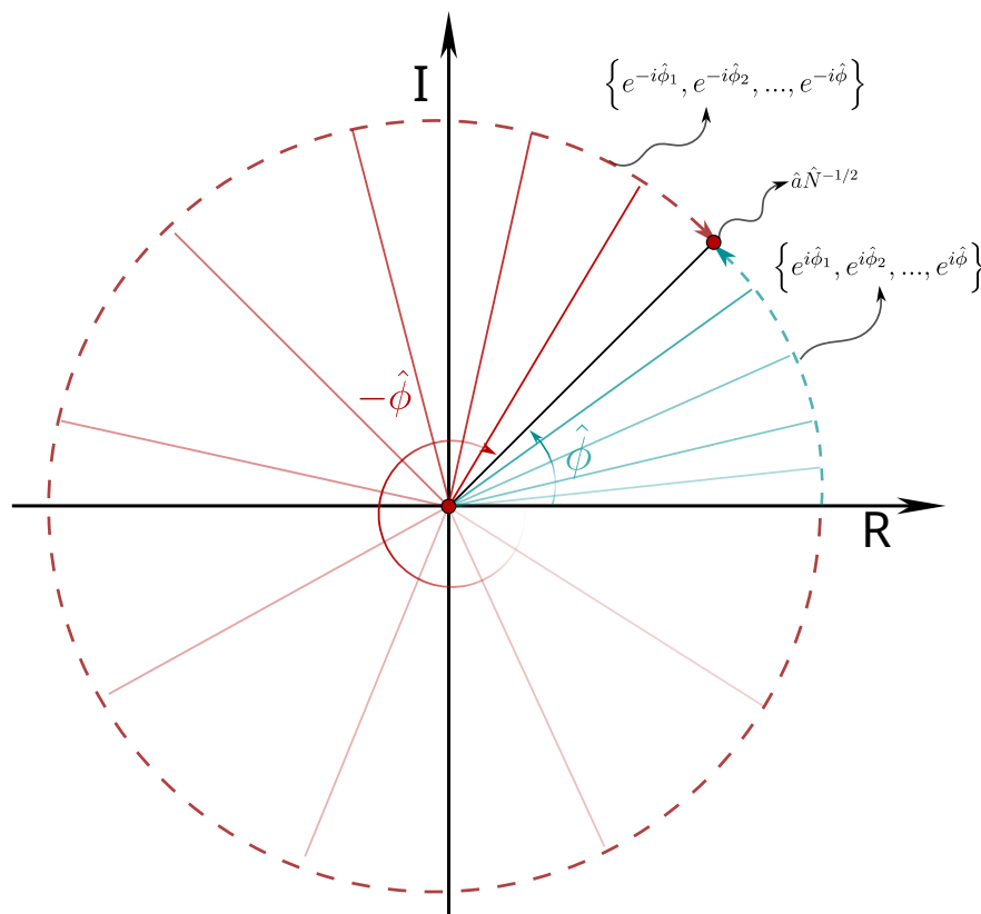
Figura 7.1: Representación esquemática sobre el plano complejo \mathbb{C}^2 en el cual se ve el efecto del exponencial de fase e^{i\hat{\phi}} y de su adjunto e^{-i\hat{\phi}} .
