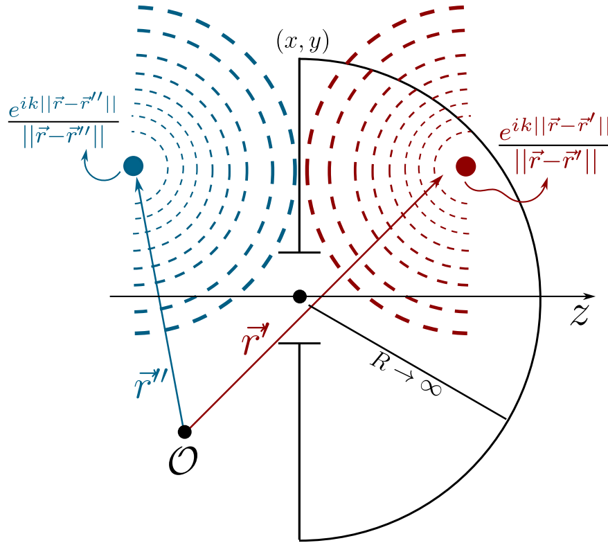
Figura 1.2: Representación de las funciones de Green para fuentes puntuales. Bajo estas condiciones de frontera, las funciones de Green se comportan como cargas puntuales, una imagen especular de la otra.
