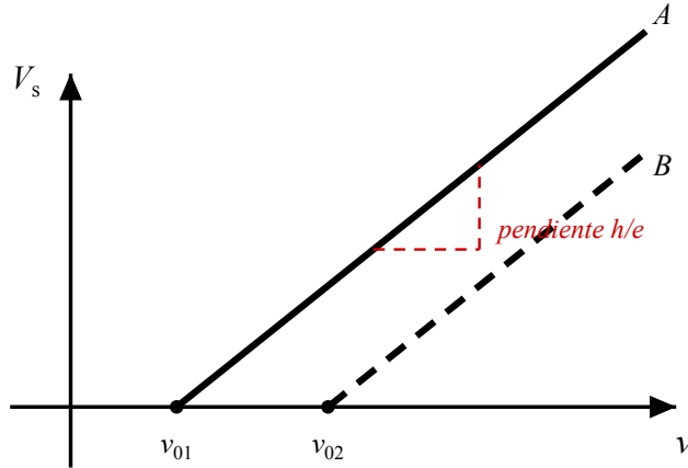
Figura 5.3: Potencial de frenado frente a la frecuencia de la luz incidente para dos metales distintos. La predicción de Einstein es que las dos rectas sean paralelas, con pendiente h/e común, y que solo difieran en la frecuencia umbral.
