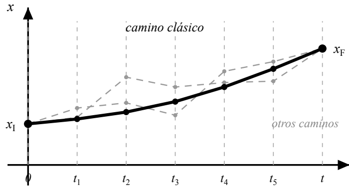
Figura 3.4: Construcción de la integral de camino. El intervalo se divide en rodajas y se integra sobre todas las posiciones intermedias posibles, de manera que a la amplitud contribuyen por igual el camino clásico y todos los caminos quebrados que lo rodean.
