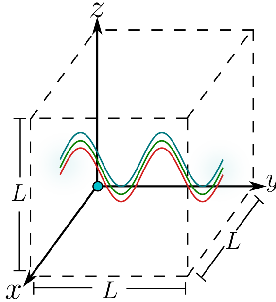
Figura 5.6: Campo eléctrico en todos sus modos confinado en una cavidad con paredes conductoras perfectas
