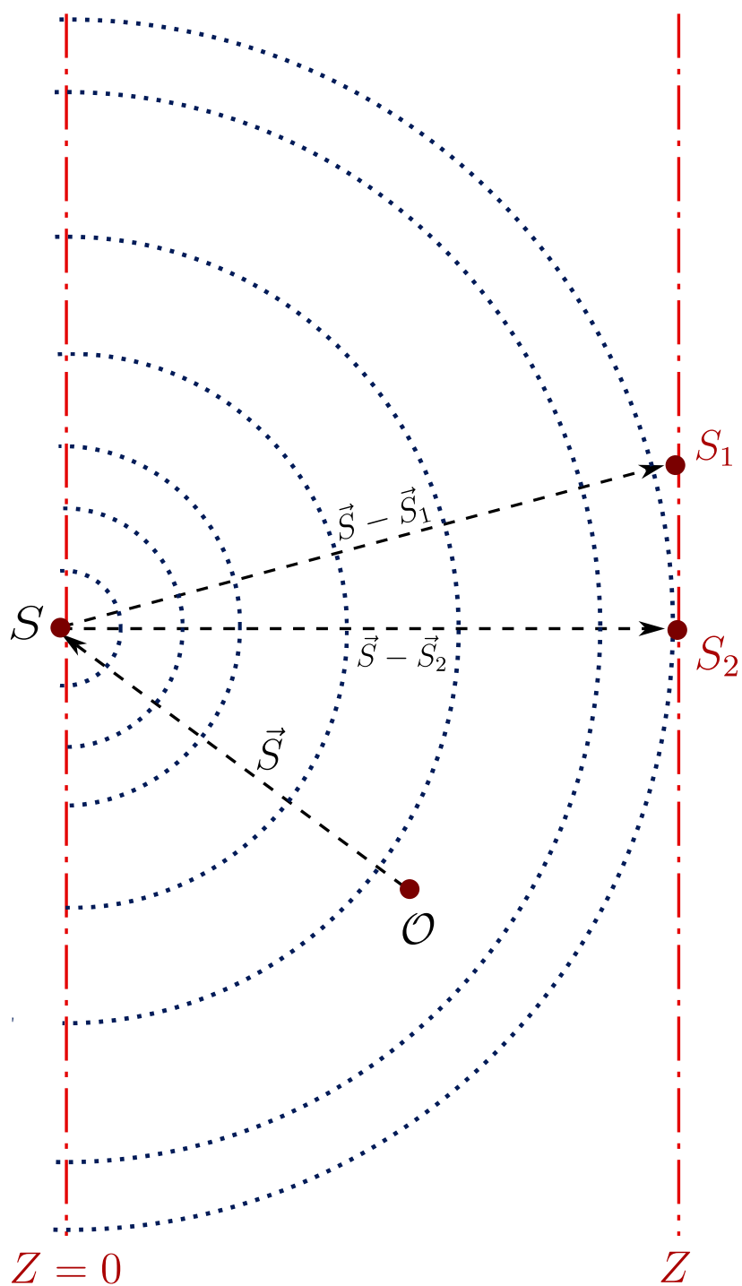
Figura 2.6: La coherencia mutua propagada al campo lejano es la transformada de Fourier de la distribución de intensidad \Gamma_0(\vec{S}) de la fuente.
