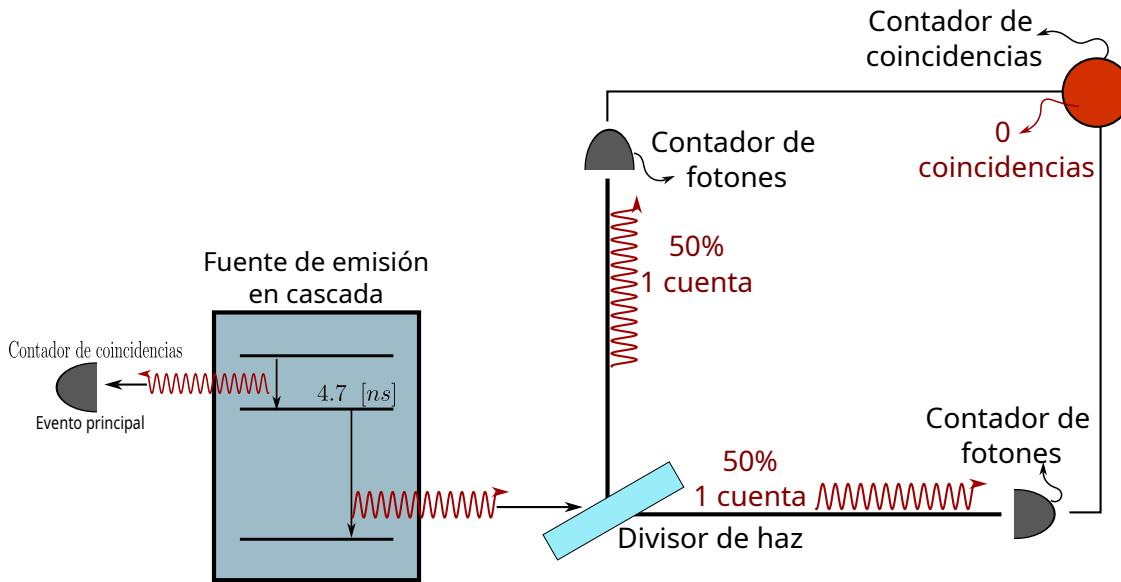
Figura 5.5: Esquema experimental del estudio efectuado por Philippe Grangier, Gérard Roger y Alain Aspect en 1986. La detección del primer fotón de la cascada abre una ventana temporal durante la cual el segundo fotón, preparado en un estado de un solo cuanto, incide sobre un divisor de haz equilibrado con un detector en cada salida.
