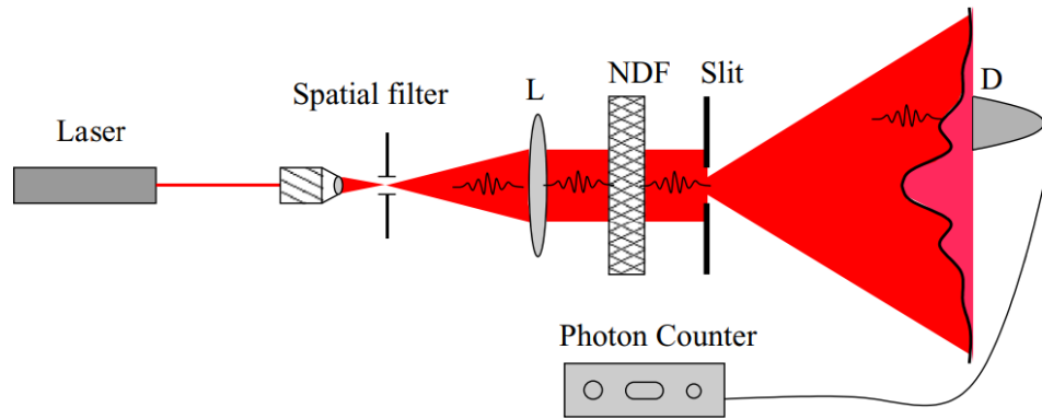
Figura 8.3: Configuración experimental.
