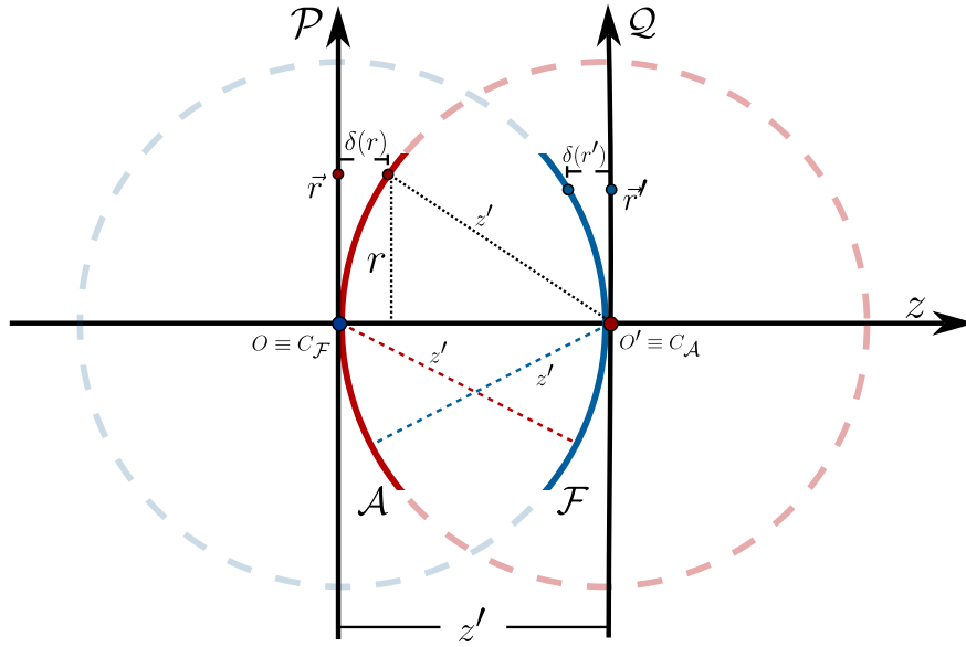
Figura 1.4: Geometría de las dos esferas confocales. El casquete \mathcal{A} es tangente al plano emisor \mathcal{P} en el vértice O y tiene su centro de curvatura en O' , mientras que el casquete \mathcal{F} es tangente al plano receptor \mathcal{Q} en O' y tiene su centro de curvatura en O , de modo que ambos radios son iguales a la distancia de propagación z' . Leída sobre estas dos superficies, la propagación de Fresnel se reduce a una transformación de Fourier exacta, que en el lenguaje de la transformada fraccionaria de Fourier de la Sección 1.7 corresponde al orden \alpha = \pi/2 .
