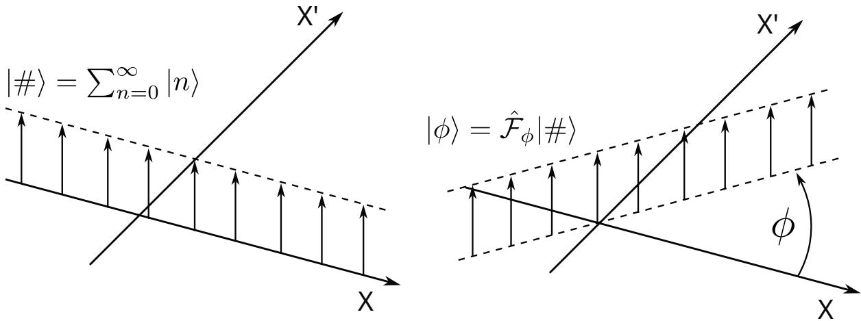
Figura 7.4: Representación gráfica de los estados de fase como la rotación de los estados numeral |\# \rangle
