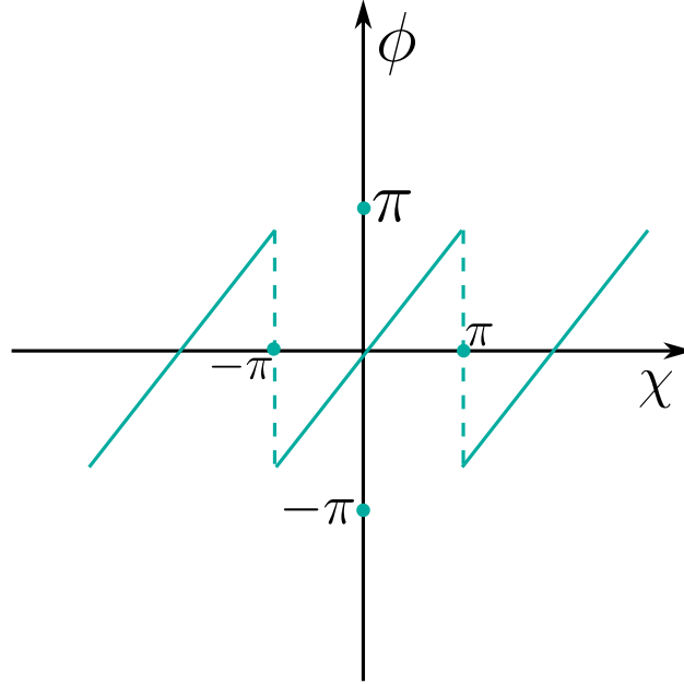
Figura 7.2: Relación entre el operador de ángulo restringido \hat{\phi} con -\pi < \hat{\phi} \leq \pi y el operador de ángulo \hat{\chi} .
