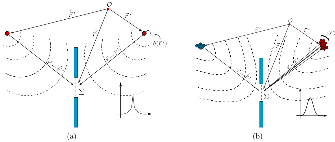
Figura 8.2: (a) Problema de Green usando una distribución \delta de Dirac. (b) Problema propuesto para una distribución arbitraria.
