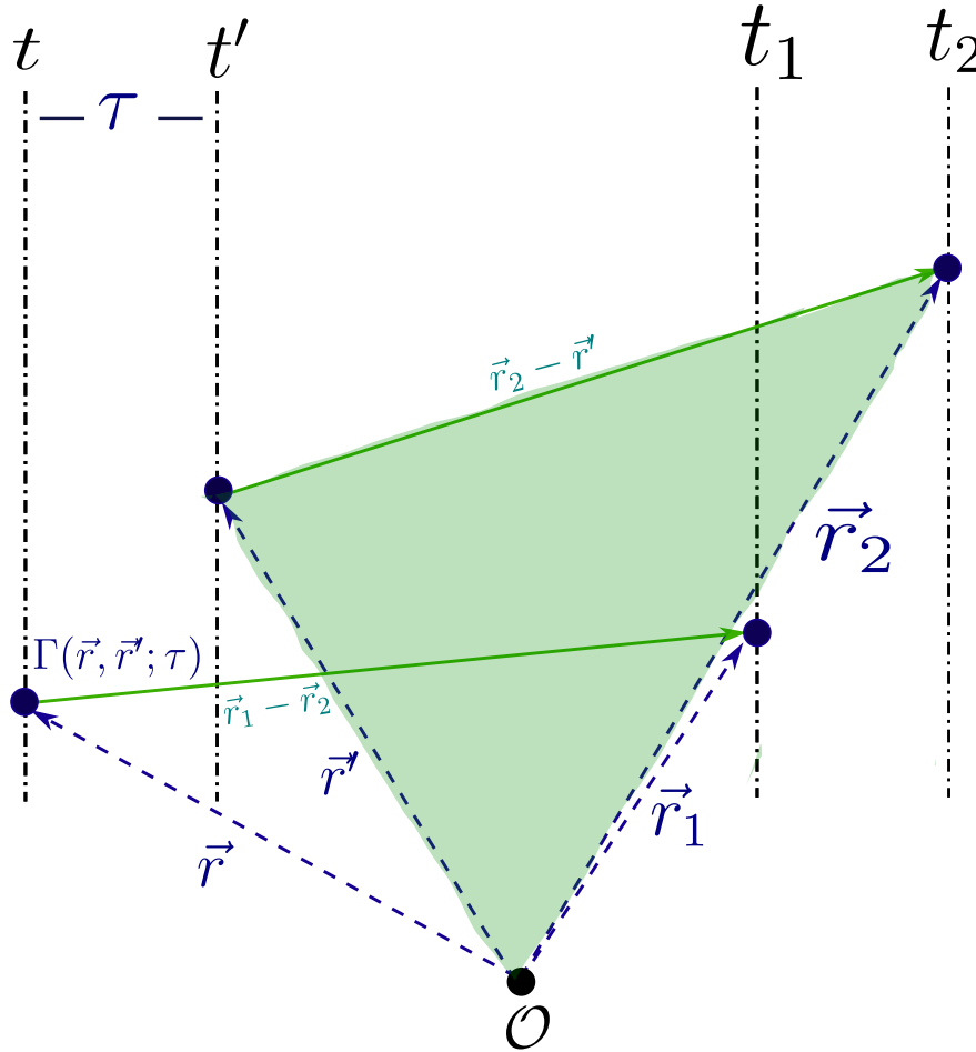
Figura 2.4: Propagación de la función de coherencia entre dos puntos \vec{r}, \vec{r}' en el plano inicial hasta la coherencia entre dos puntos \vec{r}_1, \vec{r}_2 en el plano de observación.
