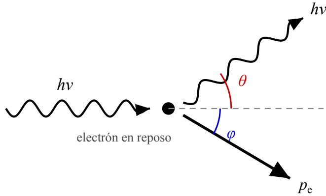
Figura 5.4: Geometría de la dispersión de Compton. El cuanto incidente cede parte de su energía y de su momento al electrón, que retrocede, y sale con una frecuencia menor y desviado un ángulo \theta .
