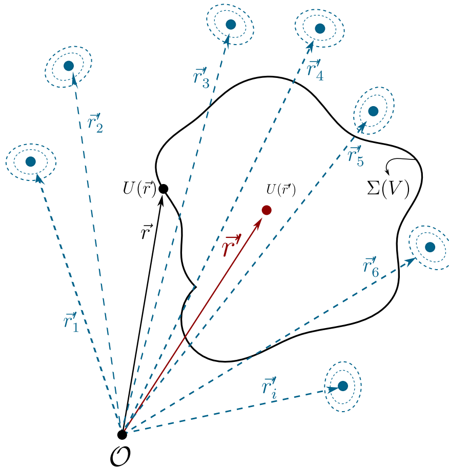
Figura 1.1: Sobre la frontera \Sigma(V) se muestra la contribución de las componentes del campo U(\vec{r}) ; dentro de la región, el campo total se construye a partir de la contribución de todos los puntos de la frontera. Se pueden añadir infinitas cargas puntuales de Green de naturaleza de propagación arbitraria; la condición para la invariancia de la ecuación (1.18) es que estas cargas imagen se encuentren fuera de \Sigma(V) .
