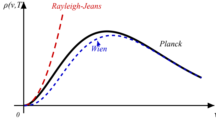
Figura 5.2: Densidad espectral de la radiación de un cuerpo negro a temperatura fija. La ley de Rayleigh y Jeans crece sin límite con la frecuencia, la de Wien falla en el infrarrojo, y la de Planck coincide con cada una de ellas en su propio dominio de validez.
