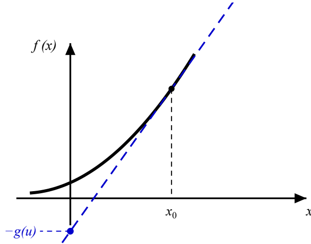
Figura 3.2: Lectura geométrica de la transformada de Legendre. El valor -g(u) es la ordenada en el origen de la recta tangente de pendiente u , de manera que describir la curva por sus tangentes contiene la misma información que describirla por sus puntos.
