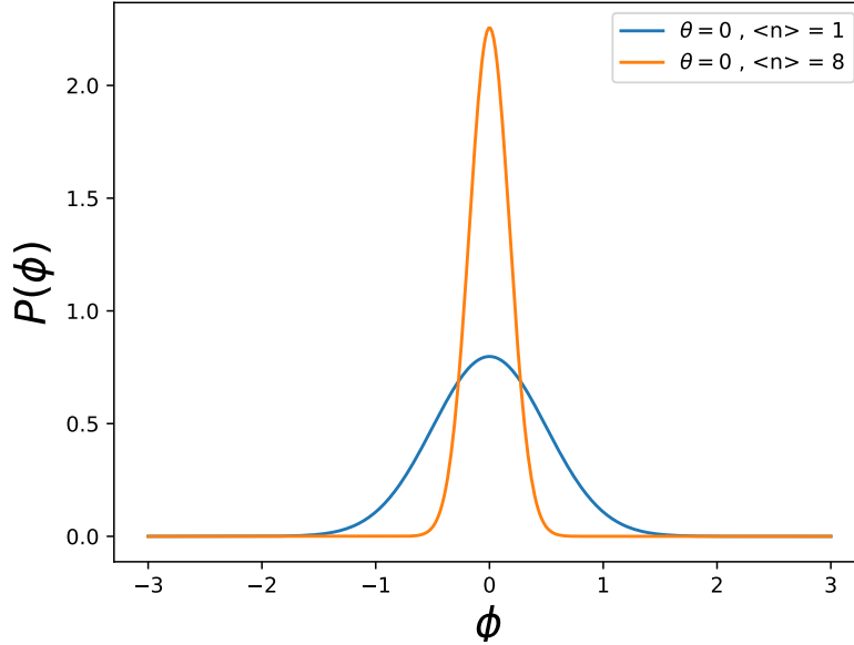
Figura 5.10: Distribución de fase para los estados coherentes, en los cuales se ilustran dos estados centrados en el origen y con dos valores medios del número de cuantos de energía distintos.
