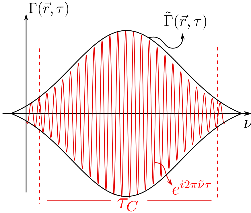
Figura 2.2: Representación gráfica de la función de coherencia de banda angosta. En negro se muestra la envolvente \tilde{\Gamma}(\vec{r}, \tau) , y en rojo las oscilaciones e^{i2\pi\tilde{\nu}\tau} . Estas oscilaciones están confinadas dentro de algo conocido como el tiempo de coherencia \tau_C , que veremos más adelante.
