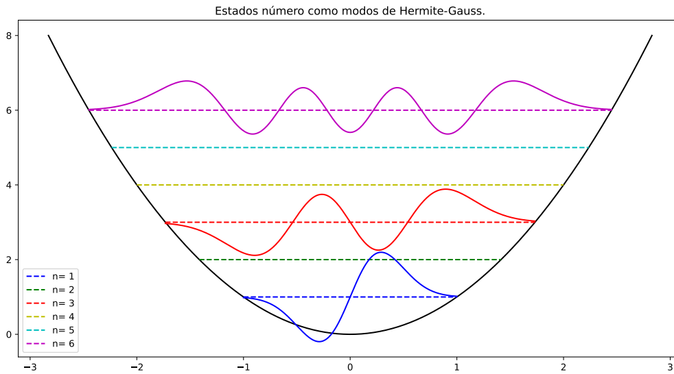
Figura 5.7: Se representan gráficamente los primeros 6 niveles de energía para un oscilador armónico cuántico, en este caso correspondiente al hamiltoniano del campo electromagnético. Para los niveles de energía; 1, 3, 6 se ilustran estos estados en la base de posición, los cuales corresponden a las funciones de Hermite-Gauss.
