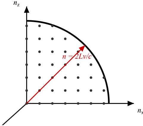
Figura 5.1: Conteo de los modos de la cavidad. Cada terna de enteros no negativos (n_x, n_y, n_z) etiqueta un modo, y los que tienen frecuencia menor que \nu llenan el octante de radio n = 2L\nu/c , de manera que su número es el volumen de ese octante.
