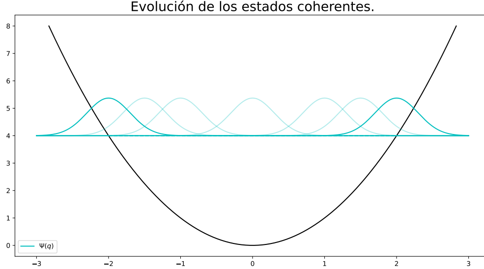
Figura 5.8: Los estados coherentes oscilan armónicamente a lo largo del potencial entre los puntos de retorno clásicos. Debido a la forma de estos estados, que sus autovalores con el operador de aniquilación correspondan a una representación compleja de los valores medios de los operadores cuadratura apunta a que físicamente estos estados representan la oscilación bien dirigida de la energía de la radiación.
