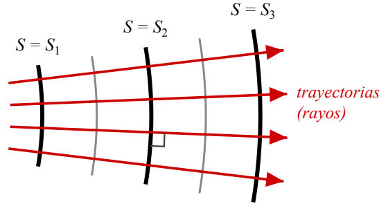
Figura 3.3: Superficies de acción constante y trayectorias mecánicas. El momento es el gradiente de S , de modo que las trayectorias cortan perpendicularmente a los frentes, exactamente como los rayos luminosos cortan a los frentes de onda.
