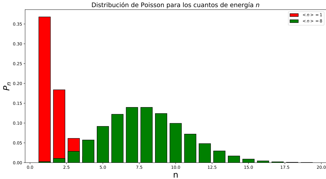
Figura 5.9: Densidad de probabilidad para los estados número coherentes.
