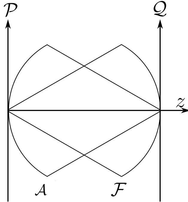
Figura 1.5: Esquema de las esferas cardinales confocales, con radios iguales a la distancia de propagación z' del campo.
