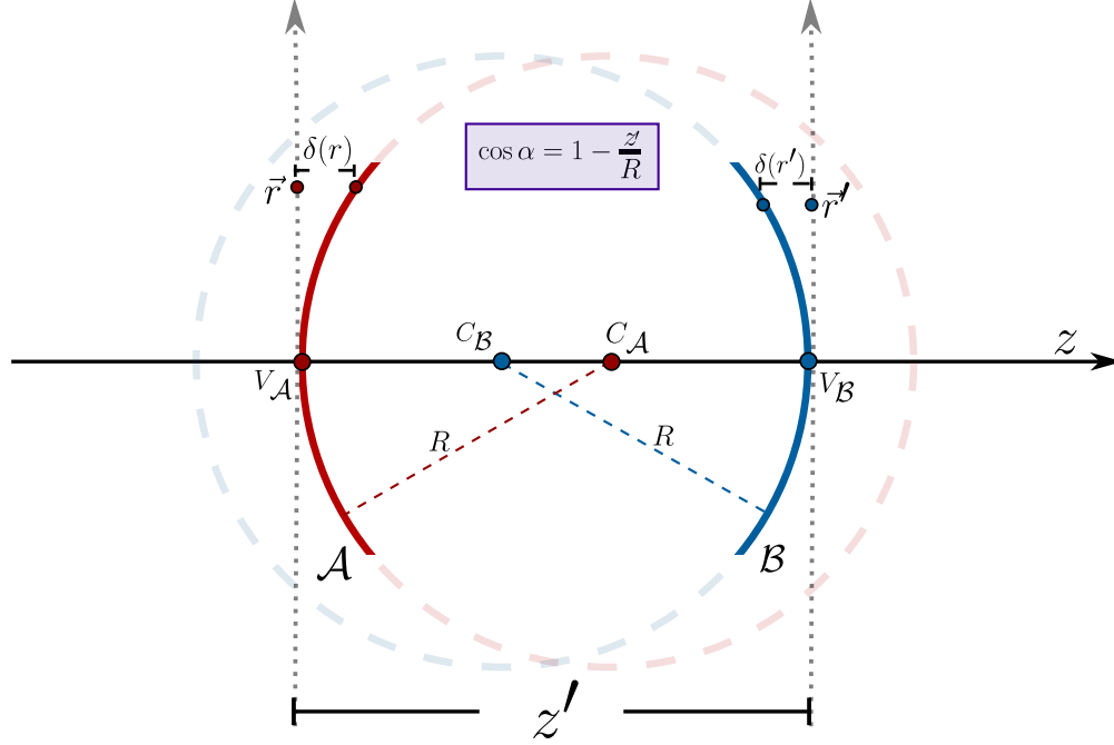
Figura 1.6: Las dos esferas cardinales de radio R asociadas a una propagación sobre la distancia z . El casquete emisor \mathcal{A} es tangente a su plano en V_A con su centro de curvatura aguas abajo en C_A , de abscisa R , y el casquete receptor \mathcal{B} es tangente a su plano en V_B con su centro aguas arriba en C_B , de abscisa z - R , de modo que los dos casquetes se curvan uno hacia el otro. La cantidad \delta es la sagita (1.104). El caso confocal de la Figura 1.4 se recupera cuando R = z , ya que entonces C_A cae sobre V_B y C_B sobre V_A .
