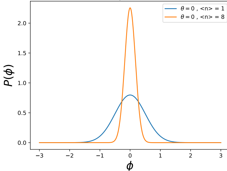
Figura 2.6: Distribución de fase para los estados coherentes, en los cuales se ilustran dos estados centrados en el origen y con dos valores medios del número de cuantos de energía distintos.
