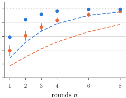
(d) Z memory, placement 2
