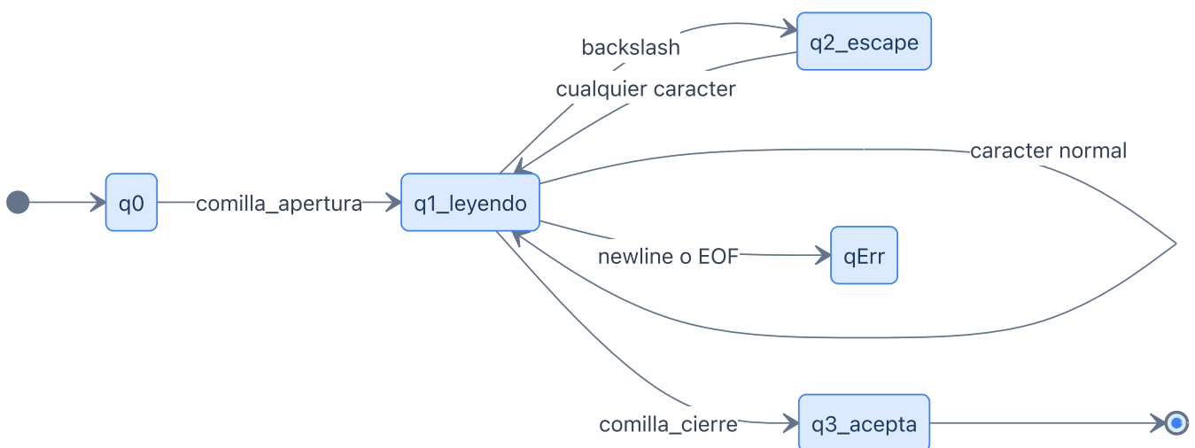
Figura 3: AFD para cadenas (STRING)
