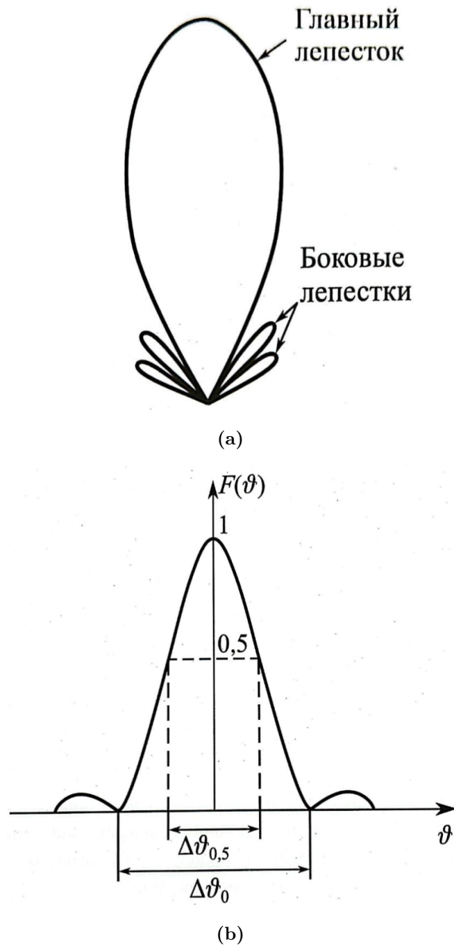
Рис. 1. Диаграмма направленности
