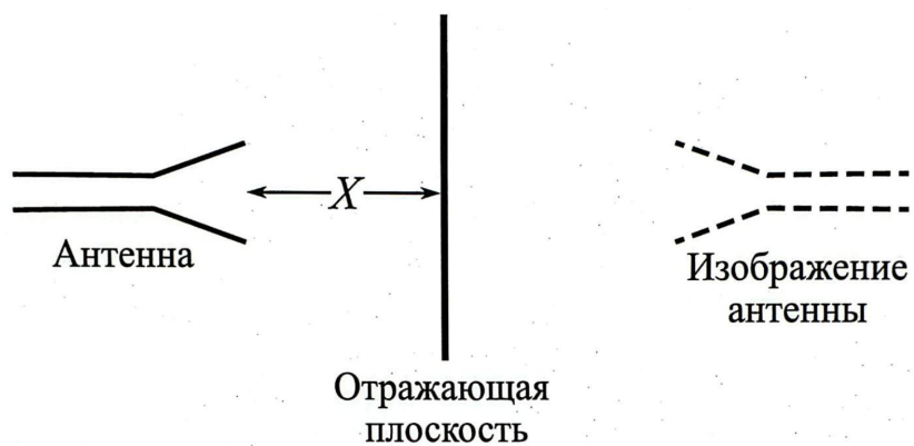
Рис. 2. Метод изображений
