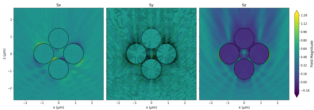
Figura 2: Vector poynting en el campo cercano.
