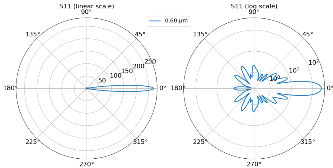
Figura 1: Radiación dispersada en función del ángulo de observación en el campo lejano por 4 esferas formando un cuadrado y un ángulo de 45^\circ .
