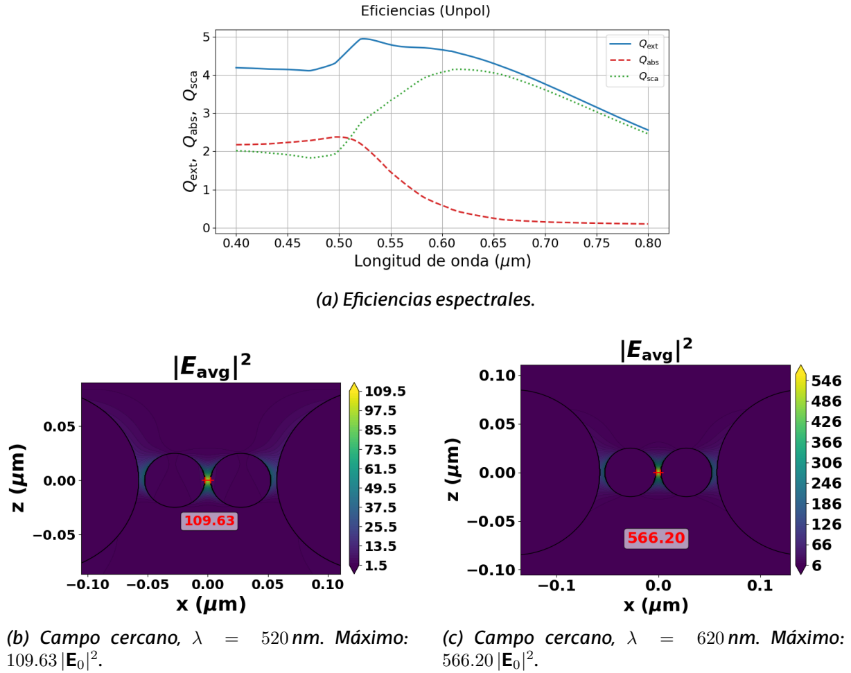
Figura 16: Tetrámero heterogéneo (85–25–25–85 nm) con d = 5 nm. El espectro muestra un pico de extinción en \lambda \approx 520 nm, donde la absorción alcanza su máxima contribución, y un pico dispersor principal en \lambda \approx 620 nm. En ambos casos la zona de concentración se localiza entre las dos esferas pequeñas centrales; a \lambda = 620 nm la intensificación alcanza 566.20 |\mathbf{E}_0|^2 , el valor más alto de todas las configuraciones estudiadas.
