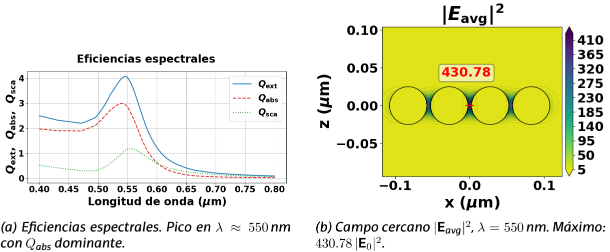
Figura 13: Tetrámero homogéneo con a = 25 nm y d = 5 nm. La resonancia se mantiene en torno a \lambda \approx 550 nm con absorción dominante. La zona de concentración se localiza en el gap central, entre las dos esferas interiores, mientras que los gaps exteriores muestran una intensificación significativamente menor.
