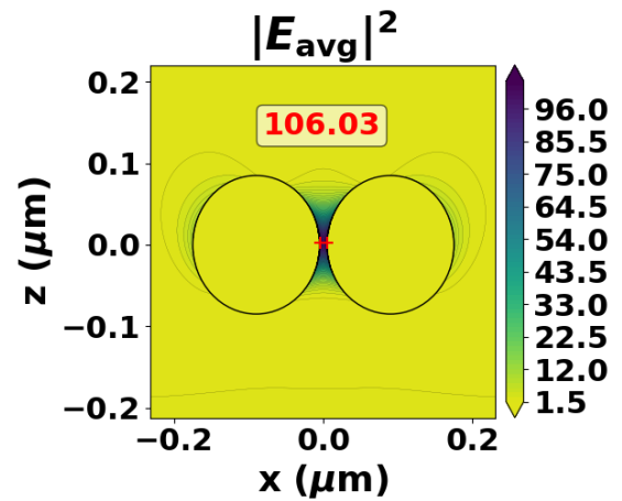
(b) d = 10 \text{ nm} , \lambda = 700 \text{ nm} . Máximo: 106.03 |E_0|^2 .
