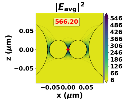
(c) Campo cercano, \lambda = 620 \text{ nm} . Máximo: 566.20 |E_0|^2 .
