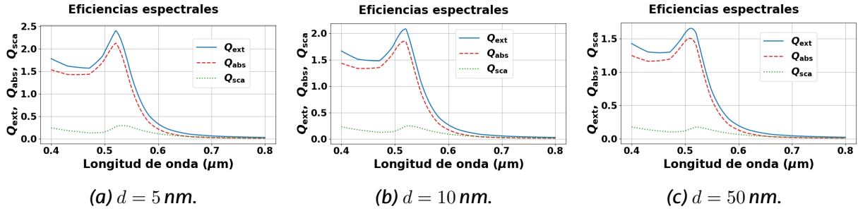
Figura 5: Eficiencias espectrales del dímero con a = 25 nm para tres separaciones. La resonancia permanece en torno a \lambda \approx 520 nm en los tres casos; el acoplamiento incrementa la amplitud del pico sin desplazarlo espectralmente. La absorción sigue siendo el canal dominante de extinción para todos los gaps estudiados. A medida que aumenta d , la amplitud del pico disminuye progresivamente, convergiendo hacia los valores de la esfera individual.
