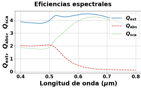
(a) Eficiencias espectrales.
