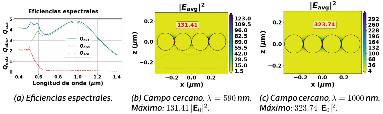
Figura 14: Tetrámero homogéneo con a = 85 nm y d = 5 nm. El espectro muestra tres picos: uno en torno a \lambda \approx 500 nm, donde la absorción y la dispersión compiten, y dos dominados por la dispersión en torno a \lambda \approx 590 nm y \lambda \approx 1000 nm. A \lambda = 590 nm la zona de concentración ( 131.41 |E_0|^2 ) se localiza en los gaps exteriores. A \lambda = 1000 nm el máximo ( 323.74 |E_0|^2 ) se desplaza al gap central, con los gaps exteriores mostrando una intensificación menor.
