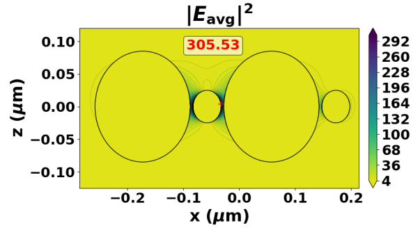
(b) Campo cercano, \lambda = 660 \text{ nm} . Máximo: 305.53 |E_0|^2 .
