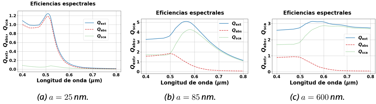
Figura 3: Eficiencias espectrales de la esfera individual de Au para los tres radios estudiados. Para a = 25 \text{ nm} la respuesta óptica está dominada por el modo dipolar con Q_{abs} dominante ( x \ll 1 ). Para a = 85 \text{ nm} el espectro presenta un pico pronunciado en torno a \lambda \approx 570 \text{ nm} donde la contribución cuadrupolar es relevante ( x \sim 1 ). Para a = 600 \text{ nm} las eficiencias varían suavemente con contribuciones multipolares de orden superior, siendo la dispersión dominante en todo el rango visible ( x \gg 1 ).
