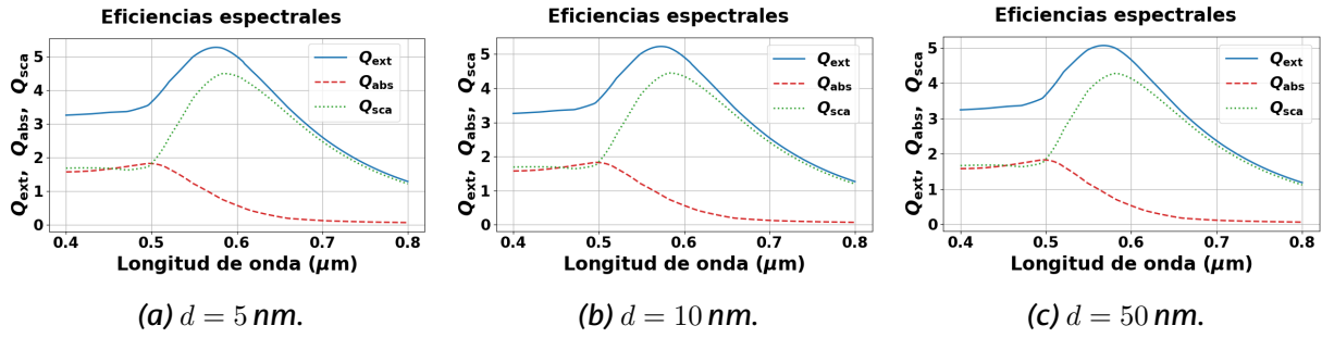
Figura 11: Eficiencias espectrales del dímero heterogéneo ( a_1 = 25 \text{ nm} , a_2 = 85 \text{ nm} ) para tres separaciones. El espectro reproduce la forma de la esfera individual de 85 \text{ nm} : pico de dispersión dominante en torno a \lambda \approx 560\text{--}580 \text{ nm} con absorción pequeña. La esfera mayor gobierna la respuesta óptica del conjunto y el gap no produce desplazamiento espectral apreciable.
