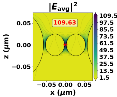
(b) Campo cercano, \lambda = 520 \text{ nm} . Máximo: 109.63 |E_0|^2 .
