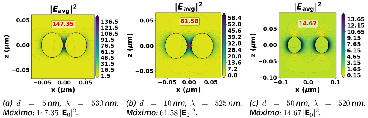
Figura 6: Campo cercano |E_{avg}|^2 del dímero con a = 25 nm evaluado a la longitud de onda de máxima Q_{sca} . La zona de concentración se localiza en el gap entre las dos esferas. Al reducir el gap de 50 nm a 5 nm, la intensificación máxima pasa de 14.67 |E_0|^2 a 147.35 |E_0|^2 , un aumento de un orden de magnitud respecto a la esfera individual ( 11.90 |E_0|^2 ).
