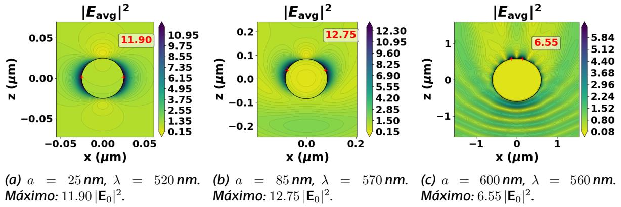
Figura 4: Campo cercano |E|^2 de la esfera individual de Au para los tres radios. Para a = 25 \text{ nm} la intensificación se localiza en los polos de la esfera perpendiculares a la dirección de propagación, característico del modo dipolar ( x \ll 1 ). Para a = 85 \text{ nm} la concentración superficial aparece ligeramente desplazada hacia adelante (la cara de sombra), reflejo de la contribución de órdenes superiores ( x \sim 1 ). Para a = 600 \text{ nm} el campo exhibe patrones de interferencia característicos del régimen de Mie avanzado.
