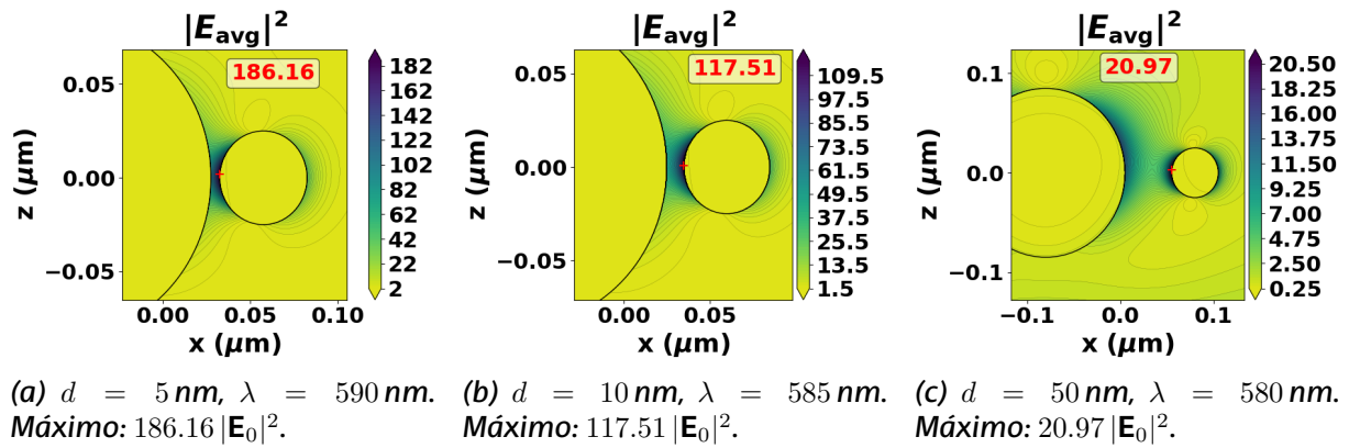
Figura 12: Campo cercano |E_{avg}|^2 del dímero heterogéneo evaluado a la longitud de onda de resonancia. La zona de concentración se localiza en el gap, entre la cara de la esfera grande y la esfera pequeña. Al reducir d de 50 a 5 \text{ nm} , la intensificación crece de 20.97 a 186.16 |E_0|^2 .
