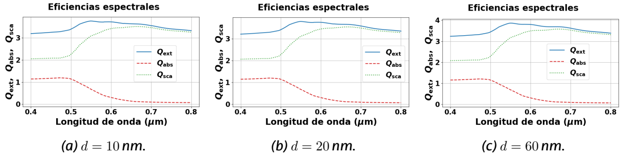
Figura 9: Eficiencias espectrales del dímero con a = 600 \text{ nm} para las tres separaciones estudiadas. Los espectros son prácticamente idénticos entre sí y al de la esfera individual: el gap no produce desplazamiento espectral ni modifica la forma del espectro.
