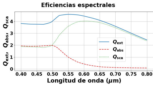
(c) d = 50 \text{ nm} . Resonancia en \lambda \approx 600 \text{ nm} .
