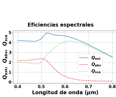
(a) Eficiencias espectrales.
