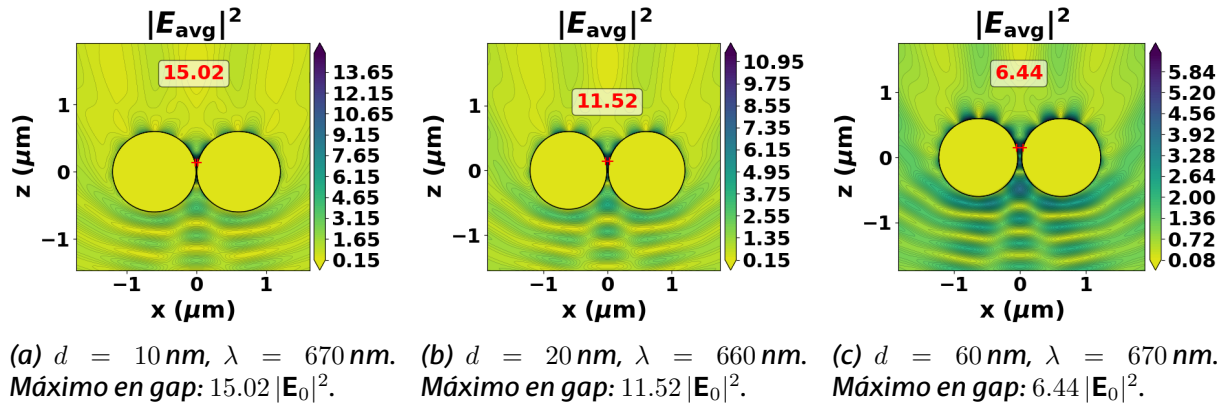
Figura 10: Campo cercano |E_{avg}|^2 del dímero con a = 600 \text{ nm} . El rasgo dominante no es la zona de concentración del gap sino los patrones de interferencia que rodean a las esferas.
