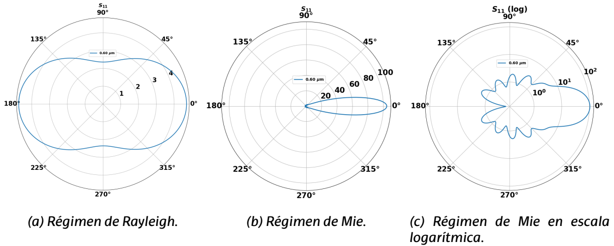
Figura 1: Patrón angular S_{11}(\theta) de una esfera de oro en dos regímenes de dispersión.
