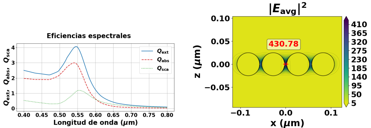
(a) Eficiencias espectrales. Pico en \lambda \approx 550 nm con Q_{\text{abs}} dominante.
