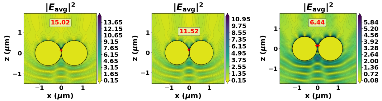
Máximo en gap: 15.02 |E_0|^2 . Máximo en gap: 11.52 |E_0|^2 . Máximo en gap: 6.44 |E_0|^2 .
