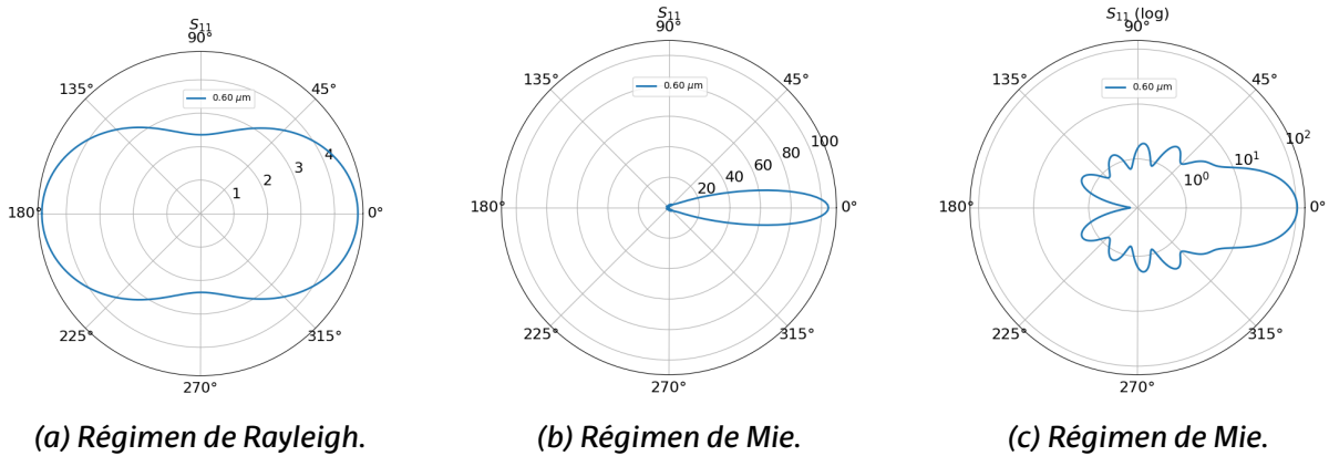
Figura 1: Patrón angular S_{11}(\theta) de una esfera de oro en dos regímenes de dispersión.
