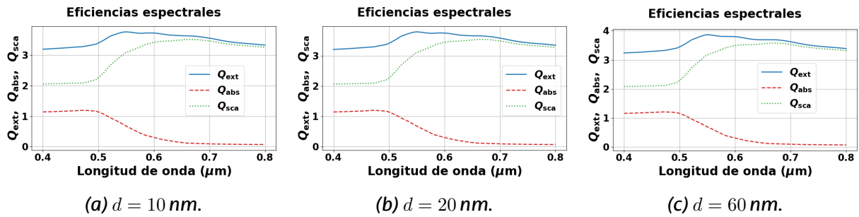
Figura 9: Eficiencias espectrales del dímero con a = 600 nm para las tres separaciones estudiadas.
