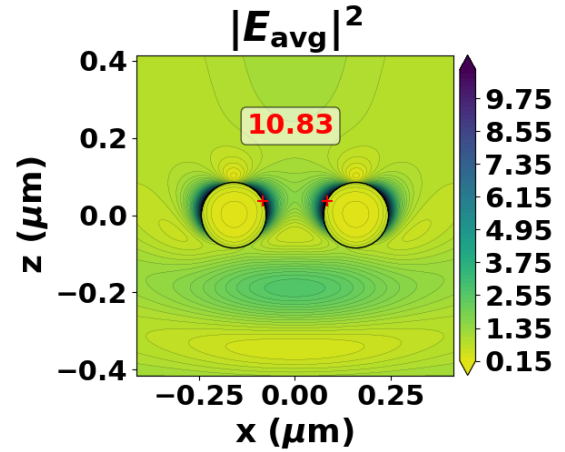
(d) d = 150 \text{ nm} , \lambda = 560 \text{ nm} .
