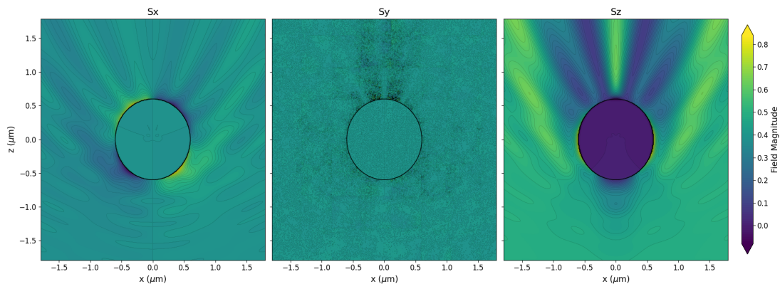
Figura 4: Vector poynting en el campo cercano por una esfera de oro.
