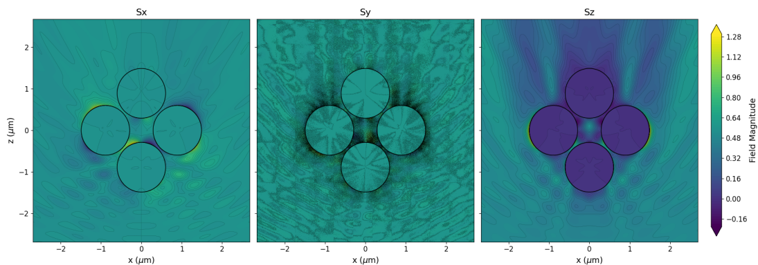
Figura 6: Vector poynting en el campo cercano.
