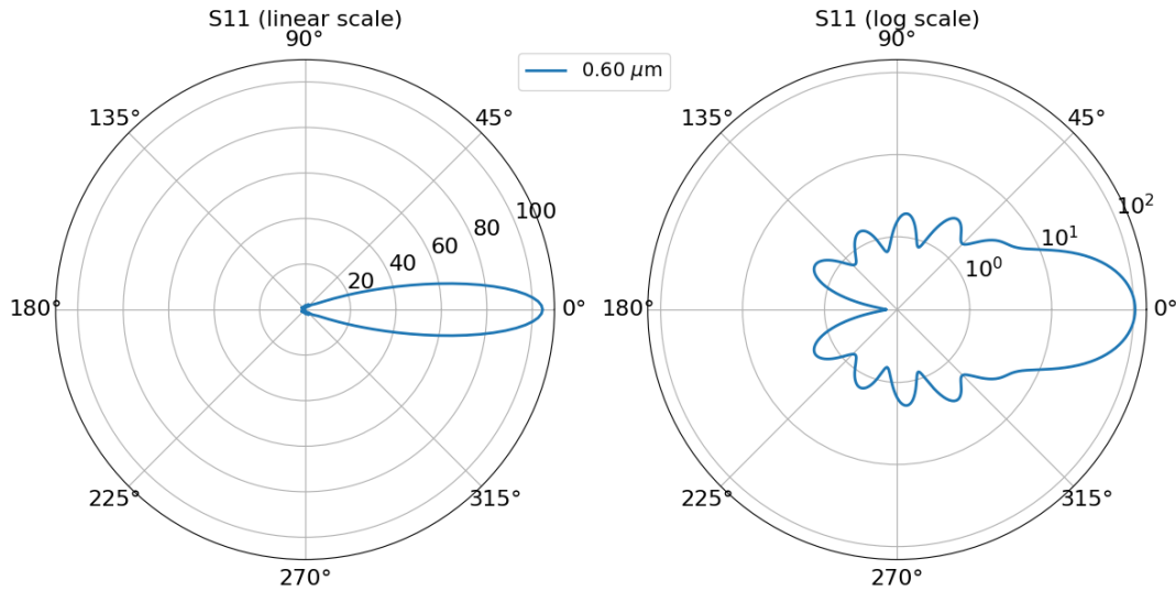
Figura 3: Radiación dispersada en función del ángulo de observación en el campo lejano por una esfera de oro de \lambda = r = 0.6 \mu\text{m} .
