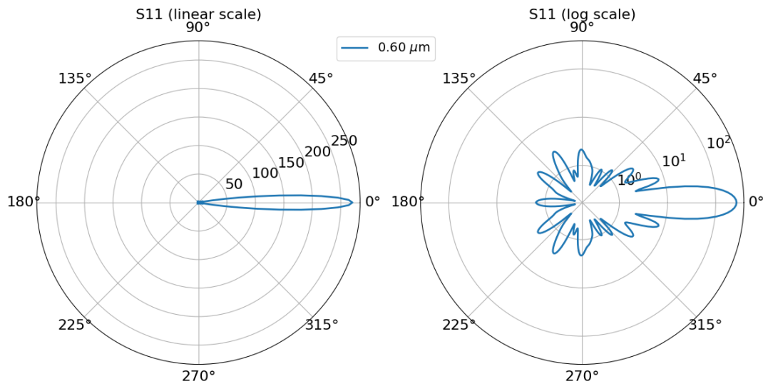
Figura 3: Radiación dispersada en función del ángulo de observación en el campo lejano por 4 esferas formando un cuadrado y un ángulo de 45°.
