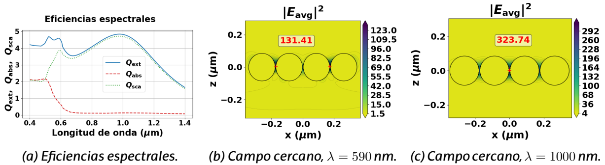
Figura 14: Tetrámero homogéneo con a = 85 nm y d = 5 nm.
