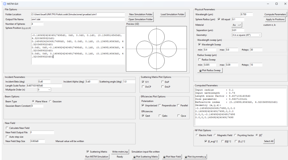
Figura 2: Interfaz gráfica del entorno en Python para MSTM, configurada para una simulación de ejemplo: cuatro esferas de oro de radio 0.1 \mu\text{m} dispuestas en un cuadrado a 45^\circ respecto a la onda incidente, con un barrido en longitud de onda de 400 a 800 nm en 30 pasos. Se aprecia también la vista previa del agregado, que se actualiza en tiempo real.
