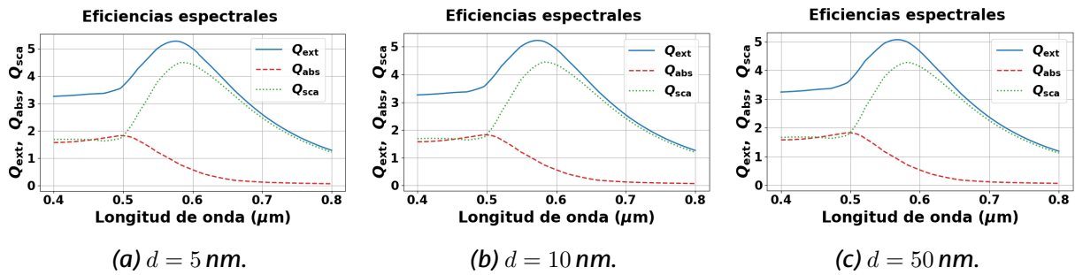
Figura 11: Eficiencias espectrales del dímero heterogéneo ( a_1 = 25 nm, a_2 = 85 nm) para las tres separaciones estudiadas.
