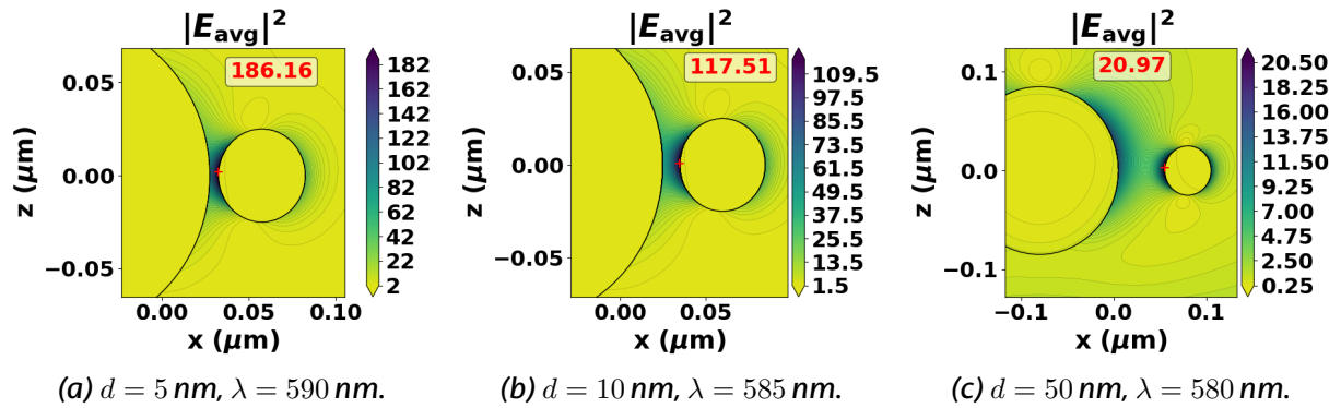
Figura 12: Campo cercano |E_{\text{avg}}|^2 del dímero heterogéneo evaluado a la longitud de onda de resonancia.
