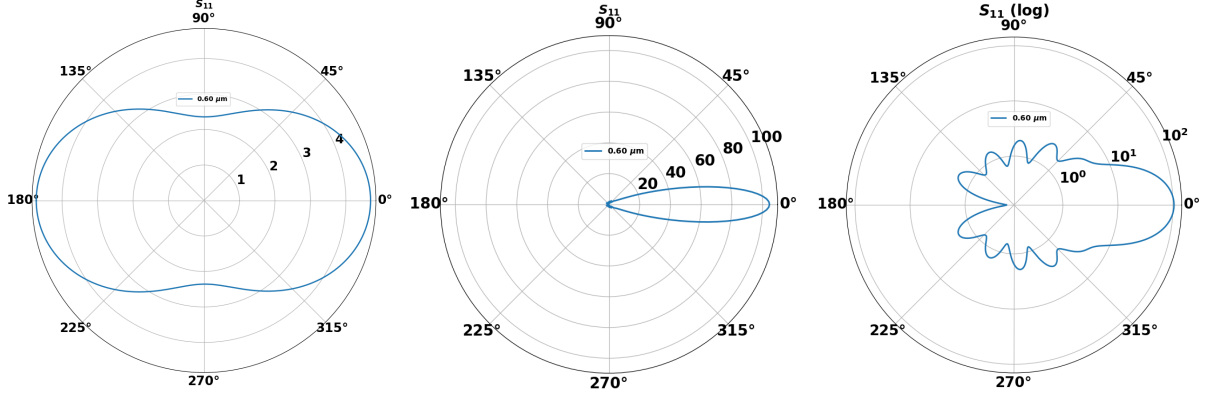
(a) Régimen de Rayleigh x \sim 0.1 . (b) Régimen de Mie x \sim 6 . (c) Régimen de Mie en escala logarítmica x \sim 6 .
