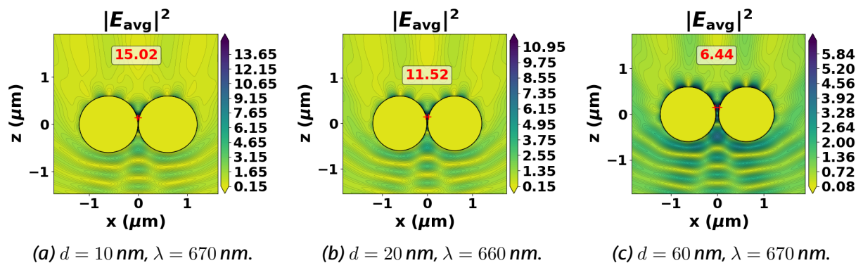
Figura 10: Campo cercano |E_{avg}|^2 del dímero con a = 600 nm evaluado a la longitud de onda de máxima Q_{sca} .
