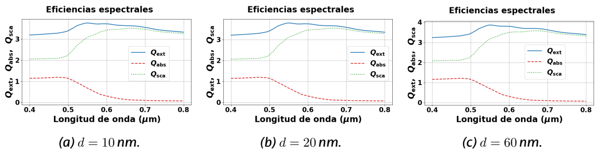
Figura 9: Eficiencias espectrales del dímero con a = 600 nm para las tres separaciones estudiadas.
