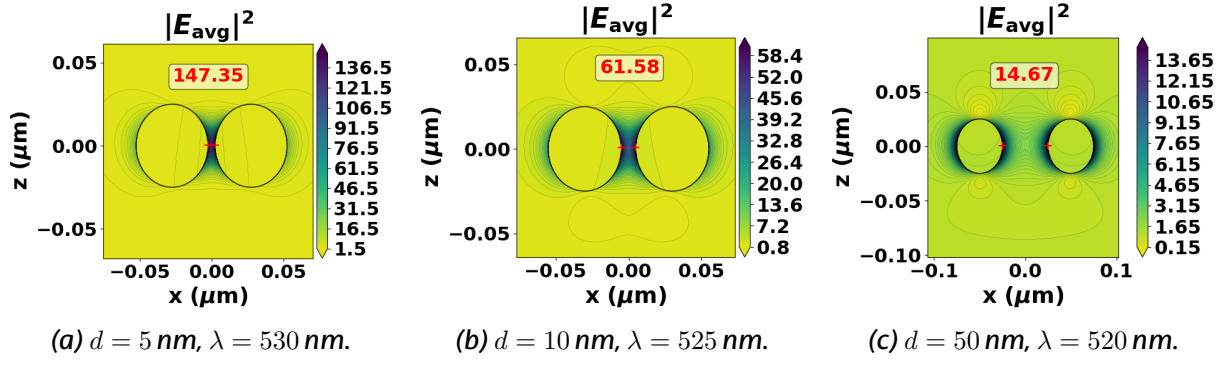
Figura 6: Campo cercano |E_{avg}|^2 del dímero con a = 25 \text{ nm} evaluado a la longitud de onda de máxima Q_{sca} .
