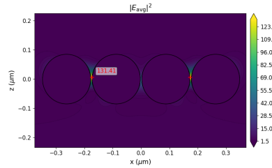
(b) Campo cercano, \lambda = 590 nm. Máximo: 131.41 |E_0|^2 .
