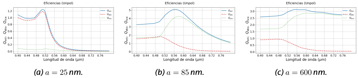
Figura 3: Eficiencias espectrales de la esfera individual de Au para los tres radios estudiados. Para a = 25 nm la respuesta óptica está dominada por el modo dipolar con Q_{abs} dominante ( x \ll 1 ). Para a = 85 nm el espectro presenta un pico pronunciado en torno a \lambda \approx 570 nm donde la contribución cuadrupolar es relevante ( x \sim 1 ). Para a = 600 nm las eficiencias varían suavemente con contribuciones multipolares de orden superior, siendo la dispersión dominante en todo el rango visible ( x \gg 1 ).
