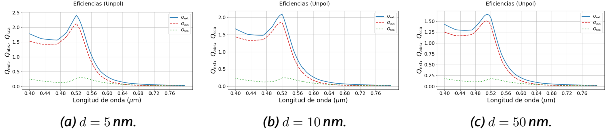
Figura 5: Eficiencias espectrales del dímero con a = 25 nm para tres separaciones. La resonancia permanece en torno a \lambda \approx 520 nm en los tres casos; el acoplamiento incrementa la amplitud del pico sin desplazarlo espectralmente. La absorción sigue siendo el canal dominante de extinción para todos los gaps estudiados. A medida que aumenta d , la amplitud del pico disminuye progresivamente, convergiendo hacia los valores de la esfera individual.
