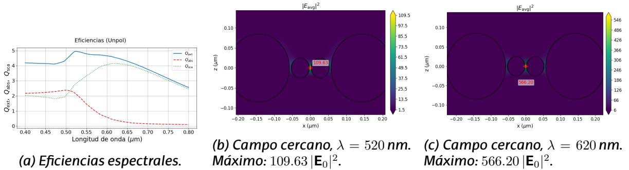
Figura 16: Tetrámero heterogéneo (85–25–25–85 nm) con d = 5 \text{ nm} . El espectro muestra un pico de extinción en \lambda \approx 520 \text{ nm} dominado por la absorción, y un pico dispersor principal en \lambda \approx 620 \text{ nm} . En ambos casos la zona de concentración se localiza entre las dos esferas pequeñas centrales; a \lambda = 620 \text{ nm} la intensificación alcanza 566.20 |\mathbf{E}_0|^2 , el valor más alto de todas las configuraciones estudiadas.
