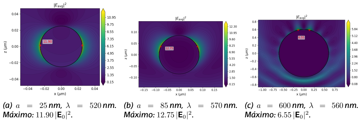
Figura 4: Campo cercano |\mathbf{E}|^2 de la esfera individual de Au para los tres radios. Para a = 25 nm la intensificación se localiza en los polos de la esfera perpendiculares a la dirección de propagación, característico del modo dipolar ( x \ll 1 ). Para a = 85 nm la concentración superficial aparece ligeramente desplazada hacia la cara de iluminación, reflejo de la contribución de órdenes multipolares superiores ( x \sim 1 ). Para a = 600 nm el campo exhibe patrones de interferencia característicos del régimen de Mie avanzado.
