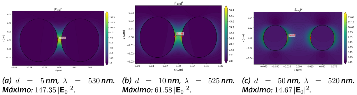
Figura 6: Campo cercano |E_{avg}|^2 del dímero con a = 25 nm evaluado a la longitud de onda de máxima Q_{sca} . La zona de concentración se localiza en el gap entre las dos esferas. Al reducir el gap de 50 nm a 5 nm, la intensificación máxima pasa de 14.67 |E_0|^2 a 147.35 |E_0|^2 , un aumento de un orden de magnitud respecto a la esfera individual ( 11.90 |E_0|^2 ).
