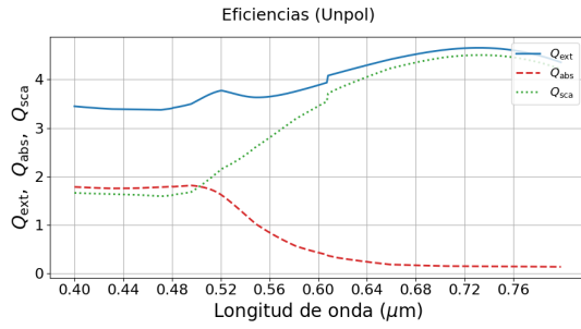
(a) d = 4 \text{ nm} . Resonancia en \lambda \approx 720 \text{ nm} .
