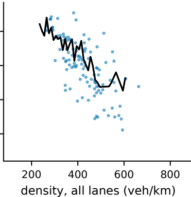
gru
