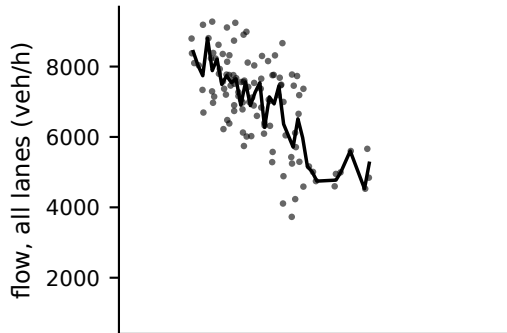
mlp
