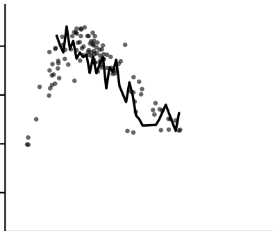
gru
