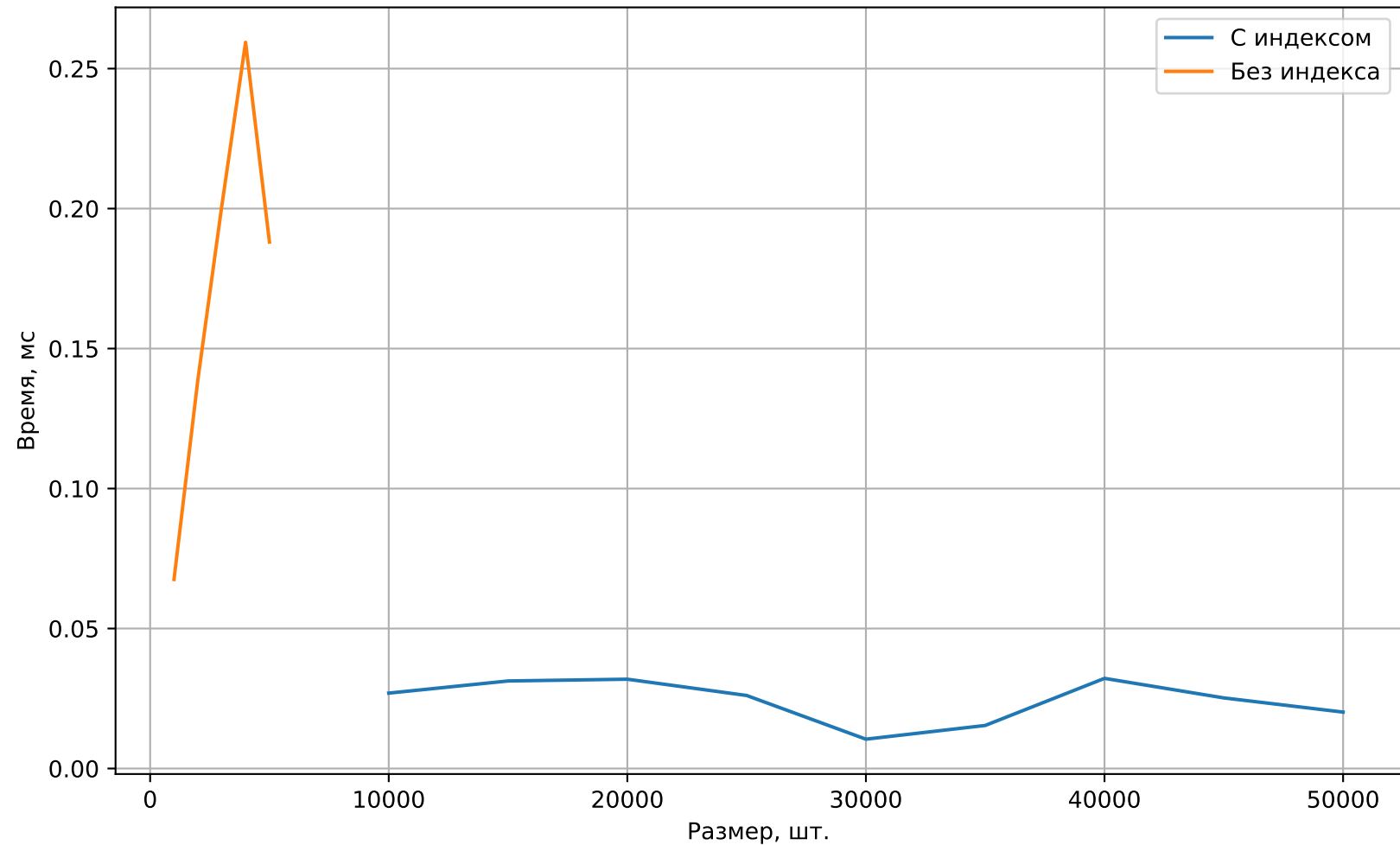
Сравнение времени выполнения
