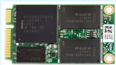
mSATA
