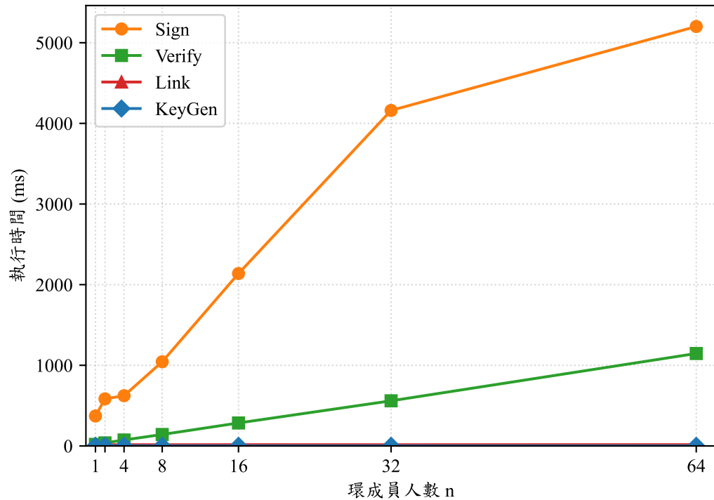
LRS 各演算法執行時間 (lrs-1024)
