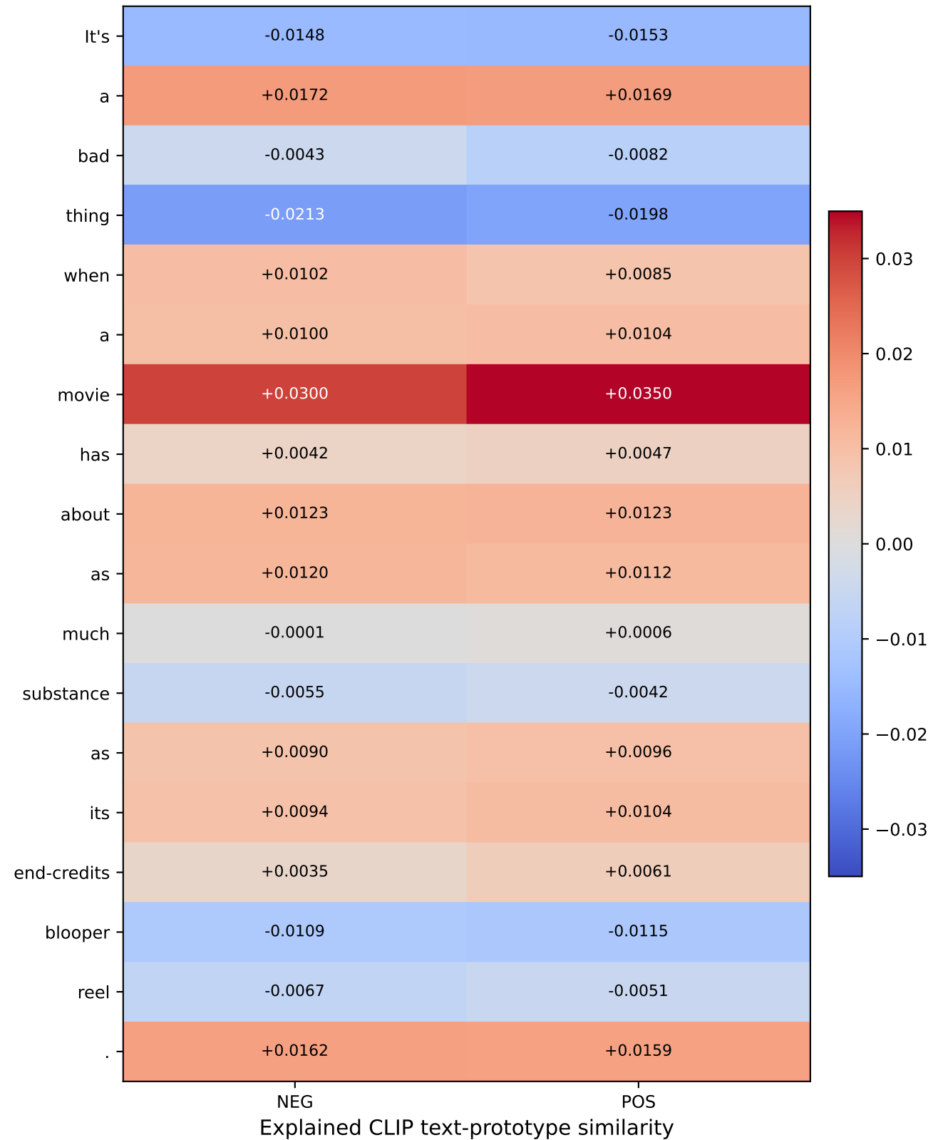
Word-level SHAP values
