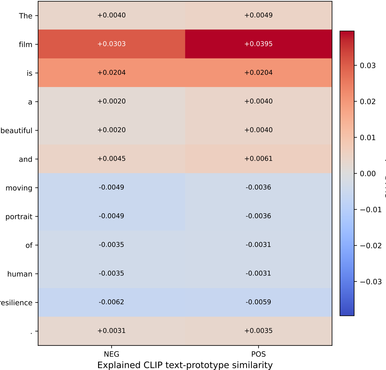
Word-level SHAP values
