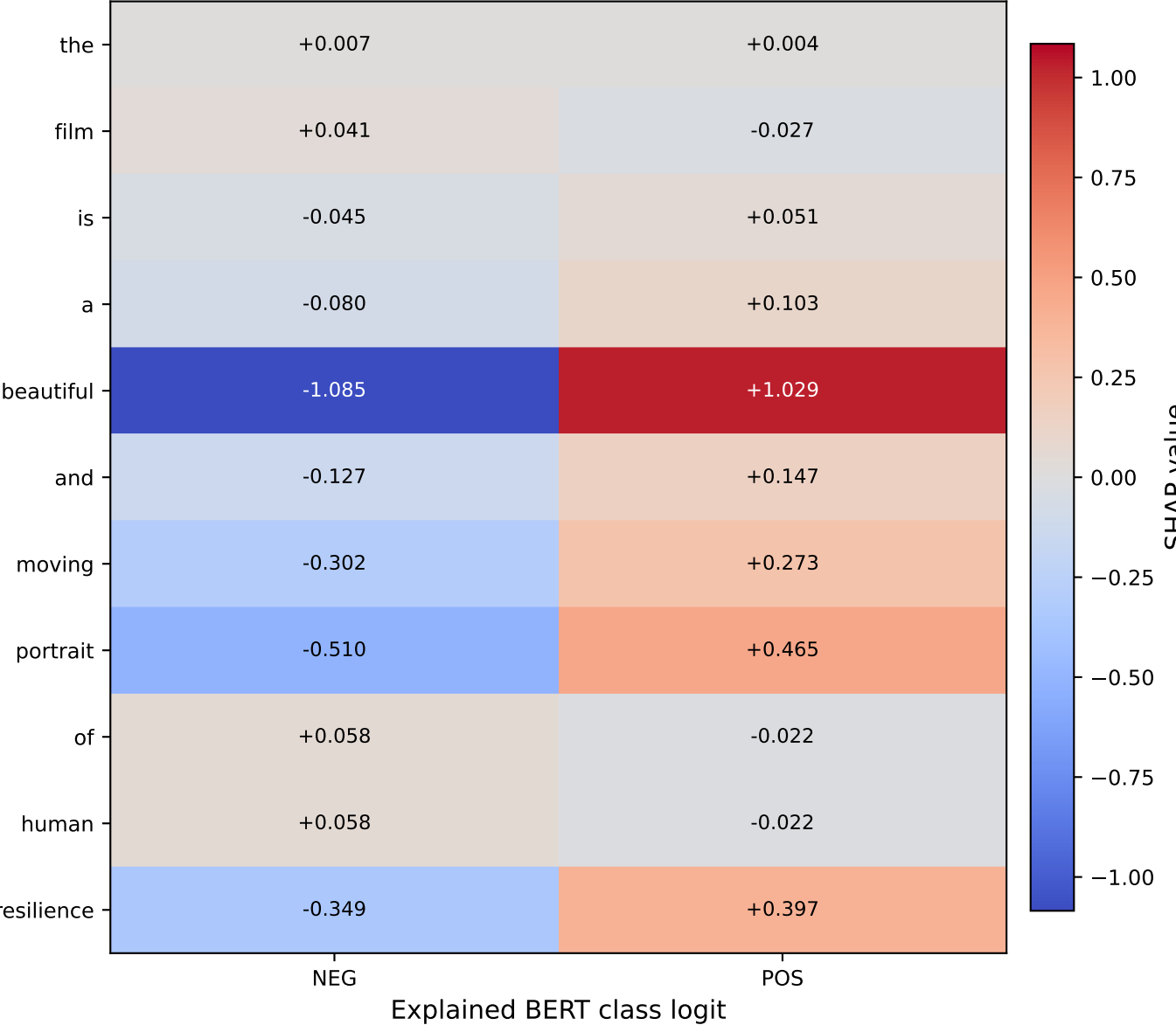
Word-level SHAP values
