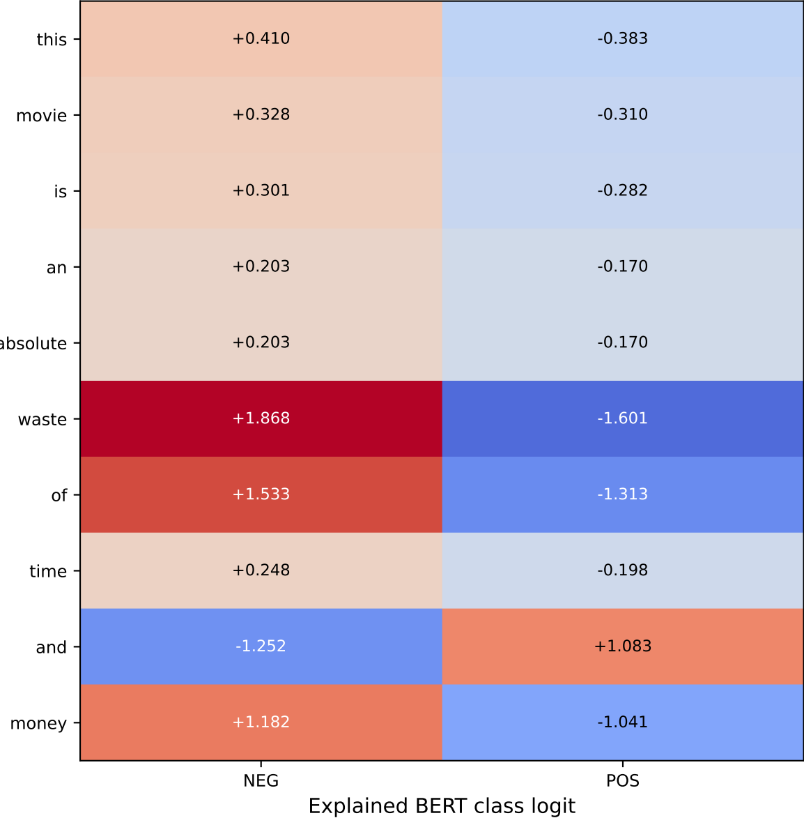
Word-level SHAP values
