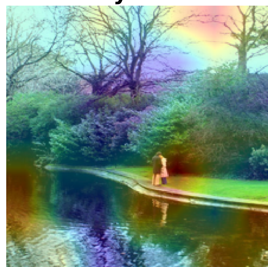
Layer 10
