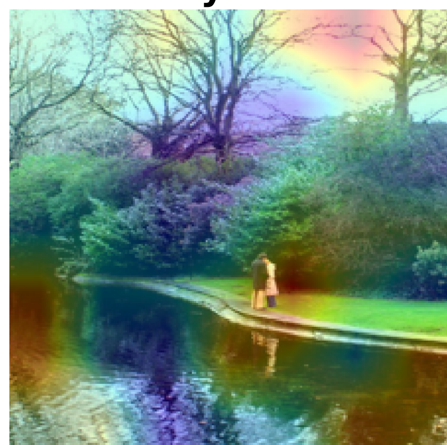
Layer 9
