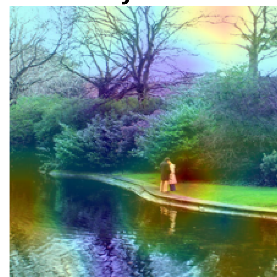
Layer 12
