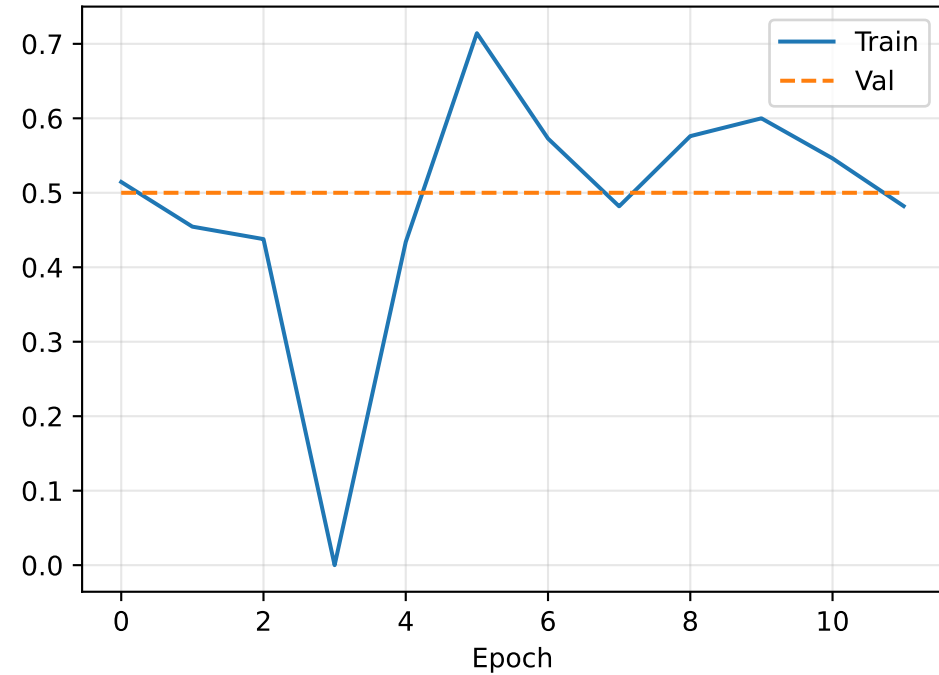
EfficientNetB0 — AUC
