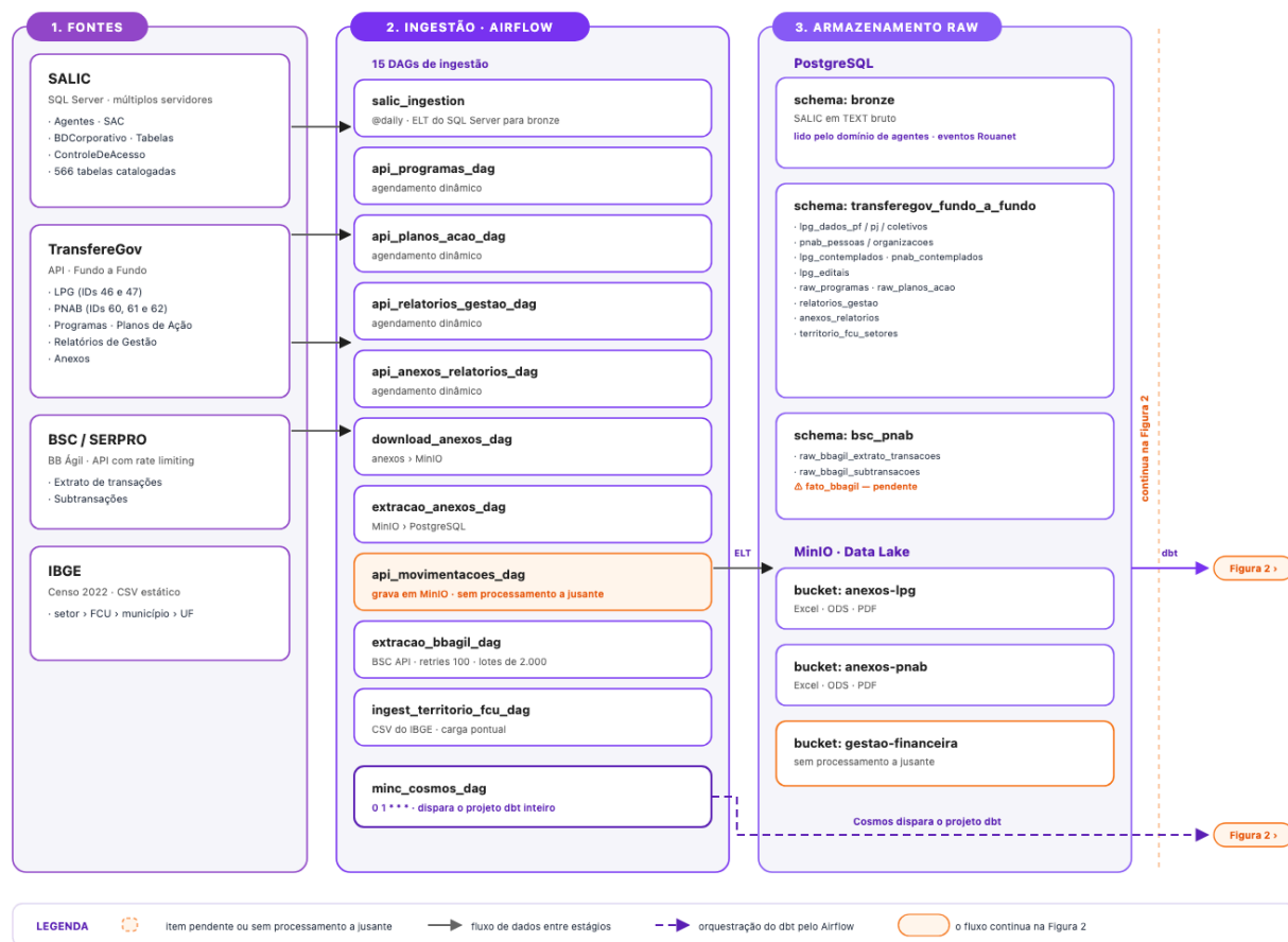
Figura 1. Arquitetura de ingestão e destino das fontes no data lake: do sistema de origem ao dado bruto. Cada rotina do orquestrador responde por um ponto de acesso de origem, com periodicidade própria. Em âmbar, os pontos pendentes. A coluna de ingestão detalha as dez rotinas do núcleo do monitoramento; as cinco incorporadas depois — as duas do plano de ação, a série do Banco Central, os agregados do IBGE e a segunda rotina do SALIC — ainda não estão representadas no desenho. Elaborado a partir da leitura do código do repositório.
